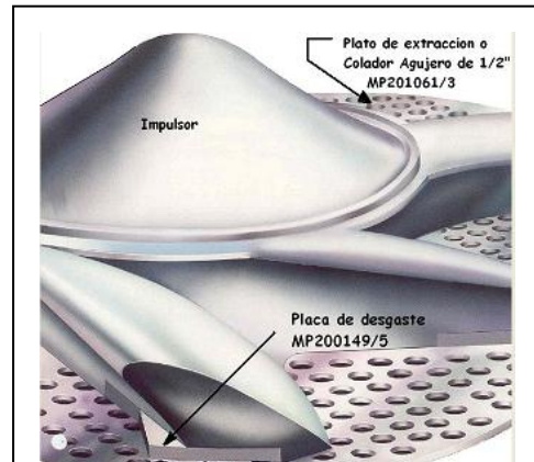
Figura 9. Rotor
