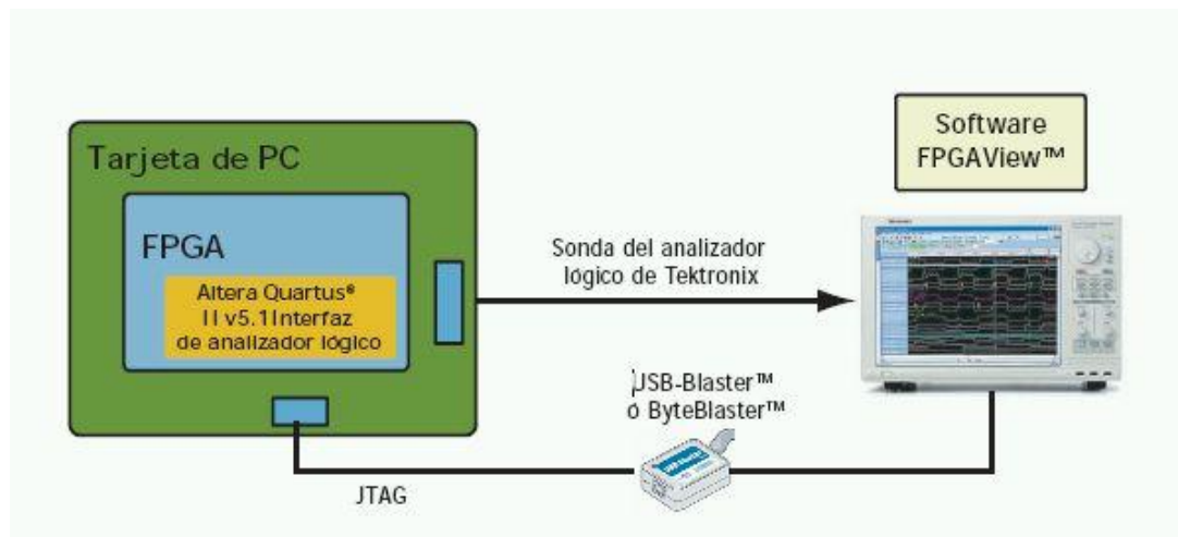
FIGURA 1.3: Esquema de Conexión Tarjeta FPGA.
