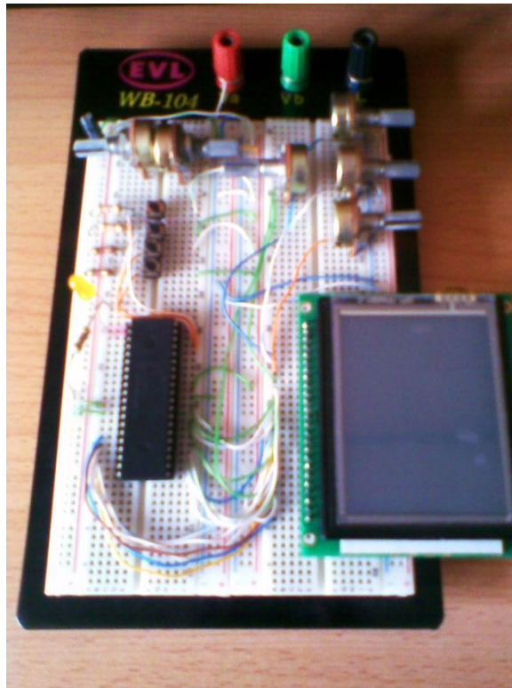
FIGURA 4.1: Conexiones en Protoboard
