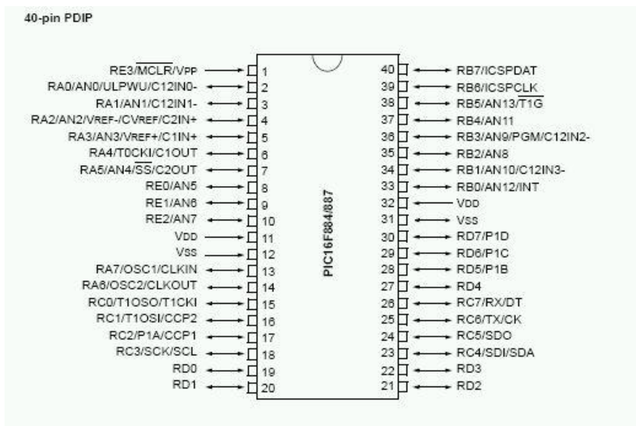
FIGURA 2.3: Configuración de pines PIC 16F887.
