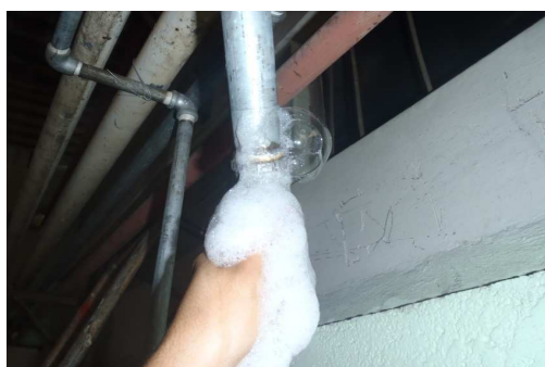
FIG. 3.11 FUGA DE AIRE COMPRIMIDO EN LA LÍNEA
