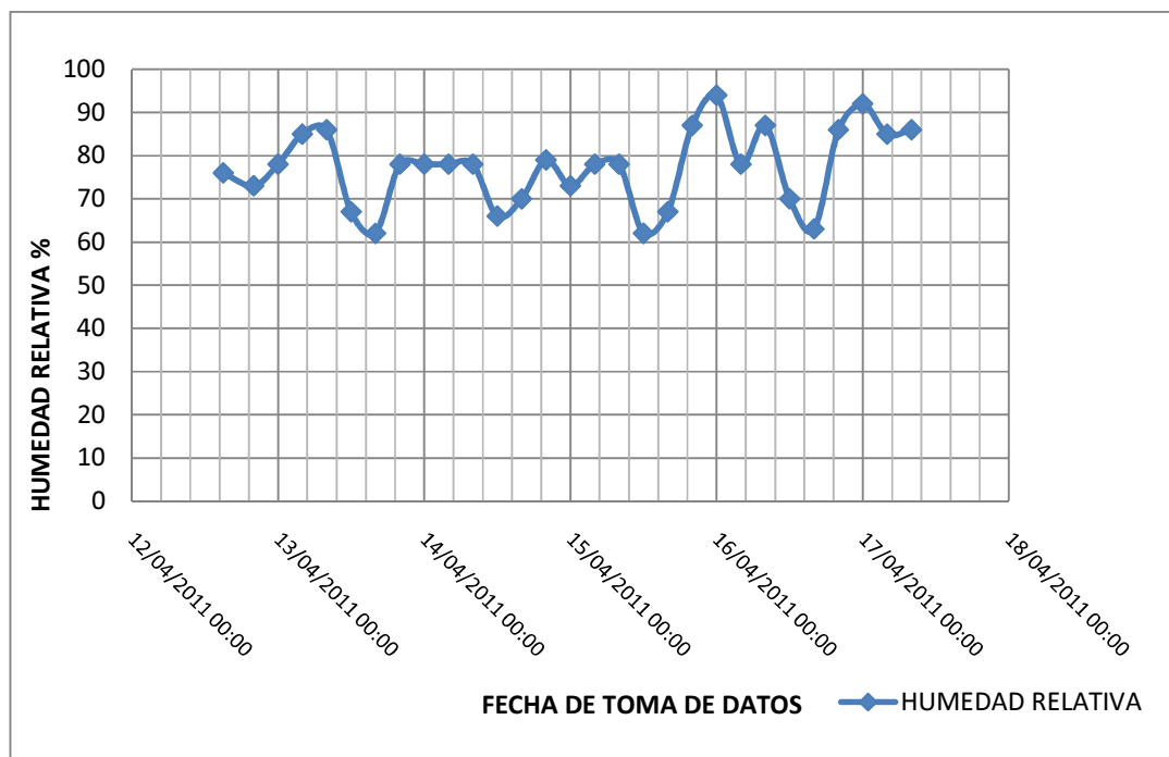
FIG. 2.3 HUMEDAD RELATIVA EN EL CUARTO DEL COMPRESOR 1
