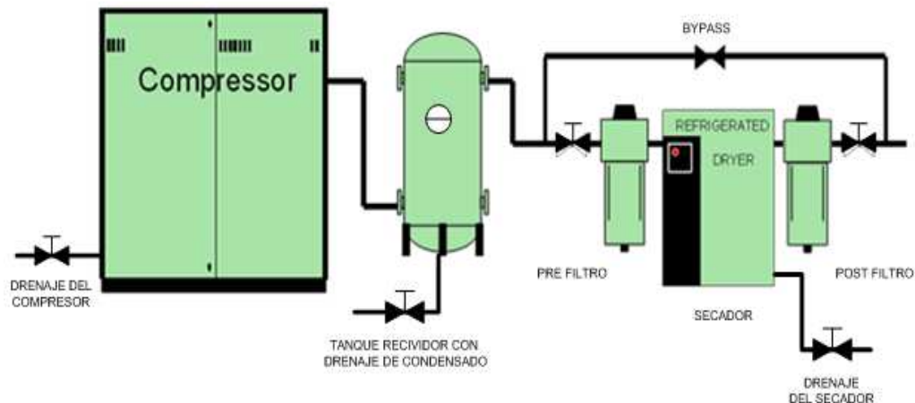
FIG. 2.12 SISTEMA DE TRATAMIENTO DE AIRE COMPRIMIDO
