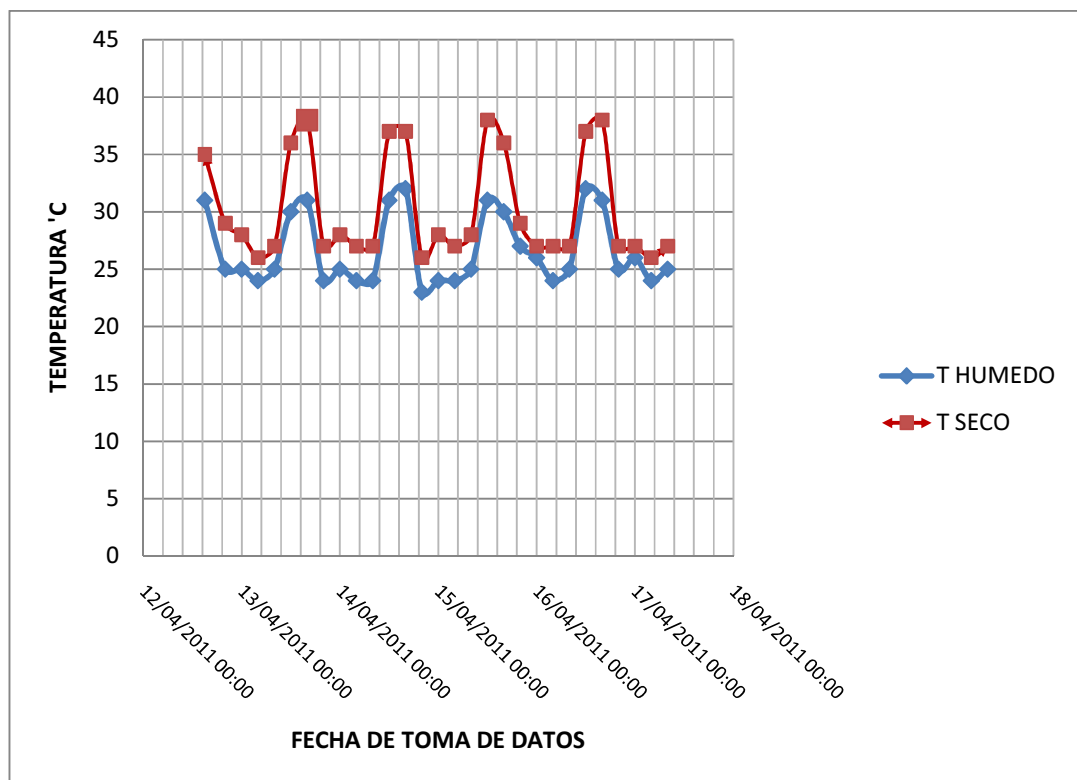
FIG. 2.2 TEMPERATURAS DEL CUARTO DEL COMPRESOR 1
