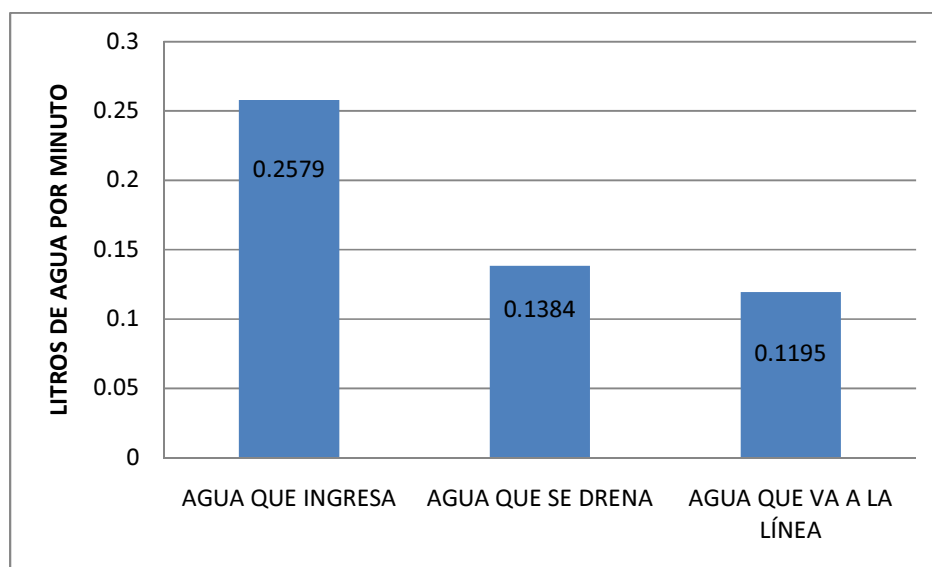
FIG. 2.8 VOLUMEN DE AGUA DEL COMPRESOR 2
