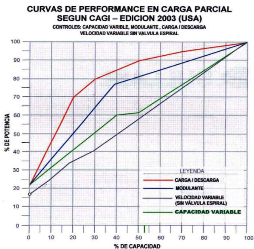
FIG. 3.8 CURVAS DE DESEMPEÑO
