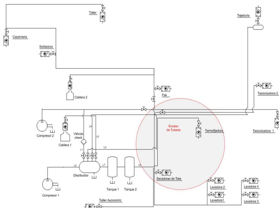
FIG. 4.4 ESQUEMA DEL SISTEMA DE DISTRIBUCIÓN ACTUAL
