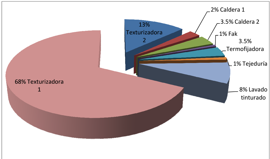
FIG. 2.17 DEMANDA INSTALADA DE AIRE COMPRIMIDO
