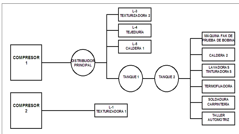
FIG. 2.15 DIAGRAMA DE BLOQUES DEL SISTEMA ACTUAL
