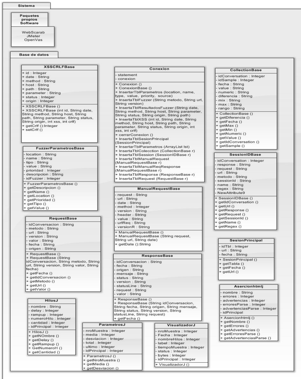
Figura ANEXO B Diagrama de clases
