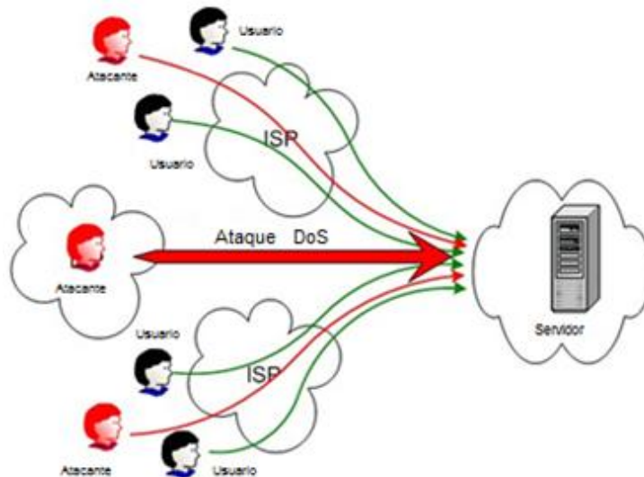
Figura 2.2 Ataque DoS [7]
