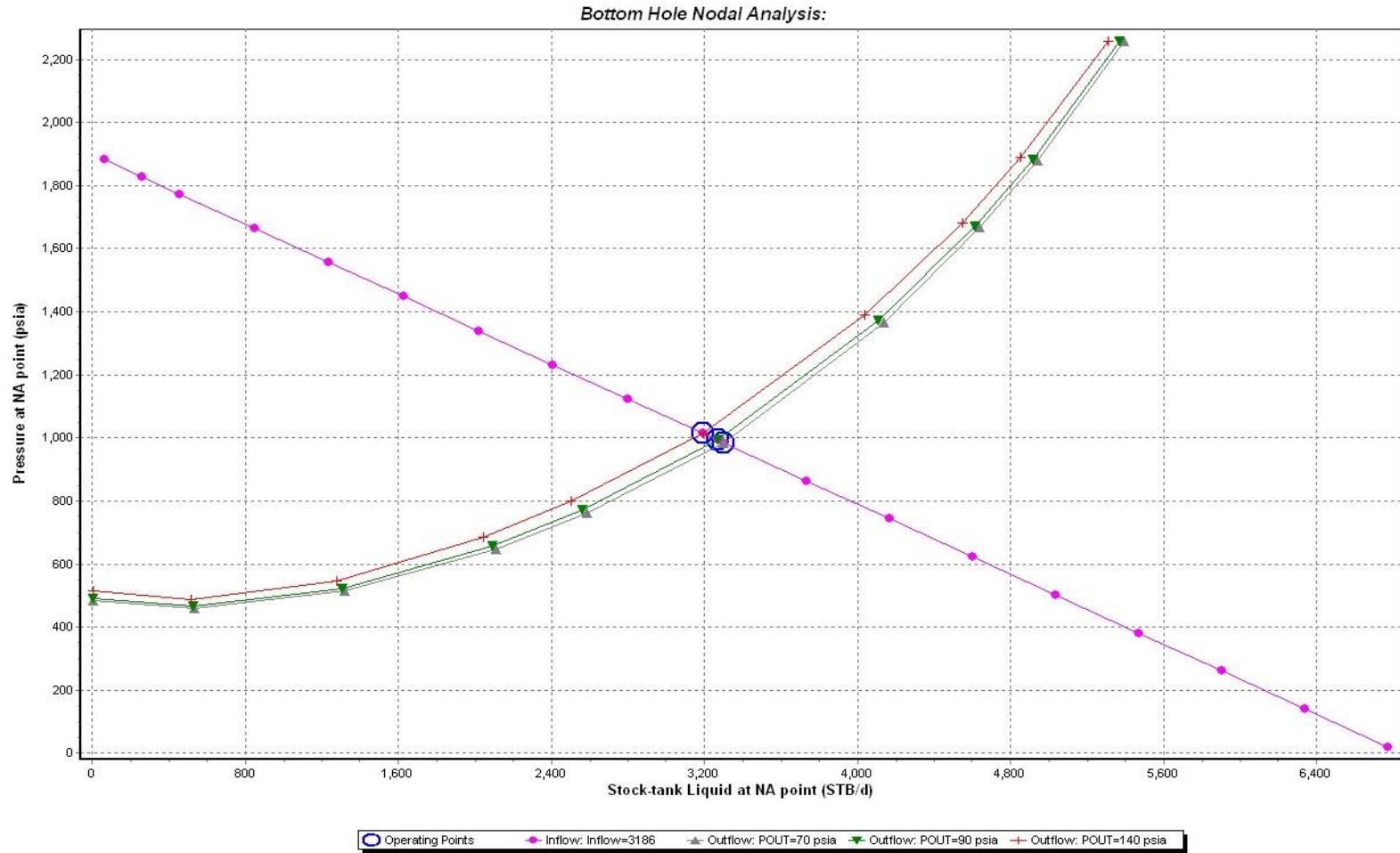
Figura D7: Análisis de sensibilidad del pozo Fanny 18 B 37
