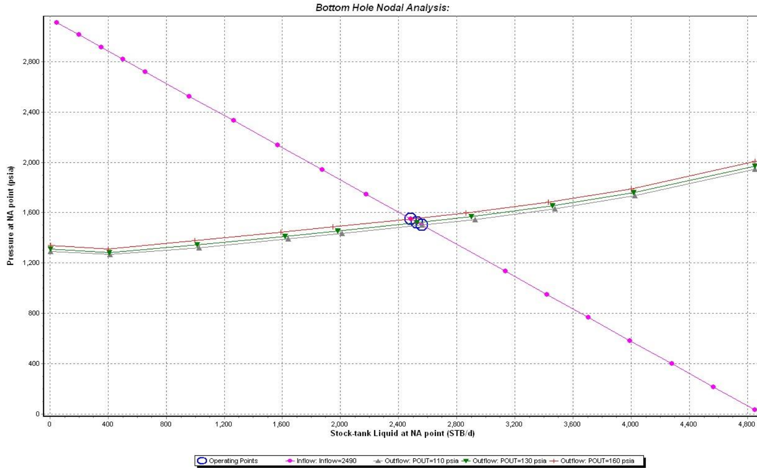
Figura D2: Análisis de sensibilidad del pozo Fanny 18 B 21
