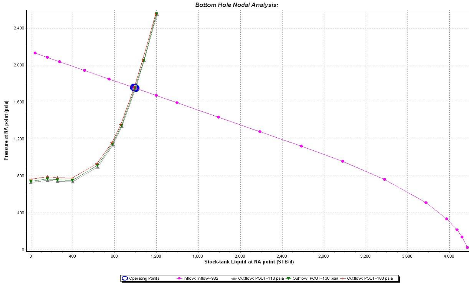
Figura D10: Análisis de sensibilidad del pozo Fanny 18 B 83
