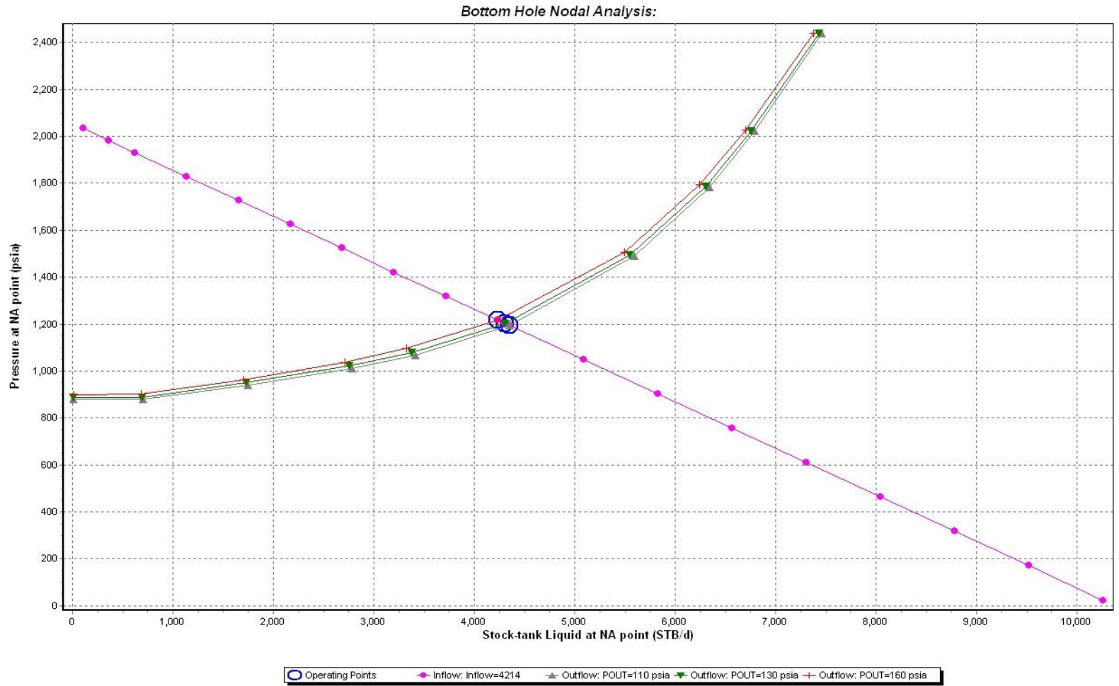
Figura D15: Análisis de sensibilidad del pozo Fanny 18 B 132H
