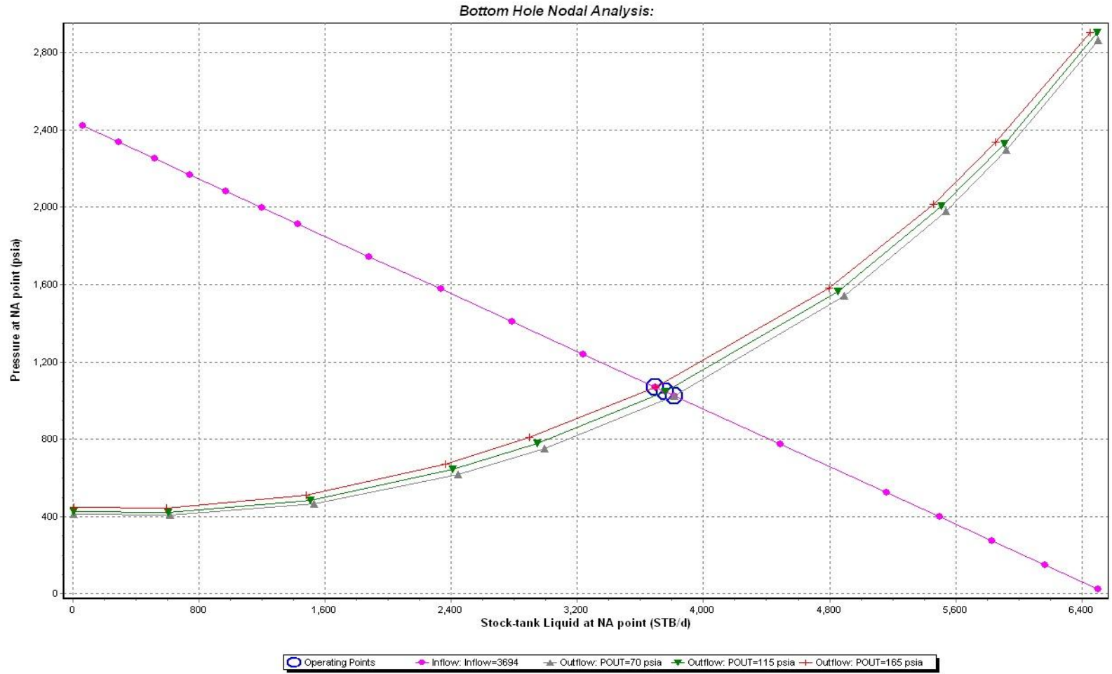
Figura D9: Análisis de sensibilidad del pozo Fanny 18 B 57
