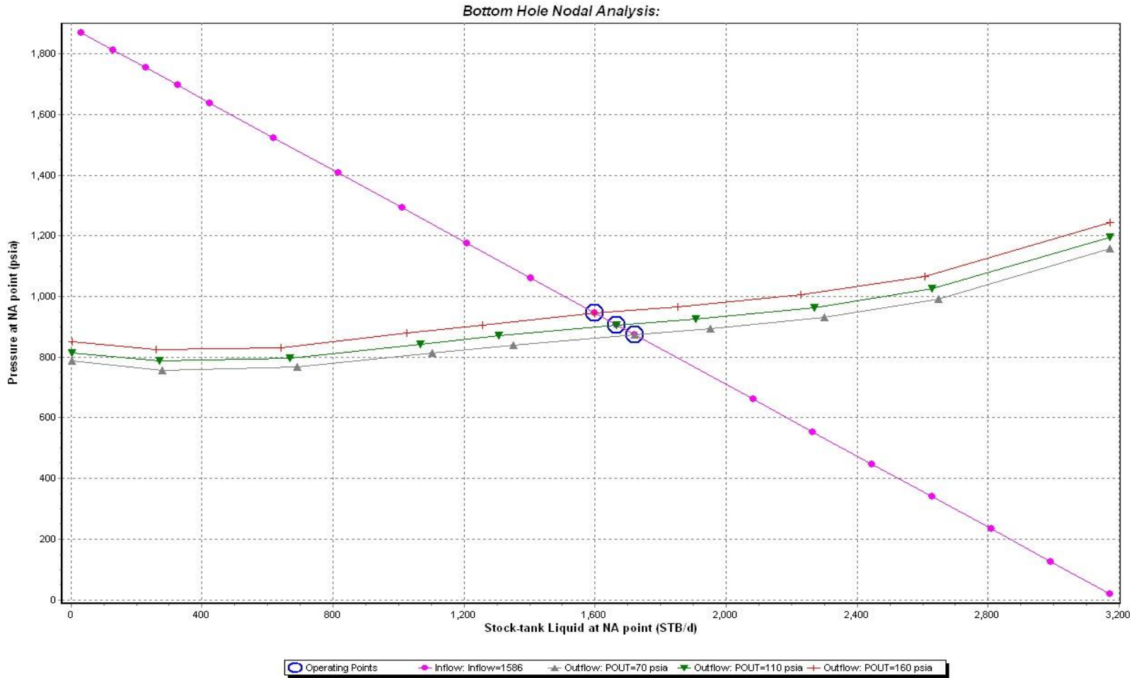
Figura D5: Análisis de sensibilidad del pozo Fanny 18 B 24H
