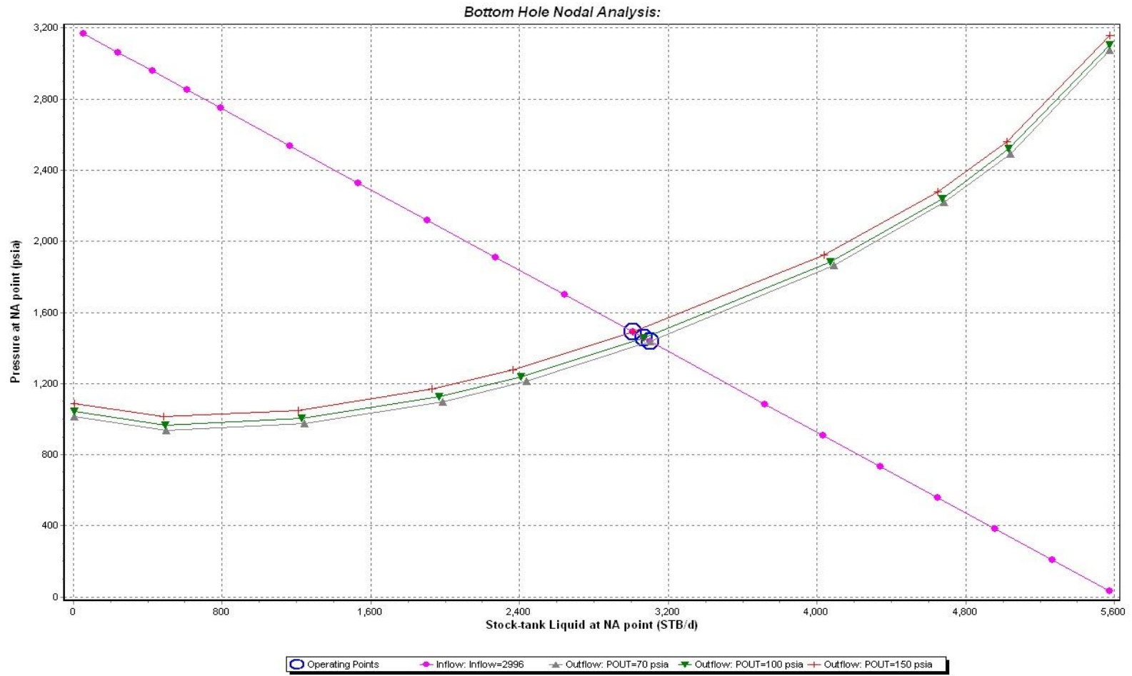
Figura D8: Análisis de sensibilidad del pozo Fanny 18 B 46
