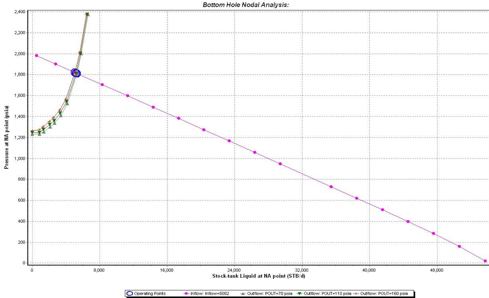
Figura D12: Análisis de sensibilidad del pozo Fanny 18 B 120H
