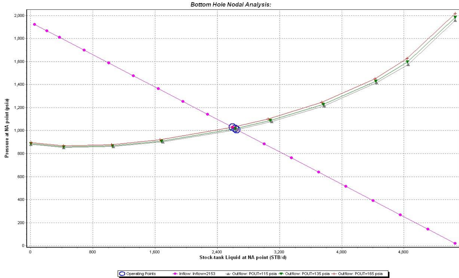
Figura D14: Análisis de sensibilidad del pozo Fanny 18 B 123H
