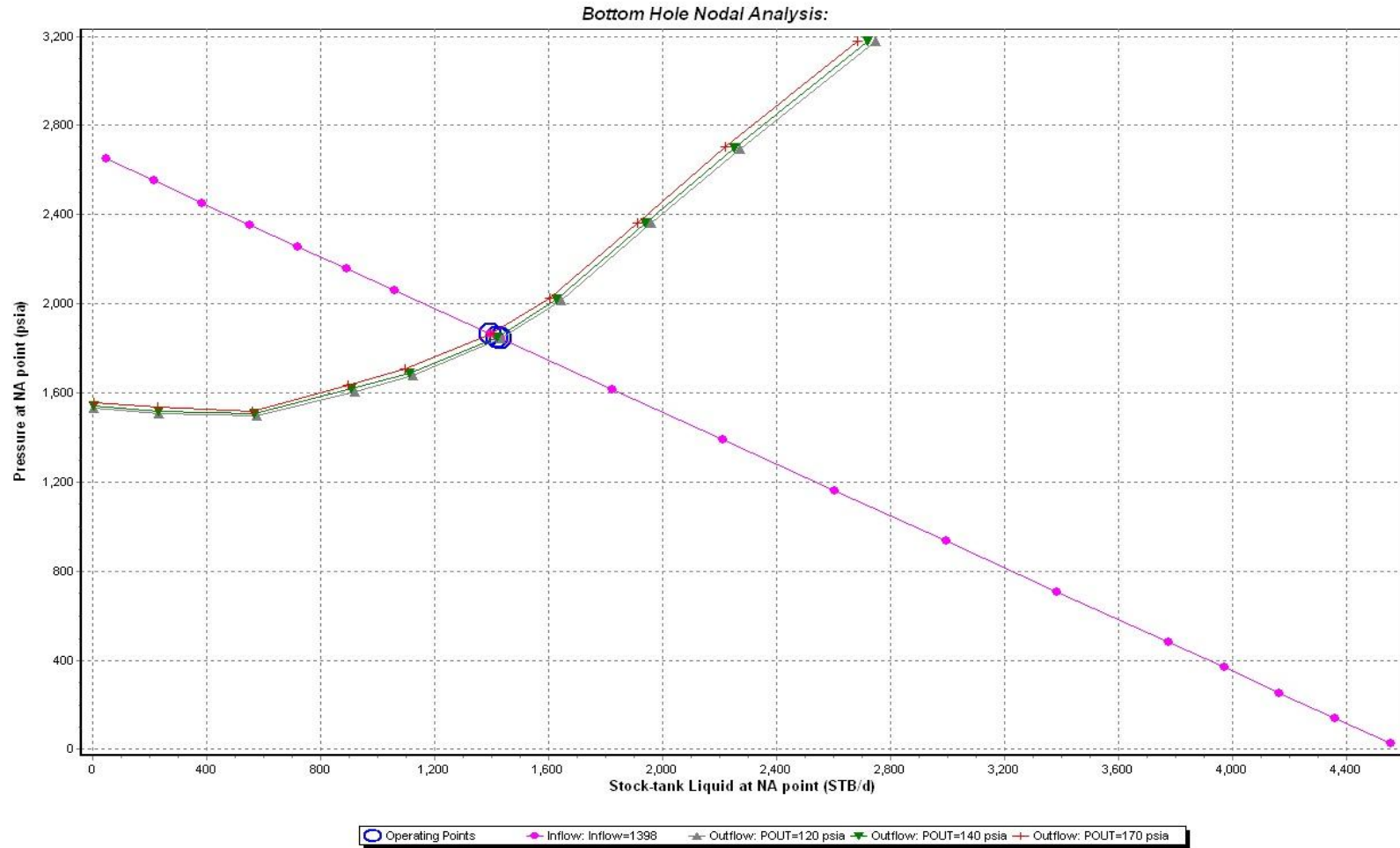
Figura D3: Análisis de sensibilidad del pozo Fanny 18 B 23RE
