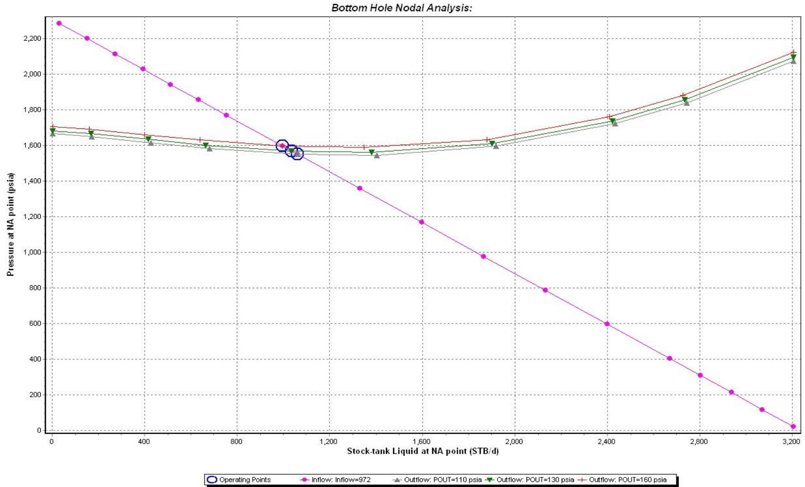
Figura D11: Análisis de sensibilidad del pozo Fanny 18 B 108H
