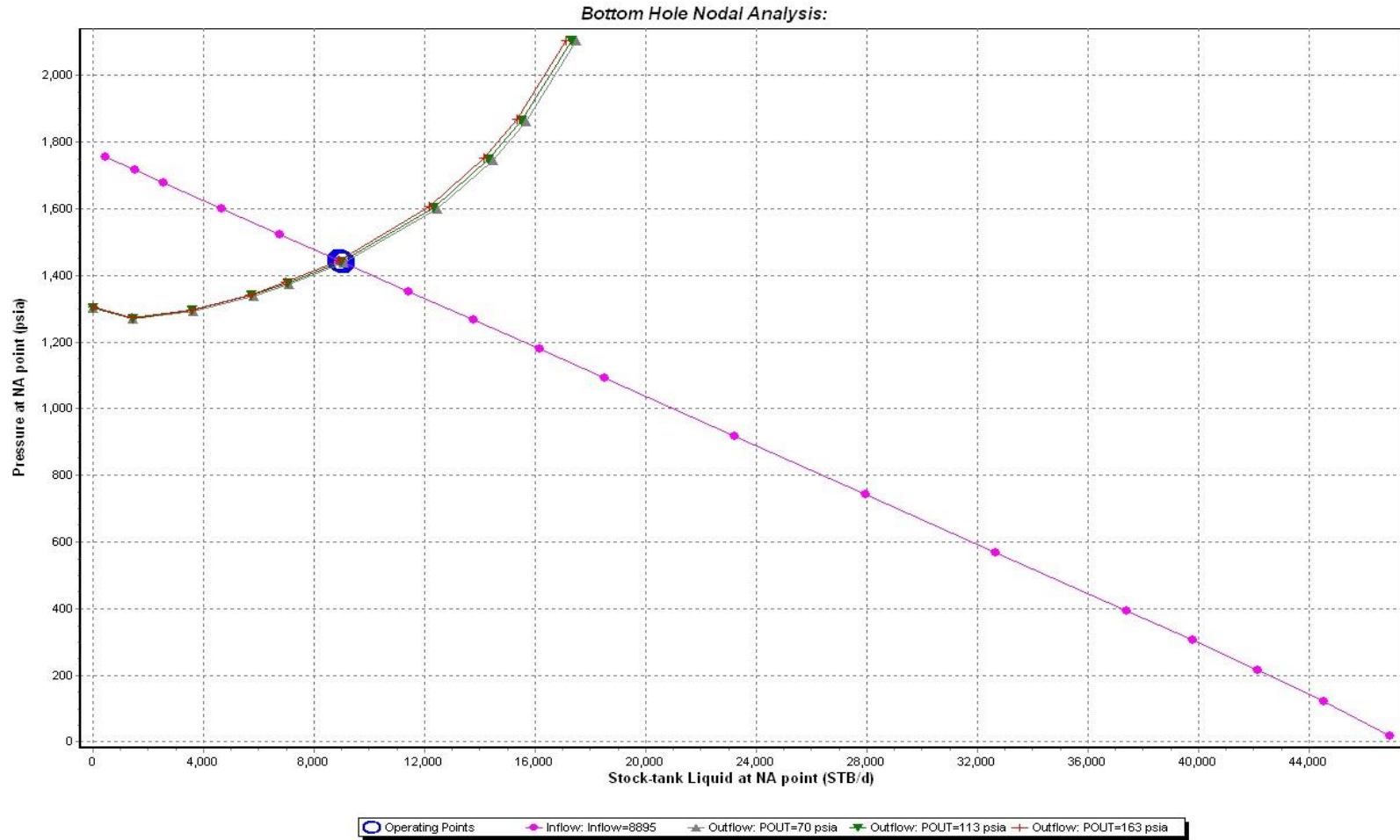
Figura D4: Análisis de sensibilidad del pozo Fanny 18 B 24H
