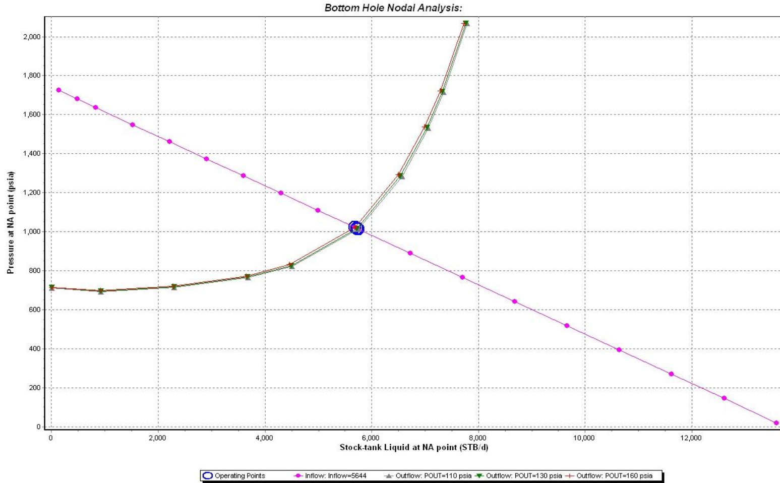
Figura D13: Análisis de sensibilidad del pozo Fanny 18 B 121H
