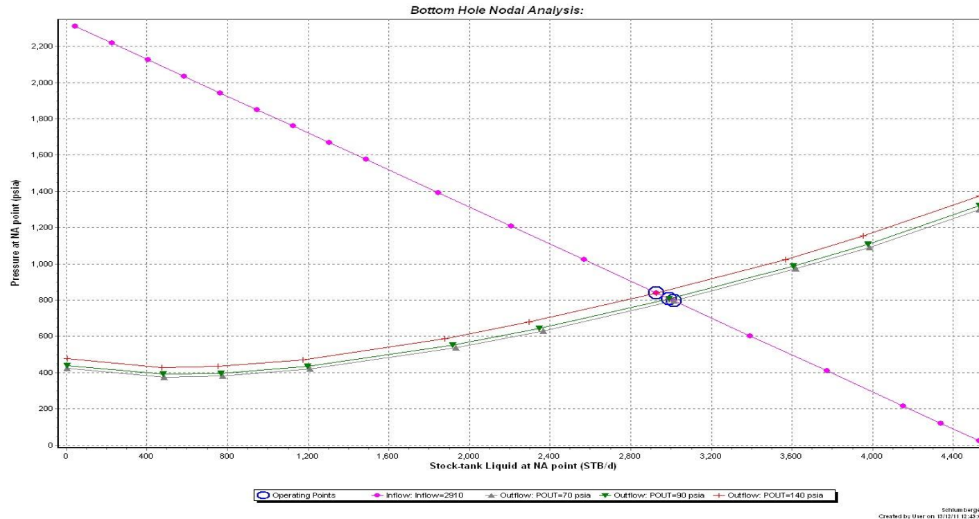
Figura D1: Análisis de sensibilidad del pozo Fanny 18 B 20
