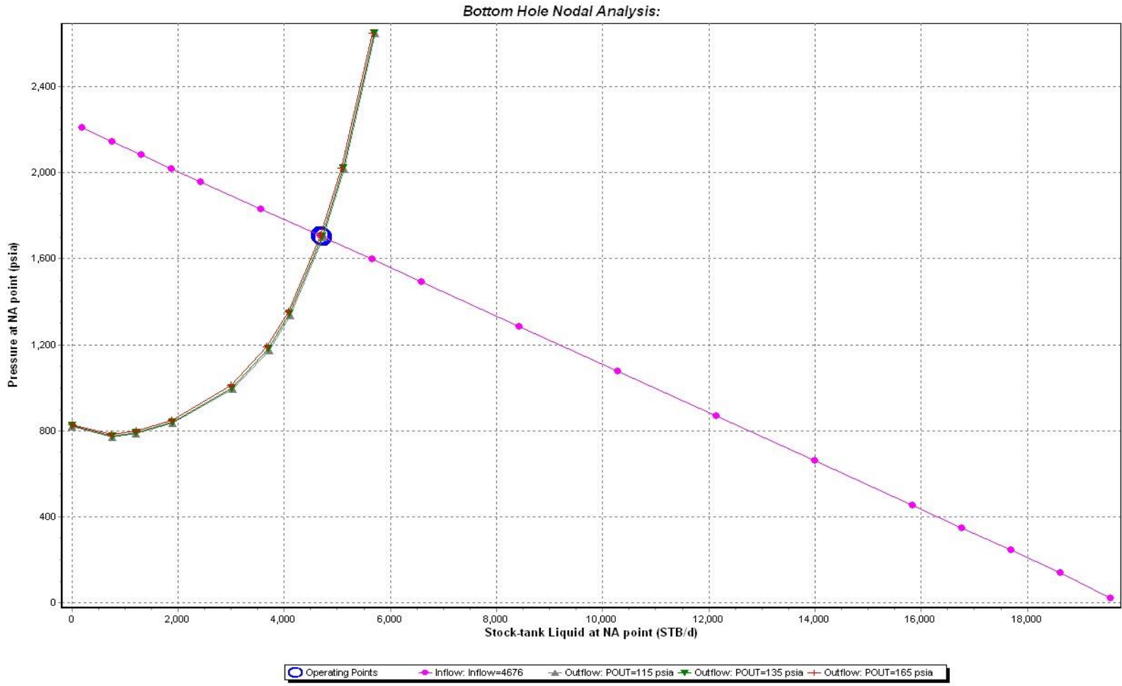
Figura D16: Análisis de sensibilidad del pozo Fanny 18 B 133H
