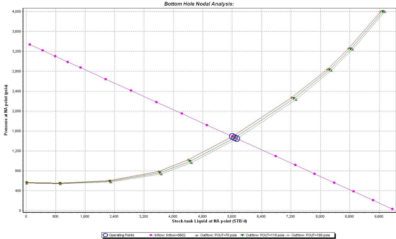
Figura D6: Análisis de sensibilidad del pozo Fanny 18 B 31
