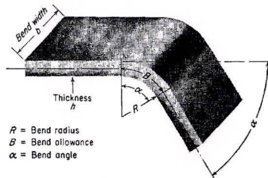
Fig. 1.4 Definición de términos para el proceso de doblado
