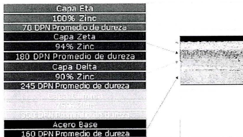
Fig. 1.6 Capas de galvanizado
