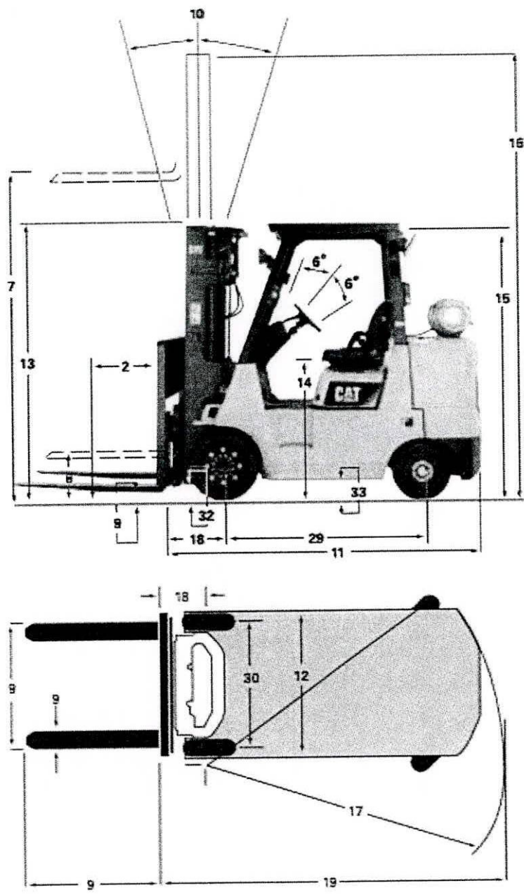
Fig. 3.6 Dimensiones aprox. de montacargas de 7 ton [18].
