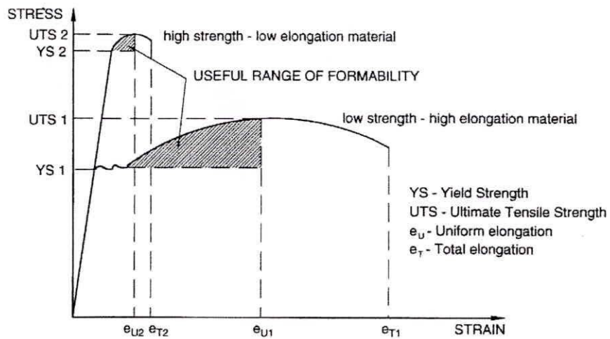
Fig. 1.5 Rango de Formabilidad [6]
