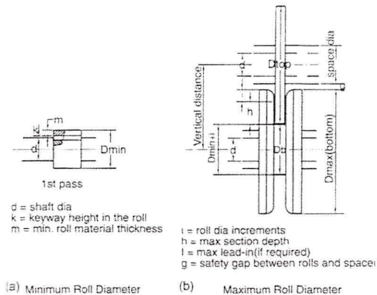
Fig. 2.10 Diámetro máximo y mínimo de rodillo.
