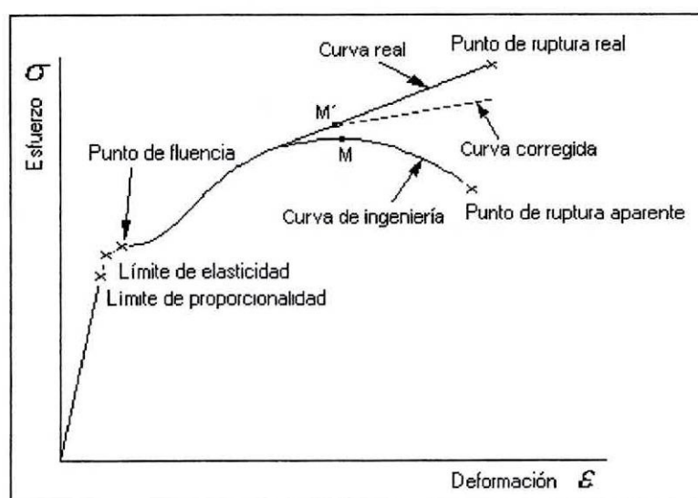
Fig. 1.1 Curva Esfuerzo-Deformación típica para un metal dúctil
