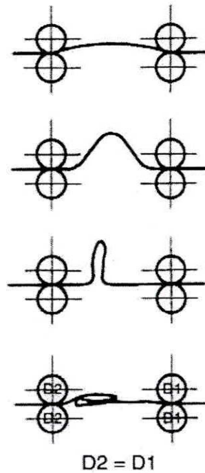
Fig. 2.9 Problemas del conformado por velocidades superficiales distintas entre rodillos
