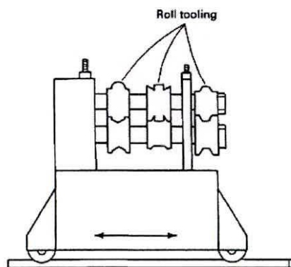
Fig. 1.8 Máquina de lado y lado para conformado
