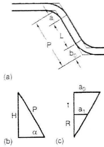
Fig. 2.13 Cálculo del tamaño de sección
