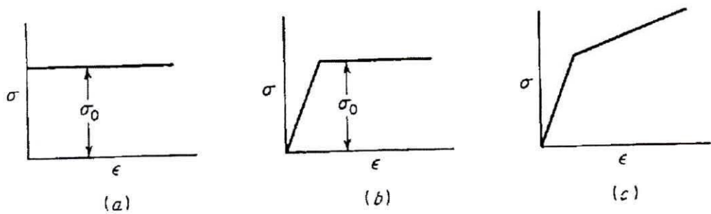
Fig. 1.2 Curvas Esfuerzo-Deformación Idealizadas. (a) Material plástico ideal rígido, (b) Material plástico ideal en la región elástica y (c) Material lineal por tramos.
