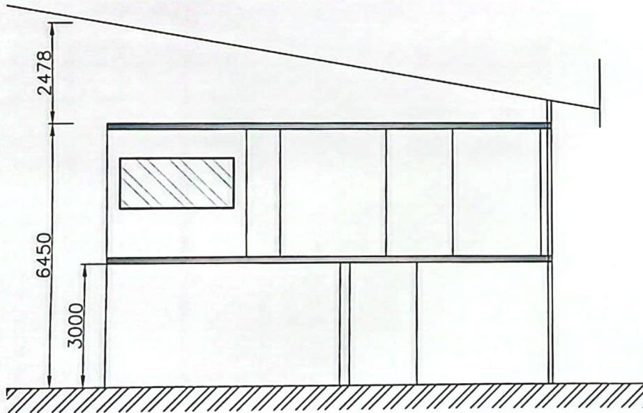
CORTE D-D'
