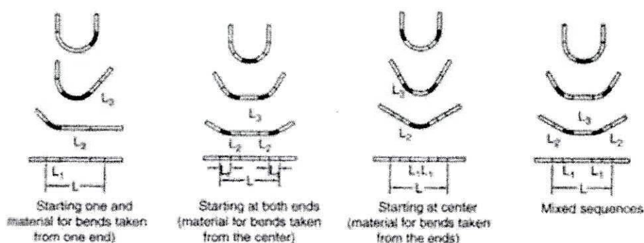
Fig. 2.14 Conformado de radios constantes en tres pasos [6].
