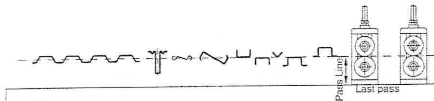
Fig. 2.8 Línea de paso en Máquina de Conformado
