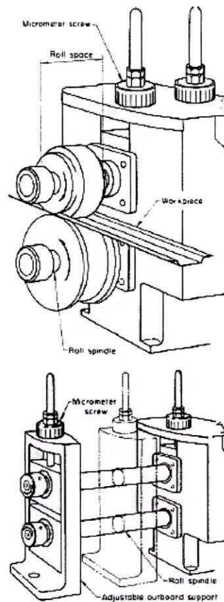
Fig. 1.7 Máquina de eje interior (arriba) y Máquina de eje exterior (abajo)
