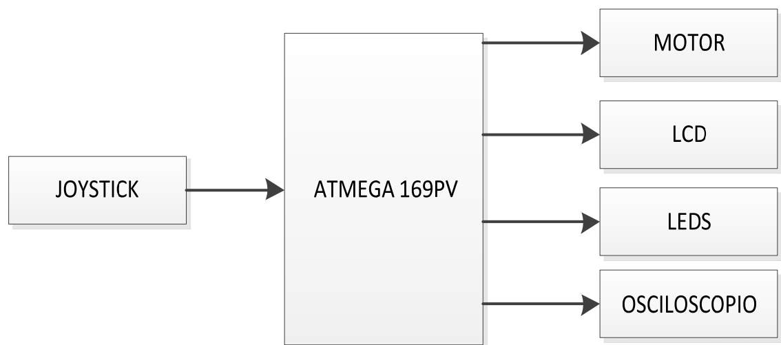
Figura 4.3 Diagrama de Bloques: Motor de 3 velocidades
