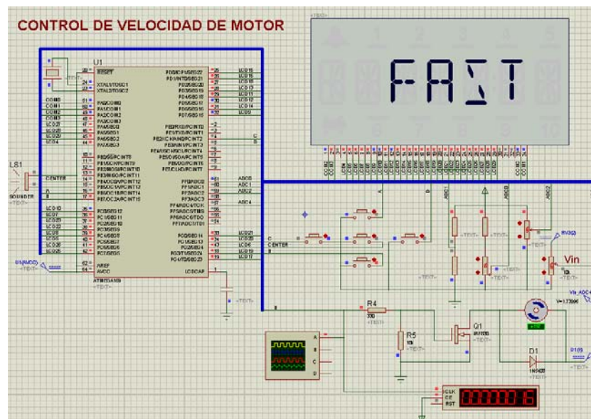
Figura 4.12 Esquemático: Control de velocidad de motor DC
