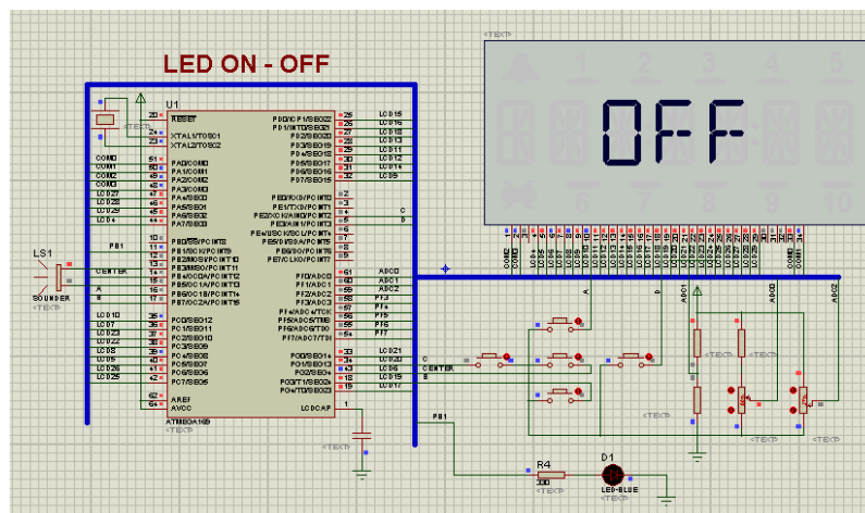
Figura 4.7 Esquemático: Encender/Apagar (Estado OFF)
