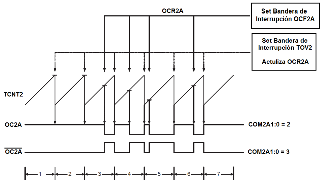
Figura 1.6 Diagrama de tiempos para el modo PWM rápido
