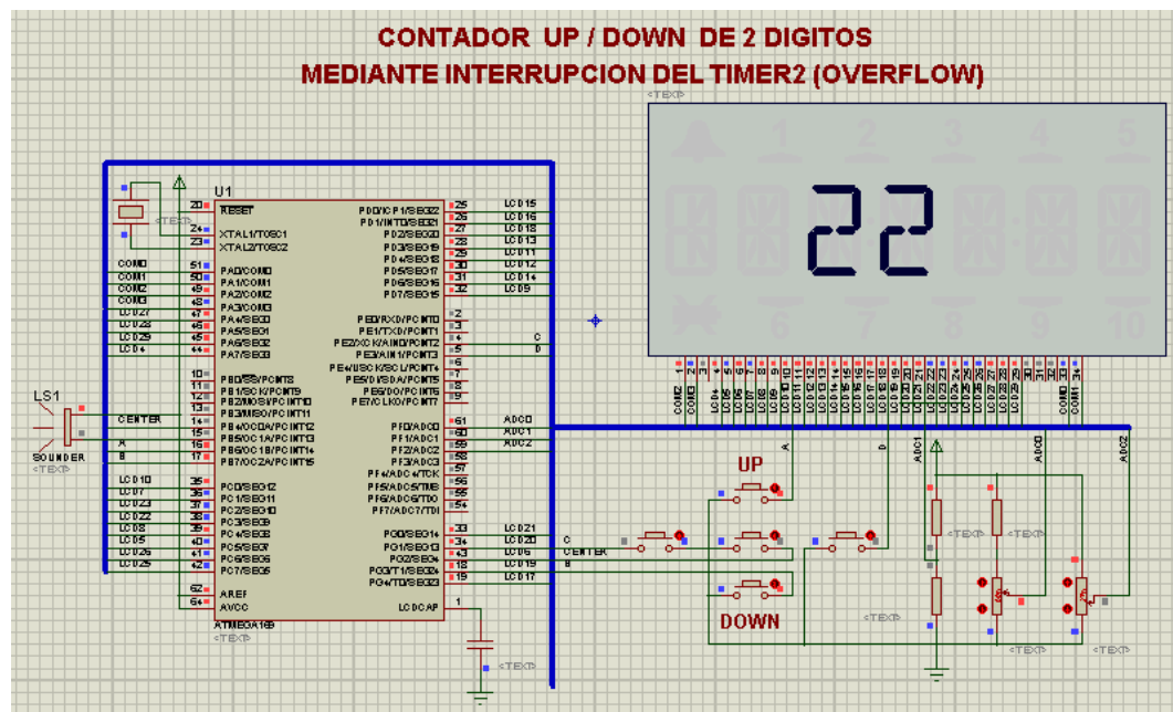
Figura 4.2 Esquemático: Contador UP/DOWN
