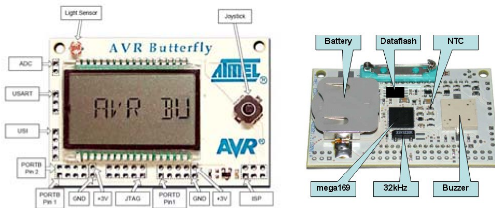
Figura 2.4 AVR Butterfly
