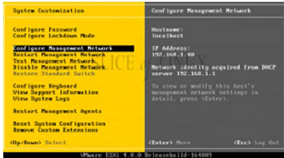
Fig. 3.21 Pantalla para cambiar la configuración de red.
