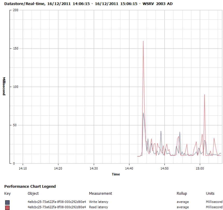
Fig. 4.24 Rendimiento del Datastore en el Active Directory.
