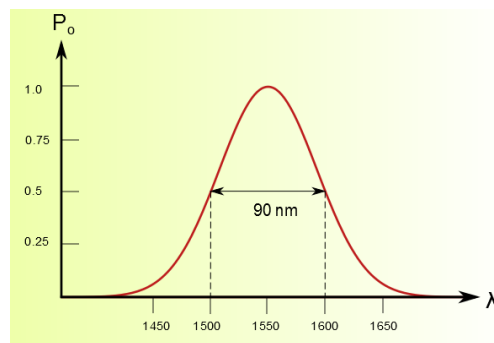
Figura 1. 3 Gráfica potencia vs longitud de onda de un LED
