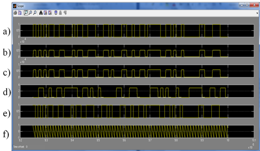
Figura 3. 11 Resultado de la Simulación#3a en el Osciloscopio
