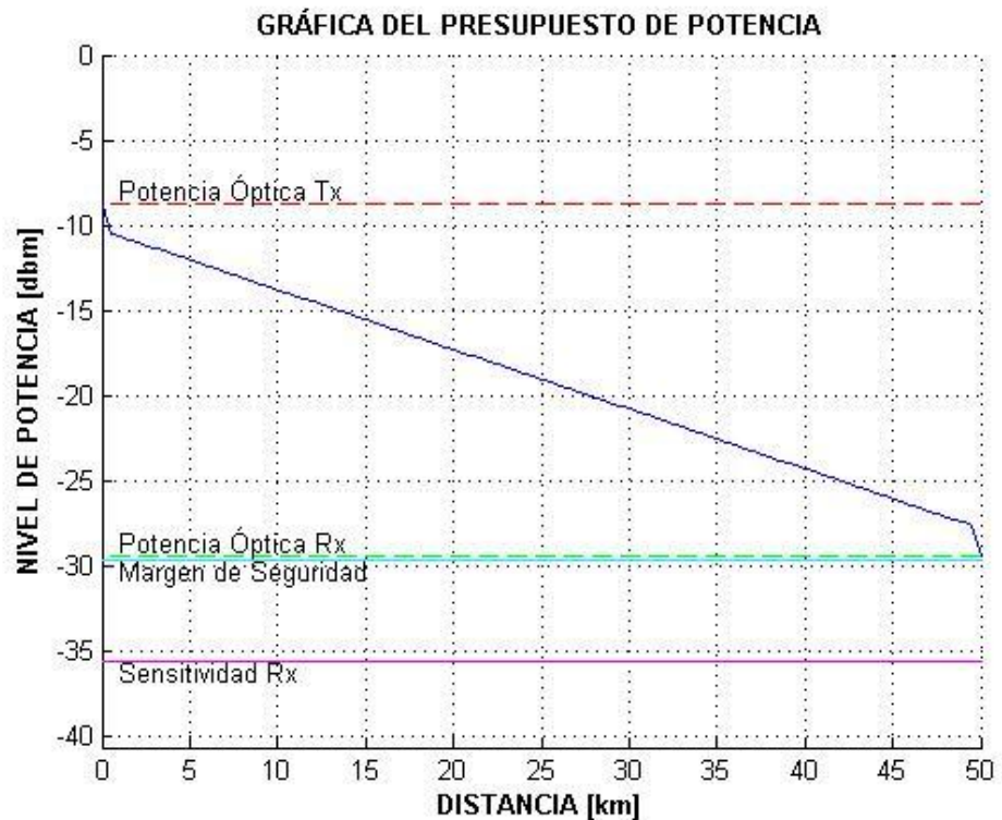
Figura 3. 19 Presupuesto de Potencia#1a
