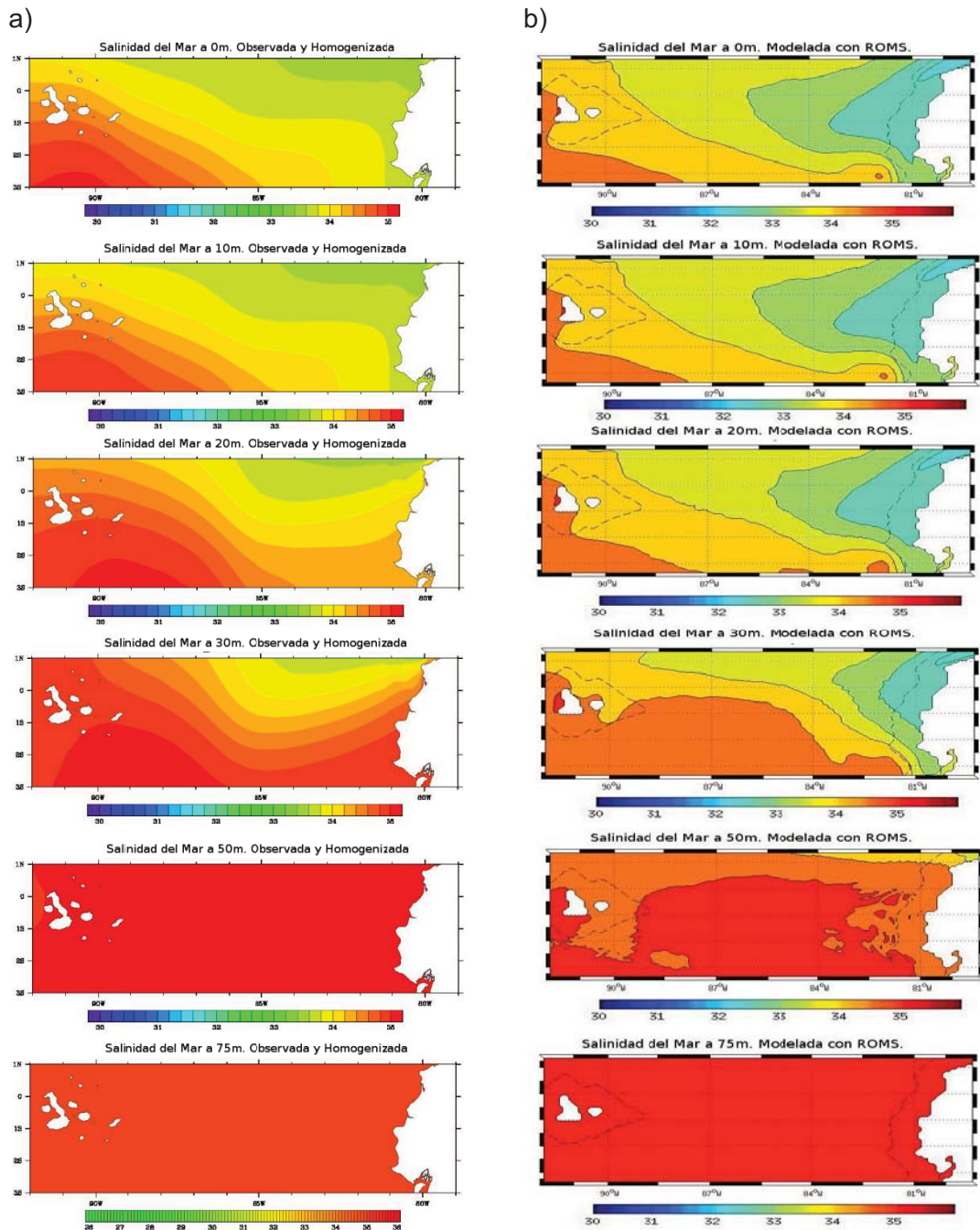
Figura 4.5.- Mapas de Salinidad del Mar del crucero oceanográfico OCT/2005. a) Datos observados y homogenizados Cressman-Poisson y b) Modelado con ROMS
