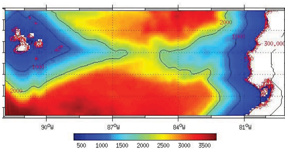
Figura 3.3.- Batimetría del área de estudio
