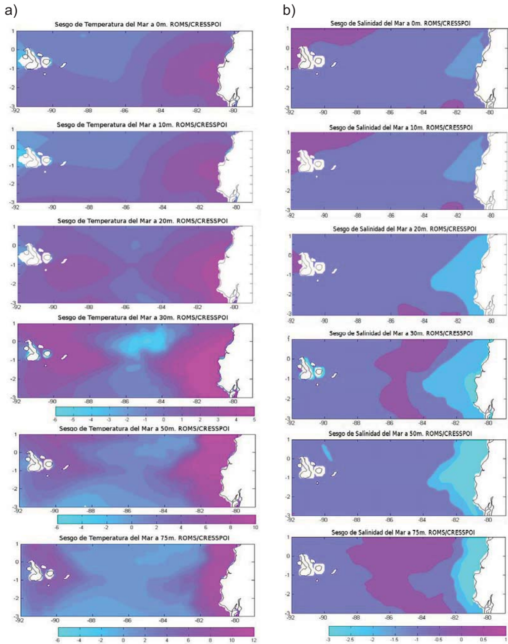
Figura 4.11.- Mapas de Sesgo respecto a los datos del crucero oceanográfico OCT/2005. a) Temperatura del Mar y b) Salinidad.
