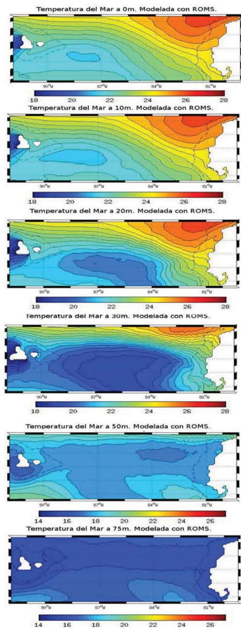
Figura 4.3.- Mapas de temperatura del mar del crucero oceanográfico OCT/2009. a) Datos observados y homogenizados Cressman-Poisson y b) Modelado con ROMS.
