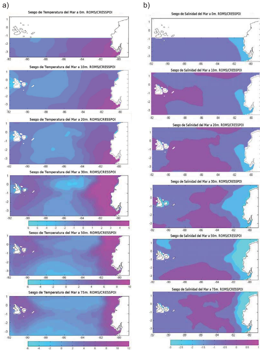
Figura 4.12.- Mapas de Sesgo respecto a los datos del crucero oceanográfico OCT/2009. a) Temperatura del Mar y b) Salinidad.
