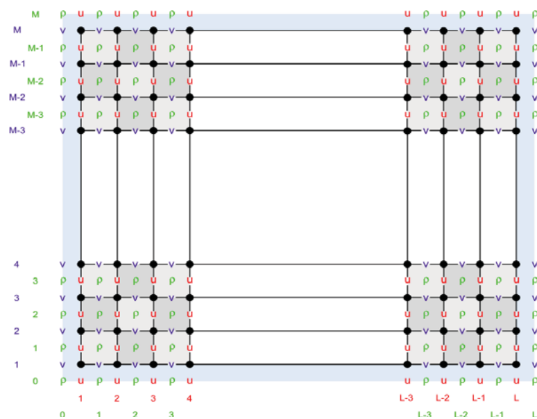
Figura 3.2.- Malla horizontal de ROMS
