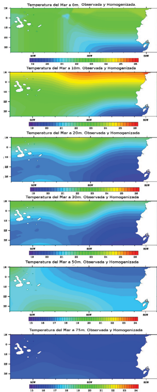
Figura 4.3.- Mapas de temperatura del mar del crucero oceanográfico OCT/2009. a) Datos observados y homogenizados Cressman-Poisson y b) Modelado con ROMS.
