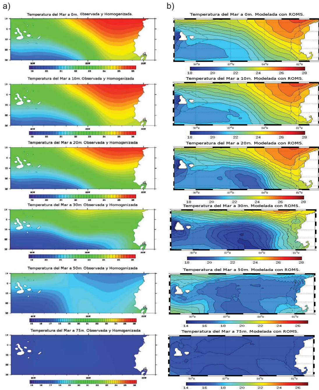
Figura 4.1.- Mapas de temperatura del mar del crucero oceanográfico SEP/2002. a) Datos observados y homogenizados Cressman-Poisson y b) Modelado con ROMS
