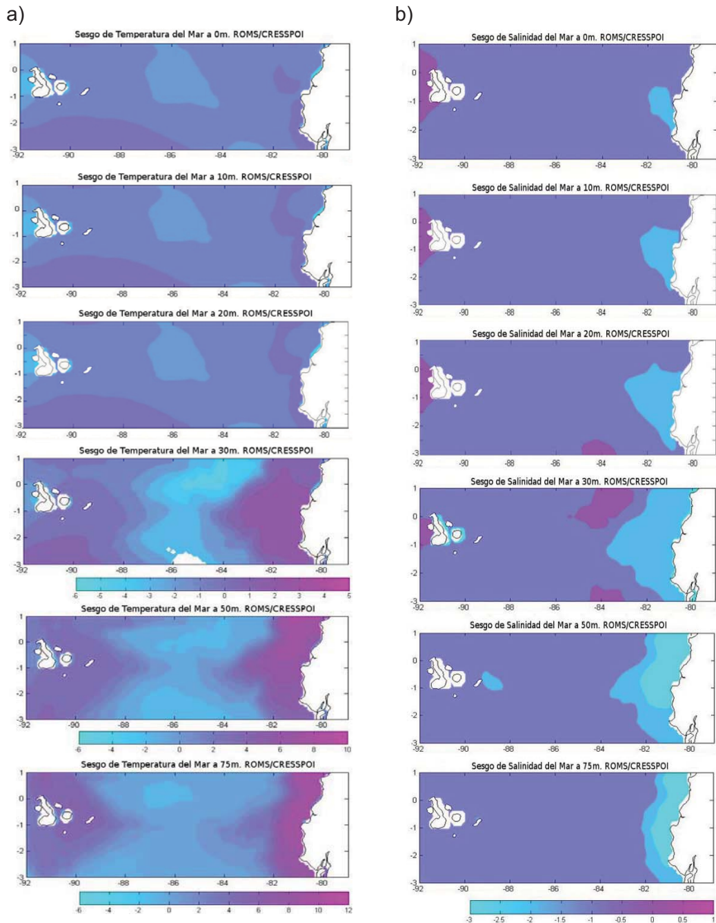
Figura 4.10.- Mapas de Sesgo respecto a los datos del crucero oceanográfico SEP/2002. a) Temperatura del Mar y b) Salinidad.
