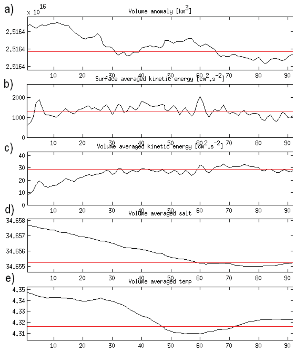
Figura 3.4.- Tiempo de evolución de diferentes variables: anomalía de volumen, promedio de la energía cinética superficial, promedio del volumen de energía cinética, promedio del volumen de salinidad y de temperatura, gráfico (a,b,c,d,e) respectivamente.
