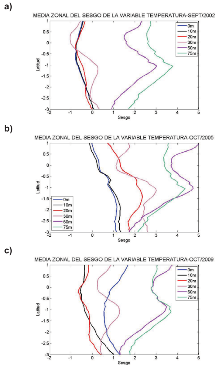
Figura 4.8.- Perfil de sesgo zonal de la temperatura del mar desde la superficie hasta los 75m, para los cruceros oceanográficos: a) SEP/2002 (línea negra), b) OCT/2005 (línea azul) y c) OCT/2009 (línea roja).
