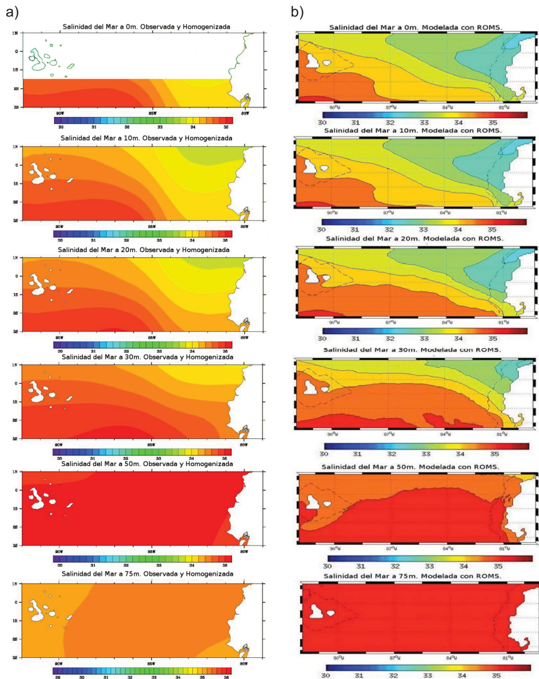
Figura 4.6.- Mapas de salinidad del mar del crucero oceanográfico OCT/2009. a) Datos observados y homogenizados Cressman-Poisson y b) Modelado con ROMS
