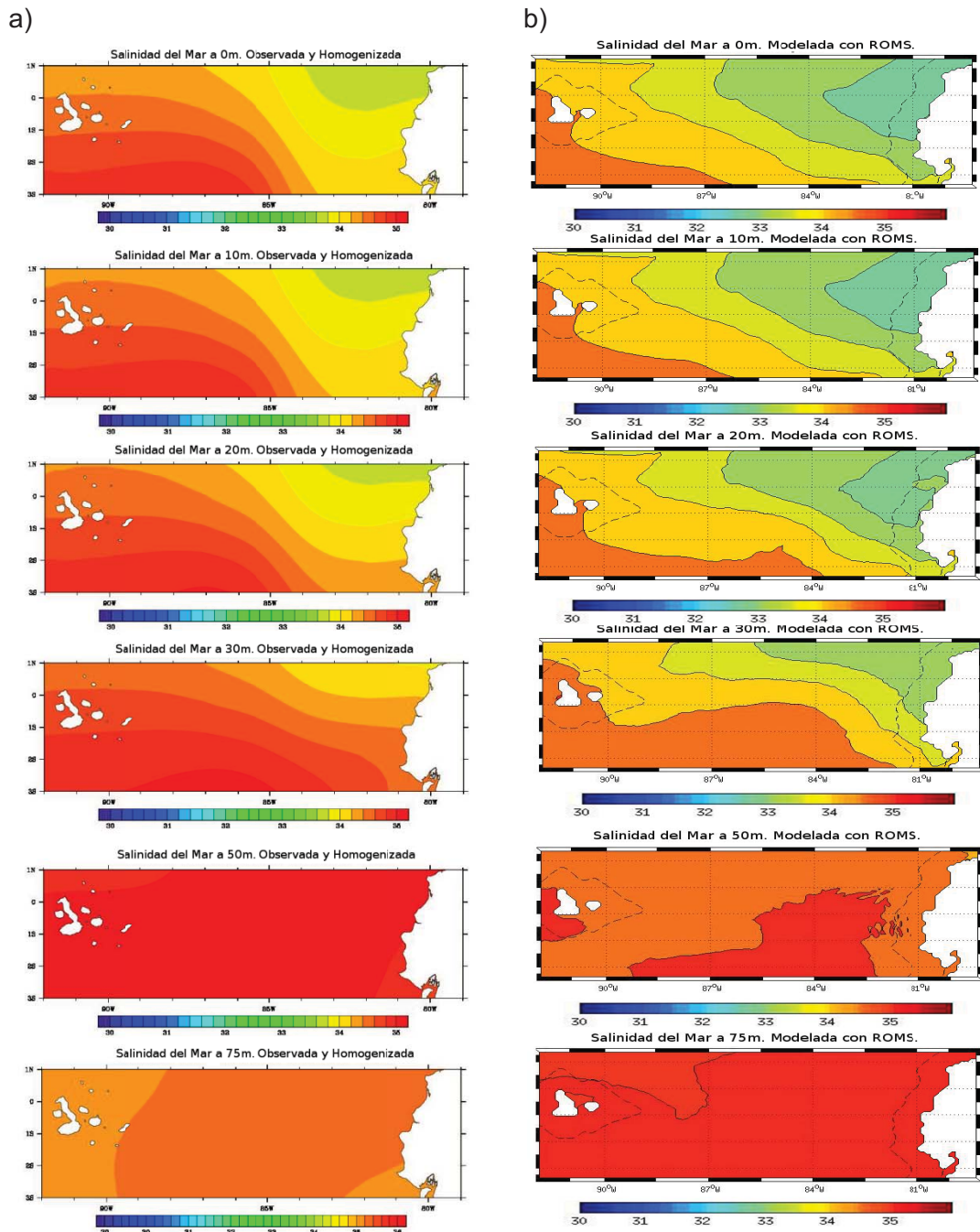
Figura 4.4.- Mapas de salinidad del mar del crucero oceanográfico SEP/2002. a) Datos observados y homogenizados Cressman-Poisson y b) Modelado con ROMS
