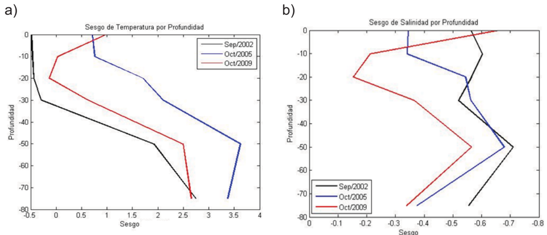
Figura 4.7.- Perfil de sesgo por profundidad (desde la superficie hasta los 75m), para los cruceros oceanográficos SEP/2002, OCT/2005 y OCT/2009; a) temperatura del mar y b) salinidad del mar.
