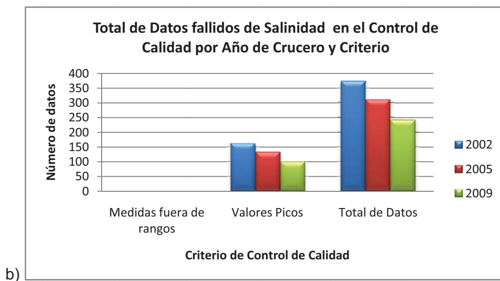
Gráfico 2.1.- Datos Fallidos en el Control de Calidad en los tres períodos de crucero 2002, 2005, 2009. a) Temperatura del Mar y b) Salinidad del Mar.
