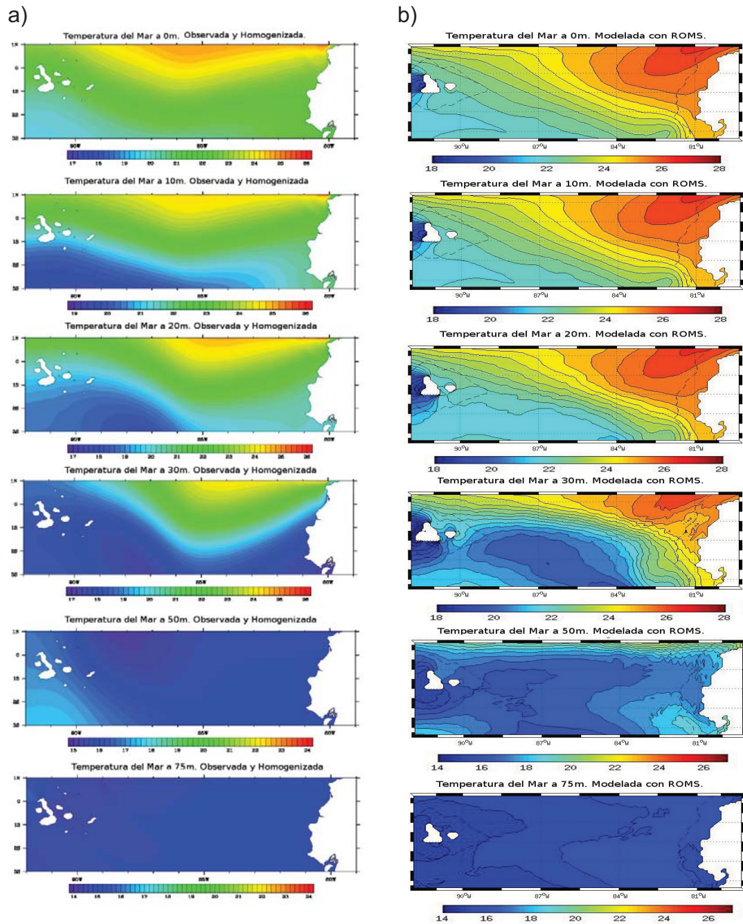
Figura 4.2.- Mapas de temperatura del mar del crucero oceanográfico OCT/2005. a) Datos observados y homogenizados Cressman-Poisson y b) Modelado con ROMS
