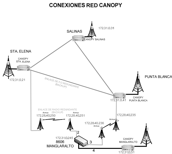
Figura 8. Topología a usar en la ampliación
