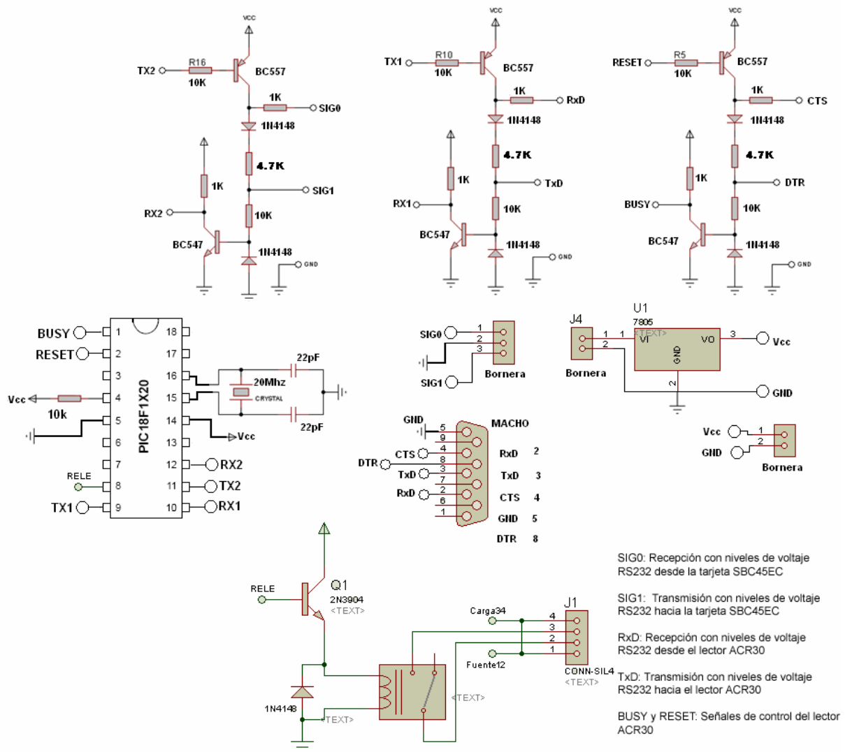
Figura 2.3. Diagrama esquemático del circuito de interfase entre el lector ACR30 y la tarjeta SBC45EC.
