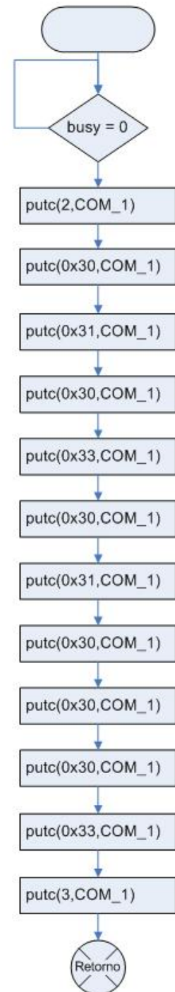
seleccionar_retrazo()
