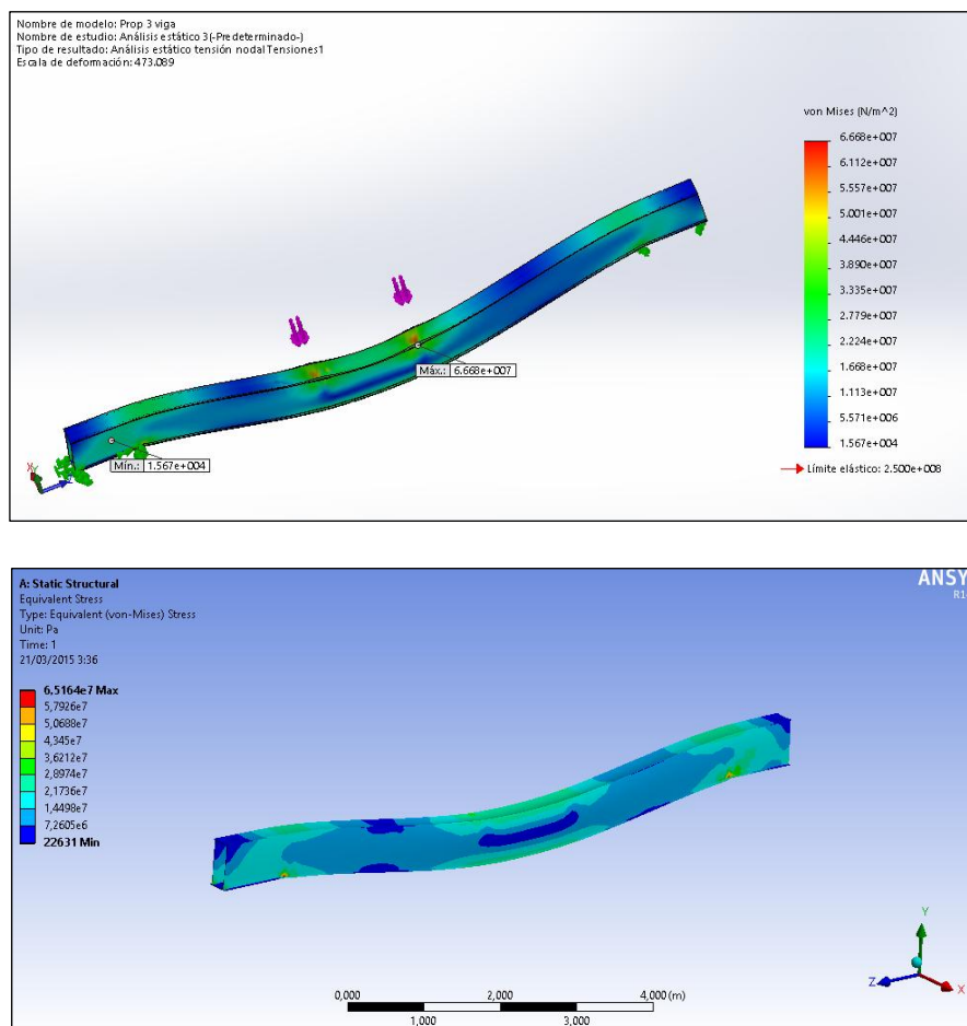
Figura 4.43 Resultados Obtenidos Mediante Solidwork® Y Ansys®; Análisis de Esfuerzos de Von Misses.
