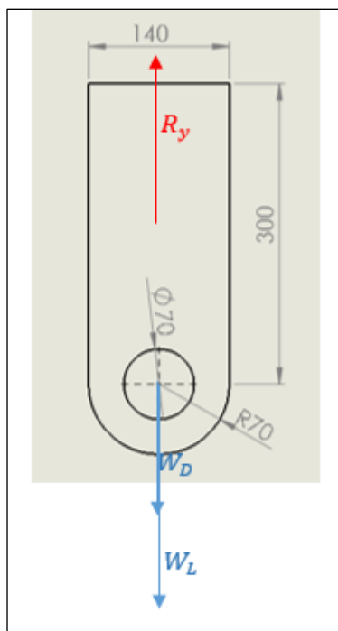
Figura 4.2 Diagrama de Cuerpo Libre de la Placa de Soporte.
