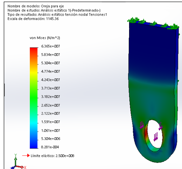
Figura 4.5 Resultados Obtenidos Mediante Solidworks®; Análisis de Esfuerzos de Von Misses.
