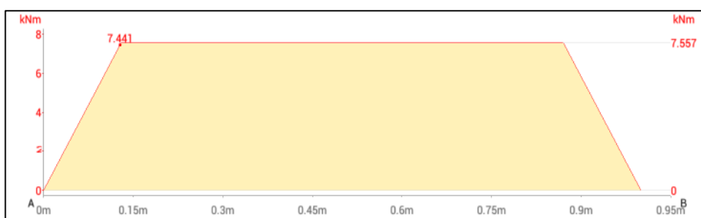
Figura 4.13 Diagrama de Momento de la Viga 1 (Pre Diseño).
