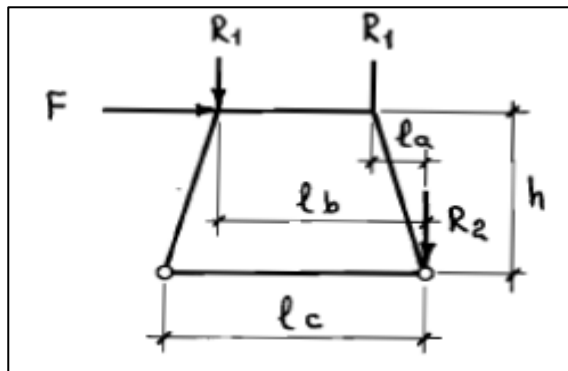
Figura 4.49 Momentos Generados Por El Levantamiento De La Carga. [20]
