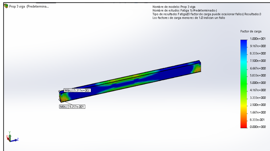
Figura 4.42 Resultados Obtenidos Mediante Solidwork®; Factor de Seguridad para Fatiga.
