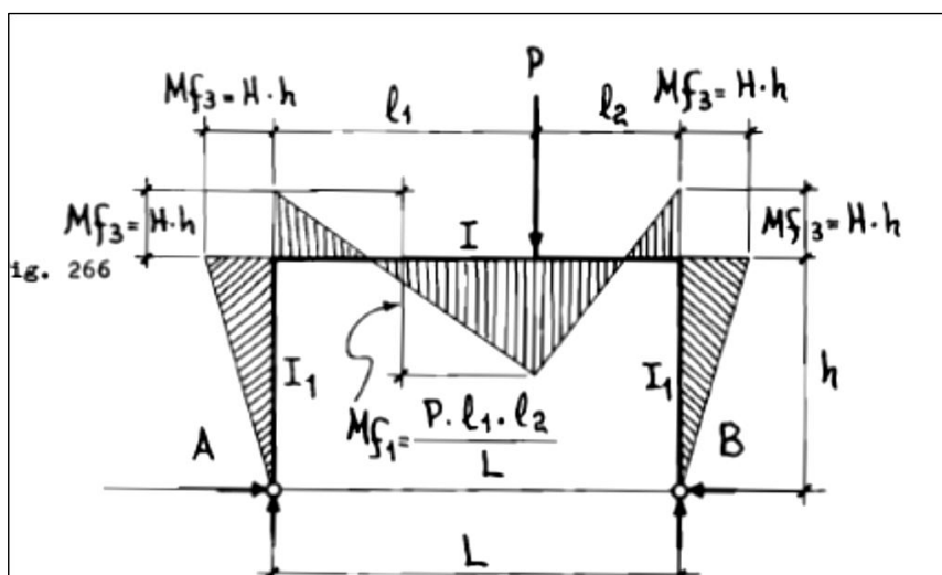
Figura 4.35 Diagrama de Momentos de un Pórtico Articulado. [20]
