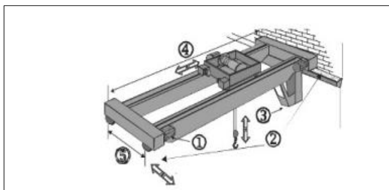
Figura 2.10 Grúa puente. [9]
