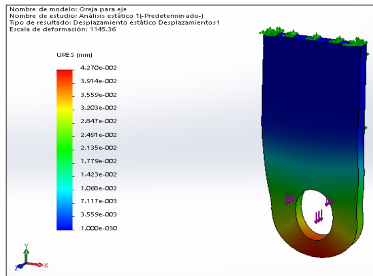
Figura 4.4 Resultados Obtenidos Mediante Solidworks®; Análisis de Deformaciones.
