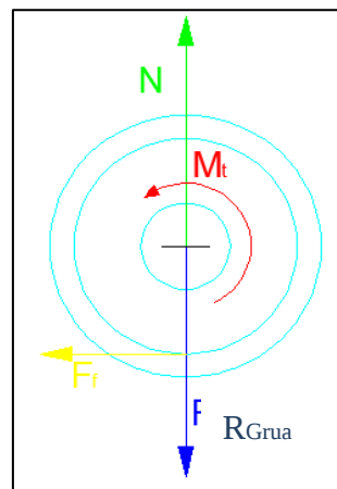
Figura 4.73 Diagrama de Fuerzas de la Rueda.
