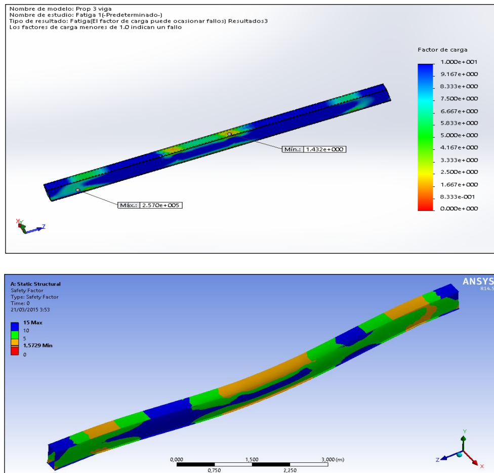
Figura 4.46 Resultados Obtenidos Mediante Solidwork® Y Ansys®; Factor De Seguridad Para Fatiga.
