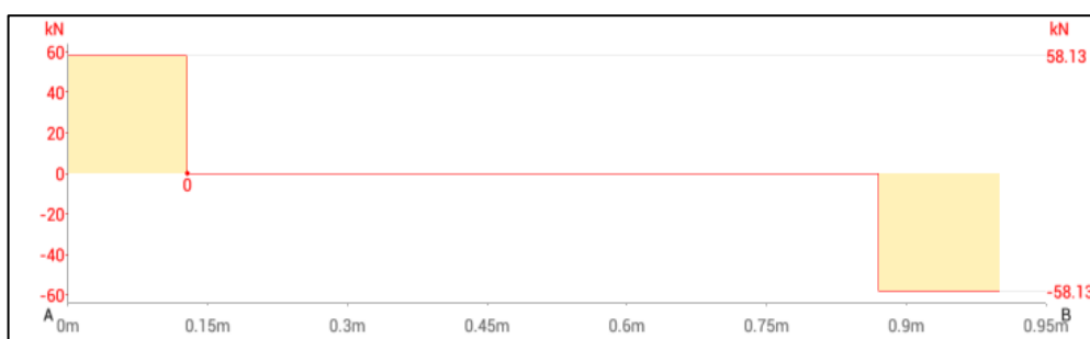
Figura 4.14 Diagrama de Cortante de la Viga 1 (Pre Diseño).
