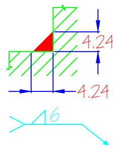
Detalle de soldadura (C) Sin escala
