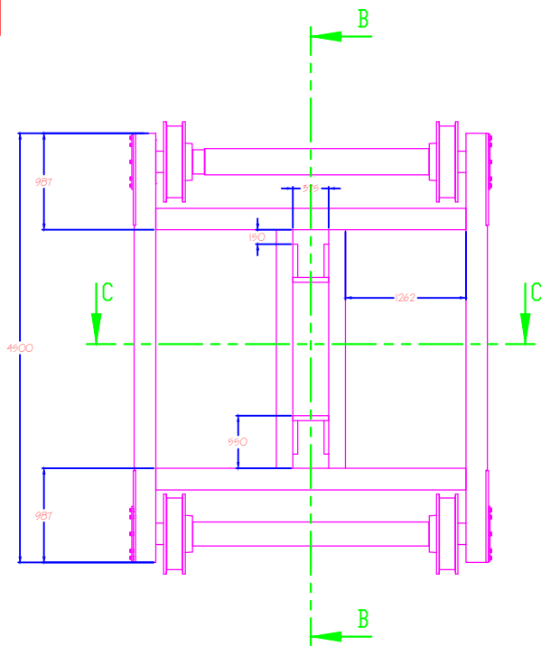
Vista Superior. Trolley
