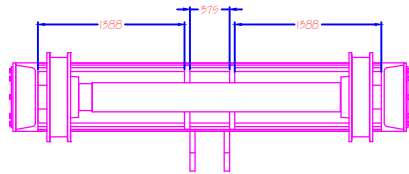
Vista Superior. Trolley
