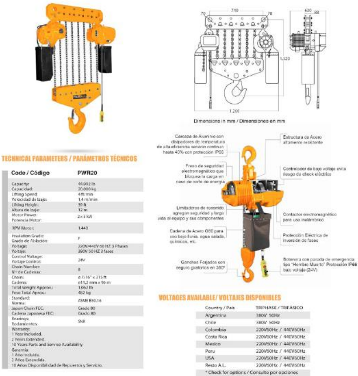
Figura # A2 Características del tecla a utilizar. [26]
