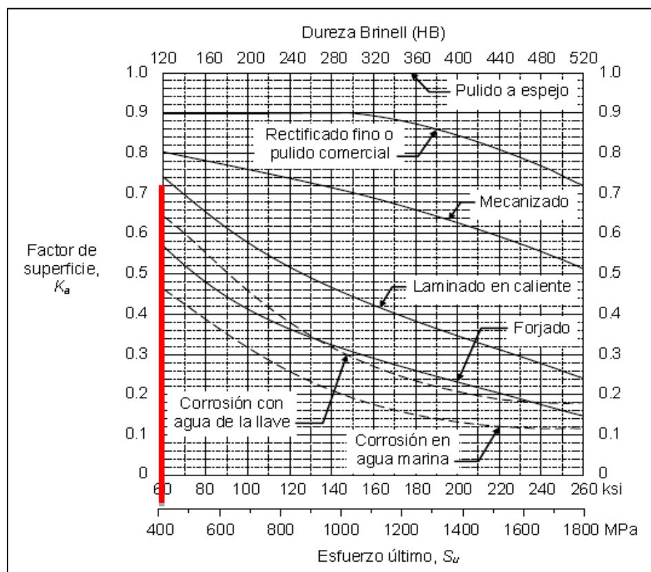
Figura 4.20 Factores de superficie para el acero. [19]
