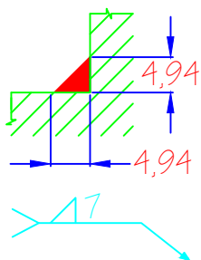
Detalle de soldadura (A) Sin escala
