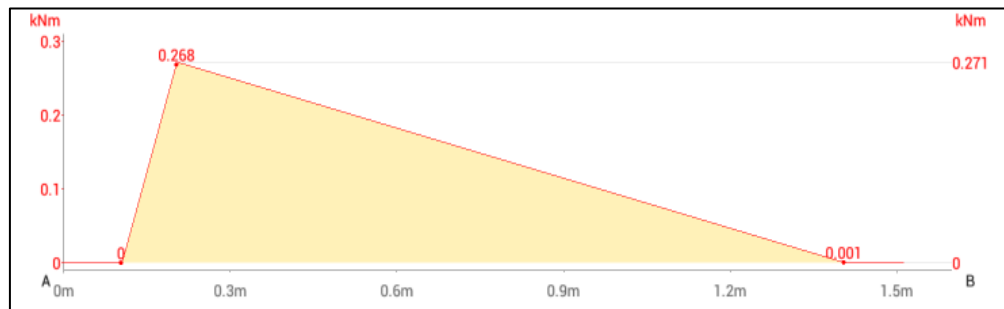
Figura 4.70 Diagrama De Momento En El Plano Z-X.
