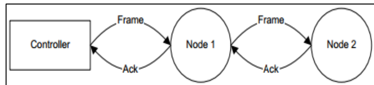
Figura 2.12: Flujo de una trama de tipo Routed Singlecast.
