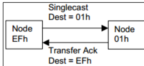
Figura 2.9: Flujo de la trama de una transmisión singlecast.
