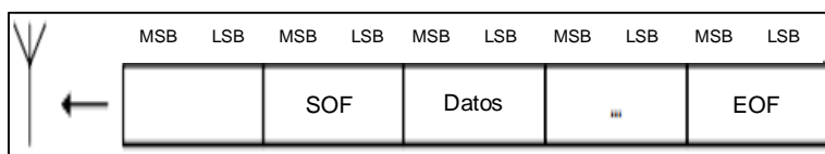
Figura 2.6: Formato de la trama de la capa MAC.
