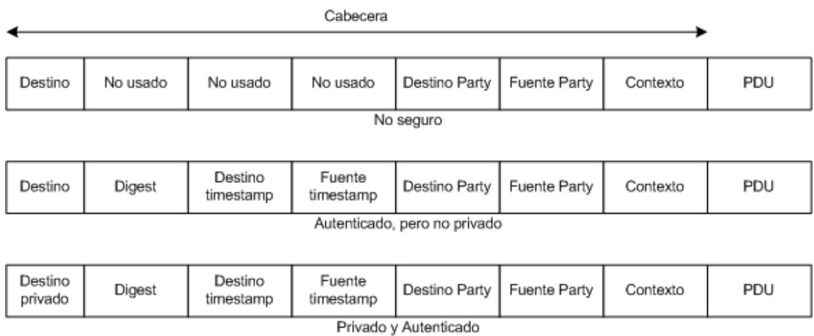
Figura { SEQ Figura \* ARABIC } : Formato del mensaje SNMPv2 (Cabecera detallada) (Ref 1)
