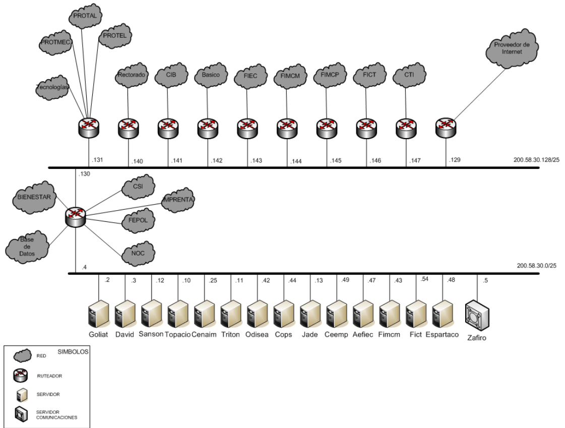
Figura { SEQ Figura \* ARABIC }: Diagrama del Backbone de la ESPOL, Campus Gustavo Galindo
