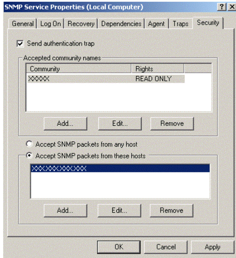
Figura { SEQ Figura \* ARABIC } Configuración del servicio SNMP(seguridad) para Windows 2000
