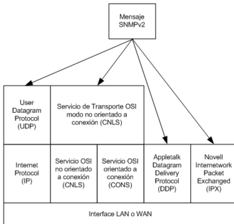
Figura { SEQ Figura \* ARABIC }: Soporte multiprotocolo del SNMPv2 (Ref 1)
