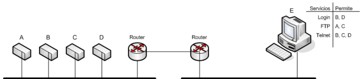
Figura { SEQ Figura \* ARABIC }: Autenticación de Host (Ref 1)
