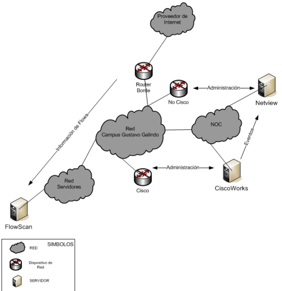
Figura { SEQ Figura \* ARABIC }: Esquema de Administración del Campus Gustavo Galindo
