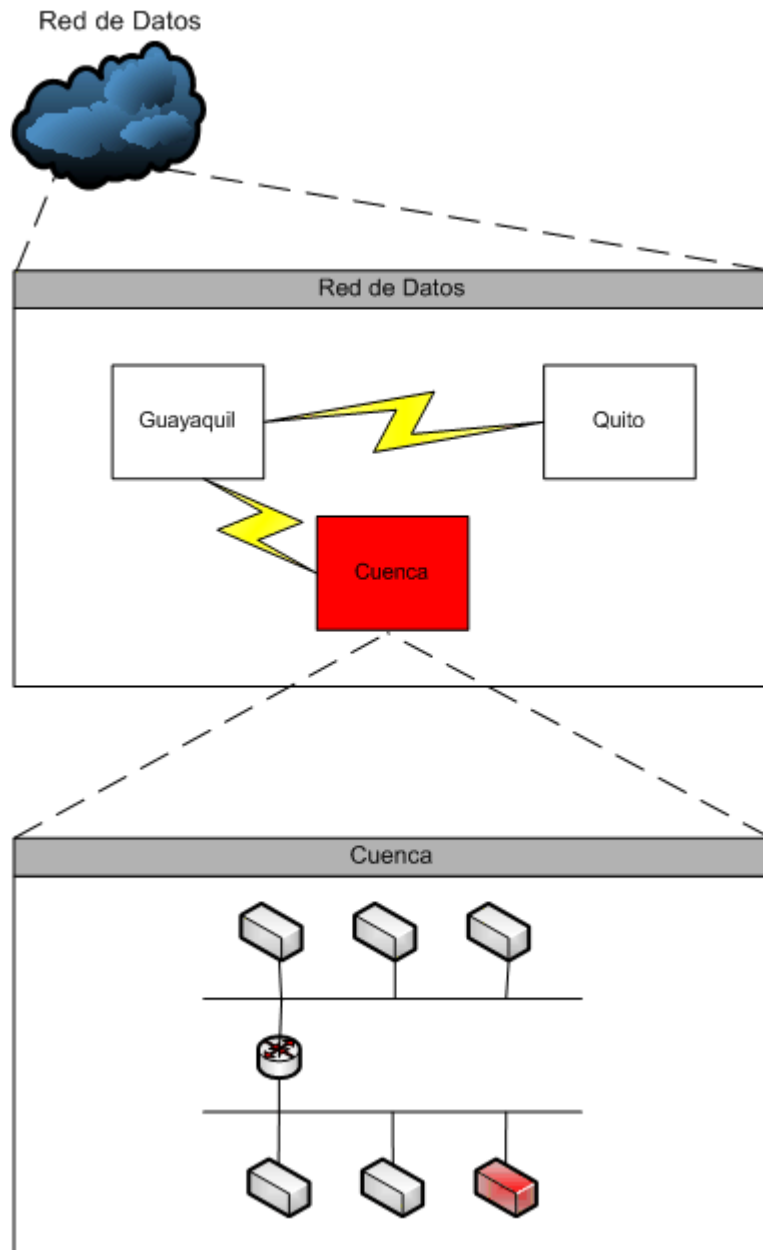
Figura { SEQ Figura \* ARABIC }: Mapa jerárquico usado para aislar fallas (Ref 1)
