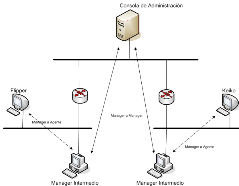
Figura { SEQ Figura \* ARABIC }: Arquitectura de administración del SNMPv2 (Ref 1)
