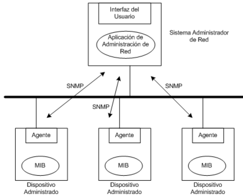
Figura { SEQ Figura \* ARABIC }: Modelo de Agente/Estación del protocolo SNMP (Ref
