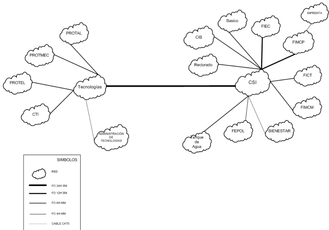
Figura { SEQ Figura \* ARABIC }: Enlaces de datos en el Campus Gustavo Galindo
