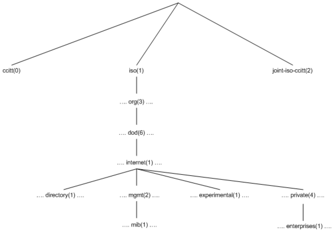
Figura { SEQ Figura \* ARABIC }: Estructura superior del árbol MIB (Ref 1)
