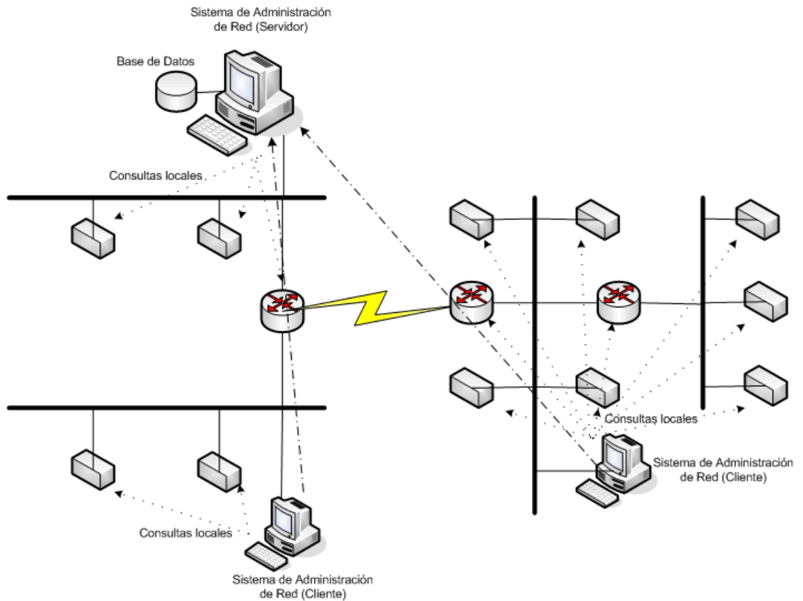
Figura { SEQ Figura \* ARABIC }: Arquitectura Jerárquica (Ref 1)
