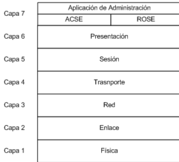
Figura { SEQ Figura \* ARABIC }: El protocolo CMIP en el modelo de referencia de la OSI (Ref 1)
