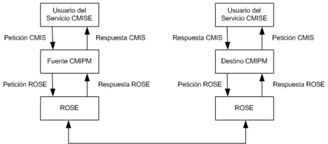
Figura { SEQ Figura \* ARABIC }: Flujo de una petición de servicio CMIS entre doe CMISE-service-user (Ref 1)
