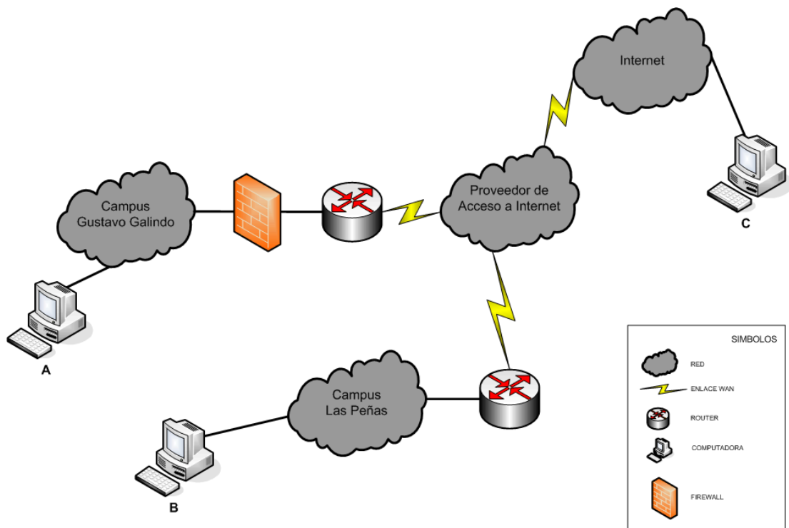
Figura { SEQ Figura \* ARABIC }: Diagrama Lógico de conexión entre Gustavo Galindo, Peñas e Internet
