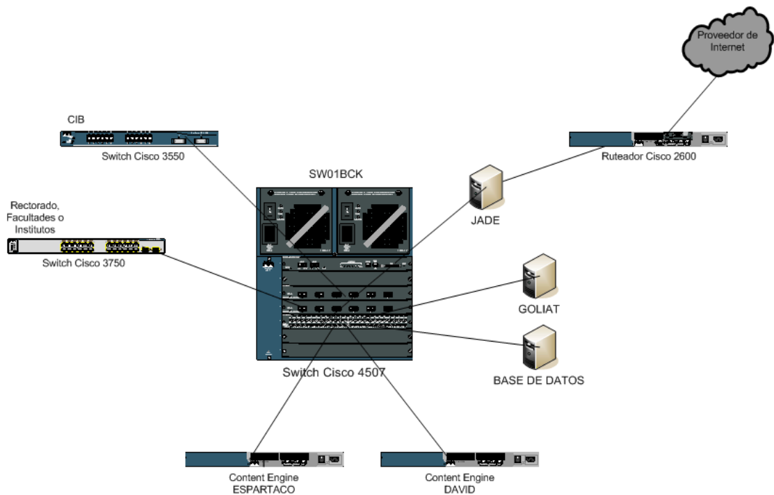
Figura { SEQ Figura \* ARABIC }: Equipos que componen el Backbone de la ESPOL
