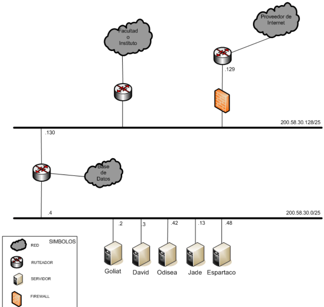
Figura { SEQ Figura \* ARABIC }: Interconexión de los componentes de Red en el Campus Gustavo Galindo
