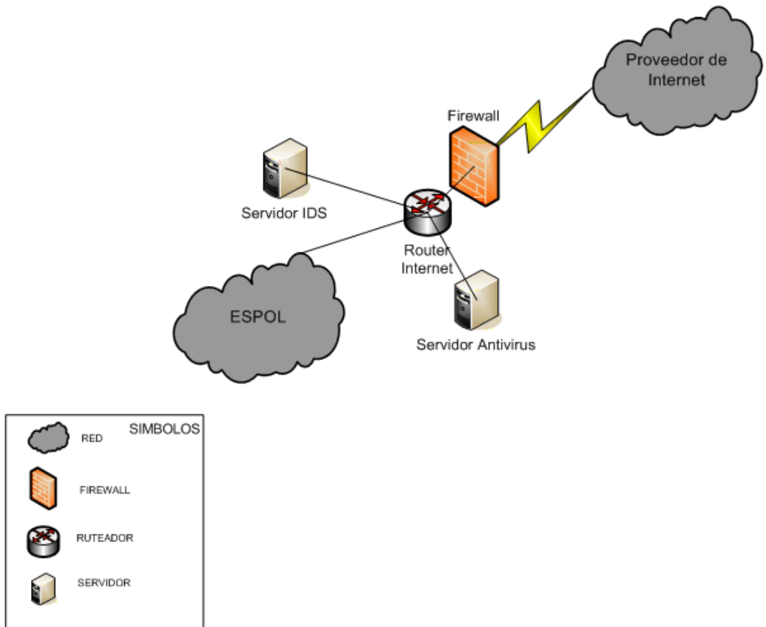
Figura { SEQ Figura \* ARABIC }: Esquema de conexión a Internet
