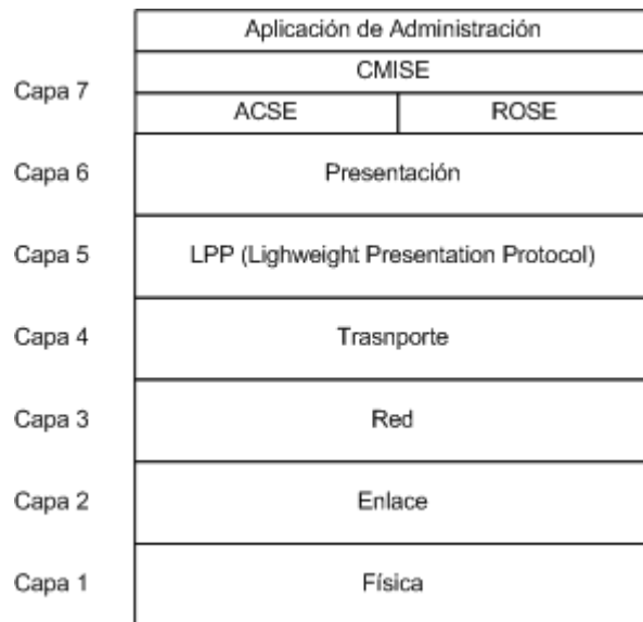
Figura { SEQ Figura \* ARABIC }: El protocolo CMOT en el modelo de referencia de la OSI (Ref 1)
