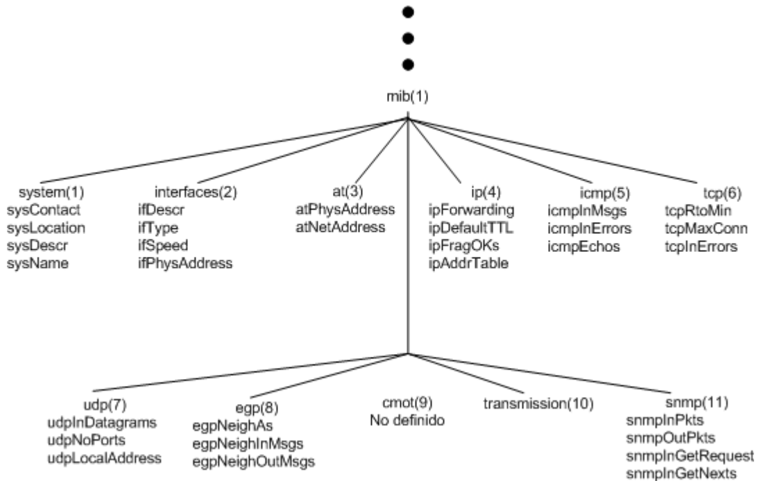
Figura { SEQ Figura \* ARABIC }: Estructura del subárbol mgmt(2) y algunos objetos MIB-II (Ref 1)
