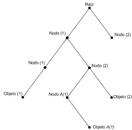
Figura { SEQ Figura \* ARABIC }: Ejemplo de un árbol ASN.1 (Ref 1)
