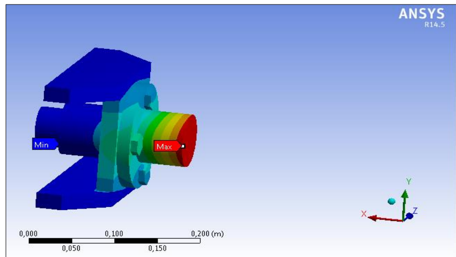
FIGURA 3.36. SIMULACIÒN DE LA DEFORMACIÒN MÁXIMA EN EL CONJUNTO RUEDA EJE
