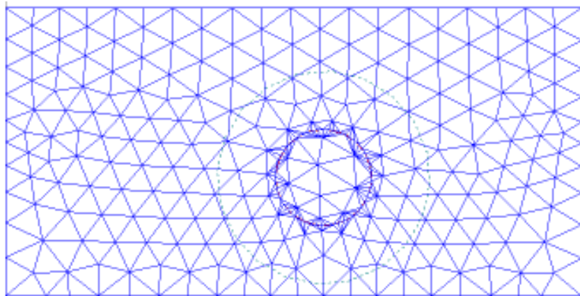
FIGURA 3.5. NUEVA MALLA LUEGO DE REFINAR LA MALLA ORIGINAL ALREDEDOR DEL CÍRCULO [18]
