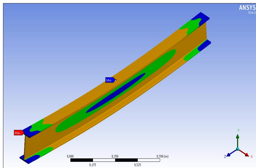
FIGURA 3.33. SIMULACIÒN DEL FACTOR DE SEGURIDAD EN LA VIGA
