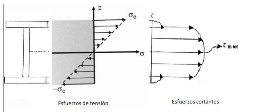
FIGURA 2.10. ESFUERZOS DE Tensión Y ESFUERZOS CORTANTES EN LA VIGA [8]
