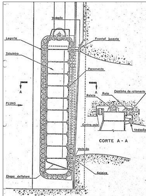
FIGURA 1.3. COMPUERTA TIPO LAGARTO [12]
