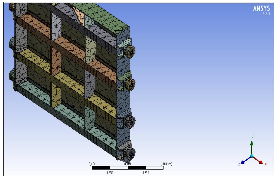
FIGURA 3.30. MALLADO TETRAÉDRICO
