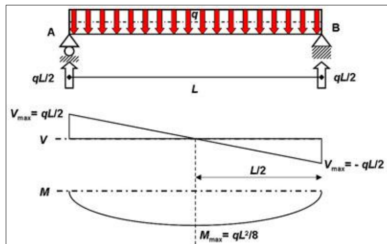
FIGURA 3.18. FUERZAS APLICADAS SOBRE LAS VIGAS HORIZONTALES [9]
