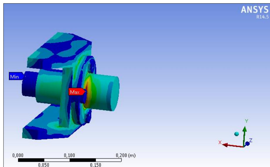
FIGURA 3.37. SIMULACIÒN DEL ESFUERZO MÁXIMO CORTANTE EN EL CONJUNTO RUEDA EJE
