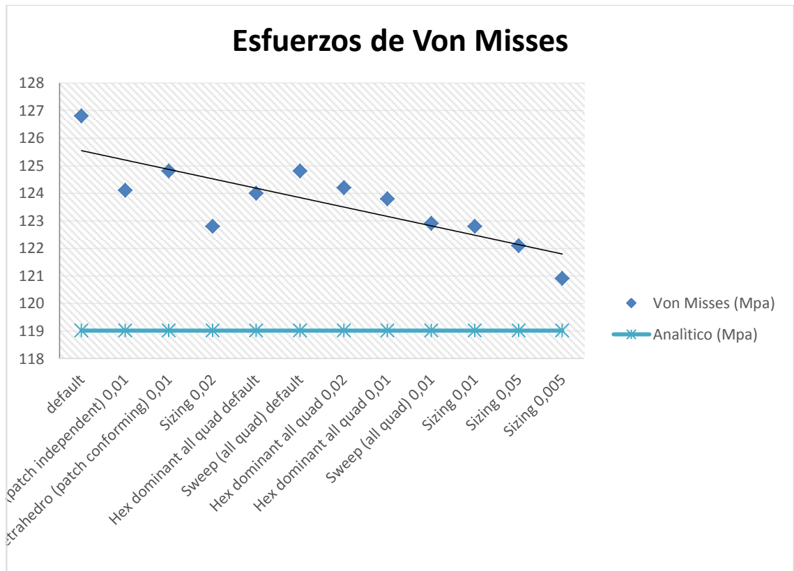
FIGURA 4.1. ESFUERZOS DE VON MISSES SOBRE LA VIGA VS TIPOS DE ELEMENTOS FEM
