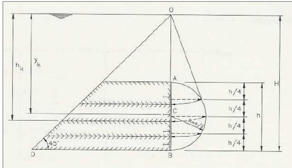
FIGURA 2.3. COMPUERTAS PLANAS SUMERGIDAS- DIVISIÓN DEL DIAGRAMA DE PRESIÓN EN 4 PARTES IGUALES [12]
