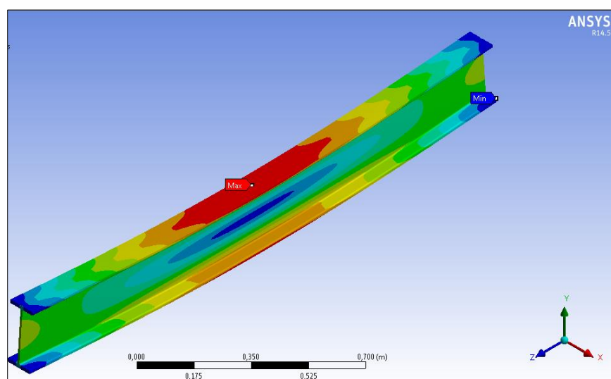
FIGURA 3.34. SIMULACIÒN DEL ESFUERZO DE VON MISSES EN LA VIGA
