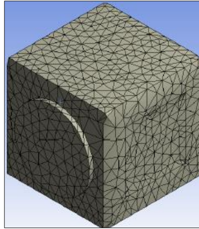
FIGURA 3.14. TIPO DE MALLADO PATCH INDEPENDENT [3]
