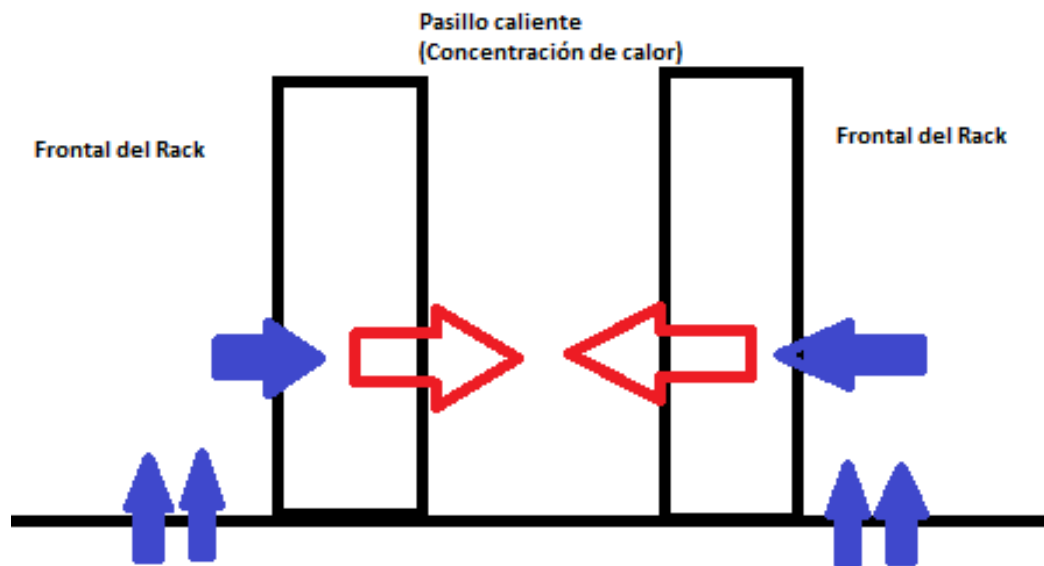
Figura 2.2 Pasillo Caliente y Pasillo Frío [2]
