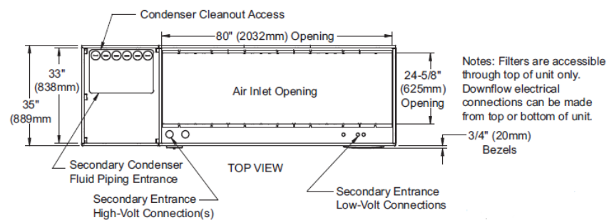
Figura 3.7 Dimensiones Equipo de Climatización DS 077 TOP VIEW [17]
