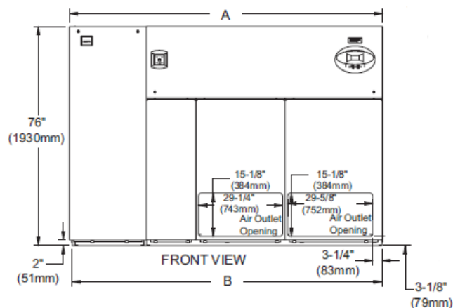
Figura 3.8 Dimensiones Equipo de Climatización DS 077 FRONT VIEW [17]
