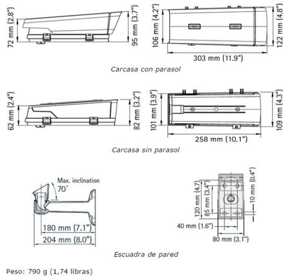
Figura 3.12 Dimensiones de Cámara IP Axis M1114-E [21]
