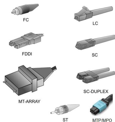
Figura 2.6 Tipos de Conectores de FO [7]
