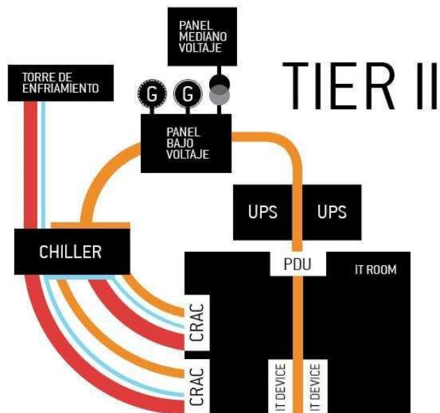
Figura 2.12 Modelo de Tier II: Infraestructura del Site con componentes Redundantes [12]
