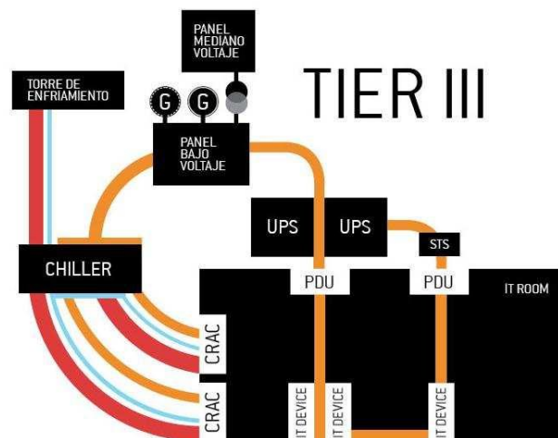
Figura 2.13 Modelo de Tier III: Infraestructura del Site concurrentemente mantenible [12]
