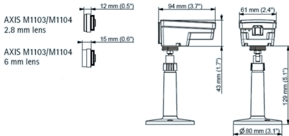
Figura 3.11 Dimensiones de Cámara IP Axis M1103[20]
