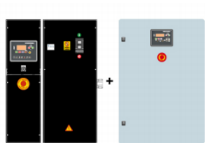
Figura 3.5 Cuadro de Control AS5 + CC2 [16]
