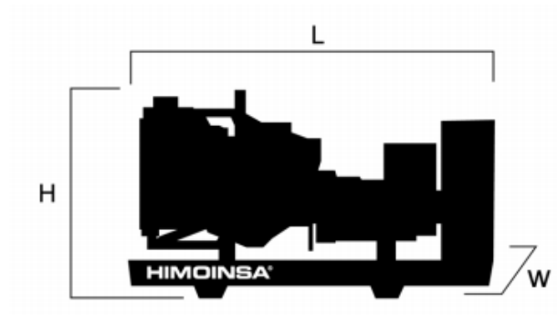
Figura 3.4 Dimensiones de Generador Himoinsa HSW-500 T5 [15]
