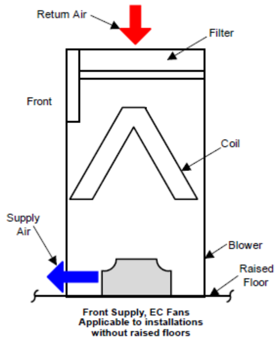
Figura 3.6 Configuración del Blower [17]
