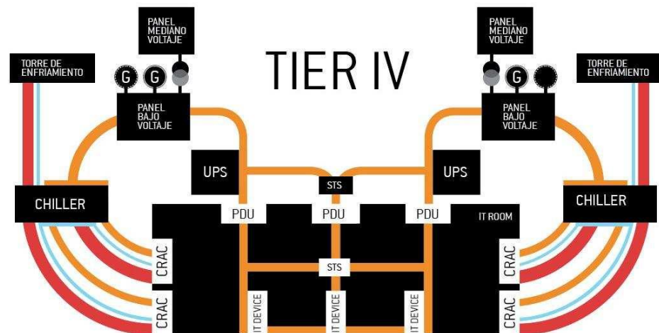
Figura 2.14 Modelo de Tier IV: Infraestructura del Site tolerante a fallas [12]
