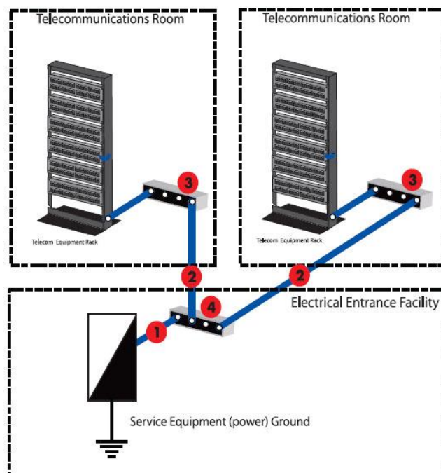
Figura 2.5 Puesta a Tierra para Cableado de Redes [5]
