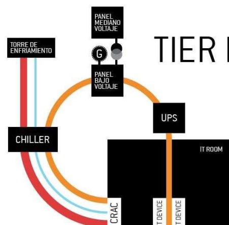
Figura 2.11 Modelo de Tier I: Infraestructura Básica [12]
