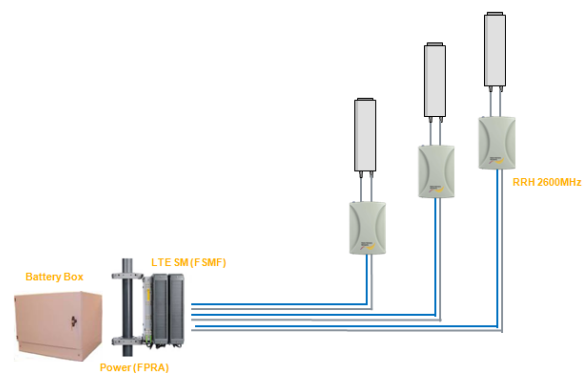
Figura 7: Solución eNodeB Flexi Multiradio distribuida [6]
