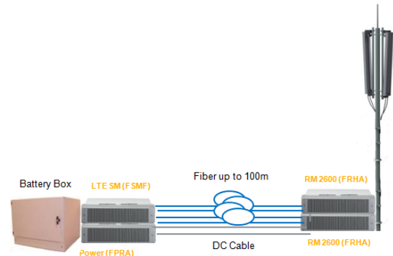
Figura 6: Solución eNodeB Flexi Multiradio concentrada [6]
