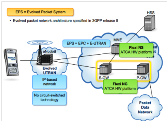
Figura 2: Arquitectura de red LTE [1]
