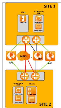
Figura 5: Diseño de alto nivel de EPC LTE [5]
