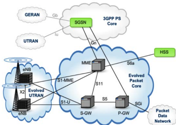
Figura 3: Interfaces de red LTE
