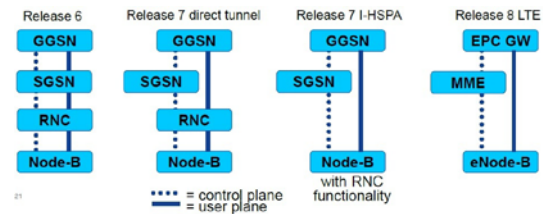
Figura 1: Evolución de arquitectura de red móvil [3]
