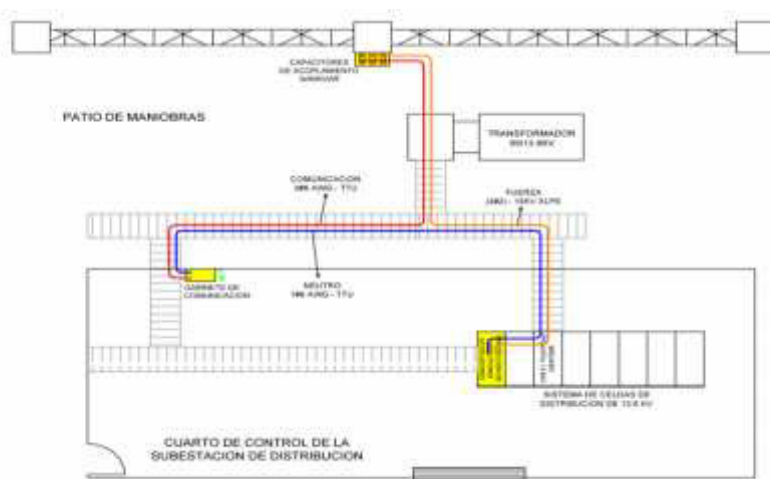
Plano de implantación de Subestación con ubicación de equipos del Sistema de Tele medición
