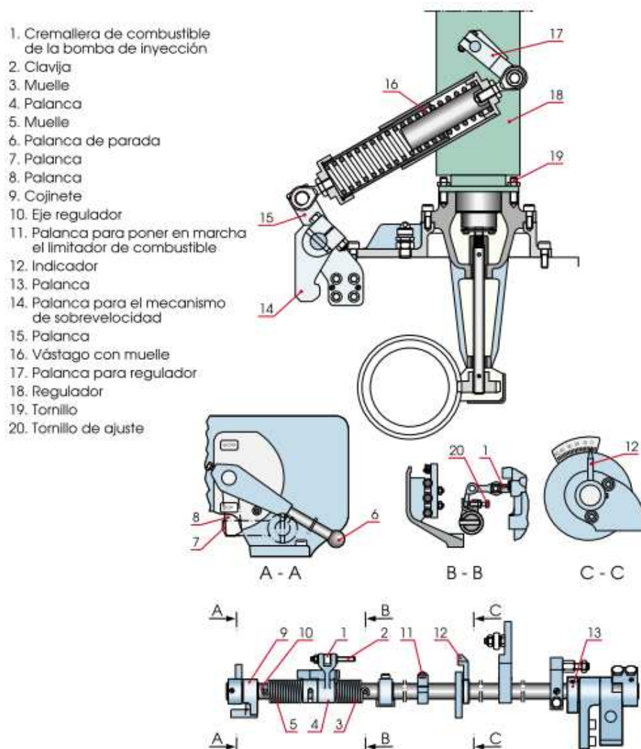
FIGURA 2.15 MECANISMO DE CONTROL.
