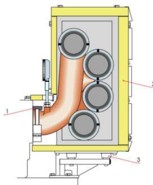
FIGURA 2.13 SISTEMA DE GASES DE ESCAPE.
