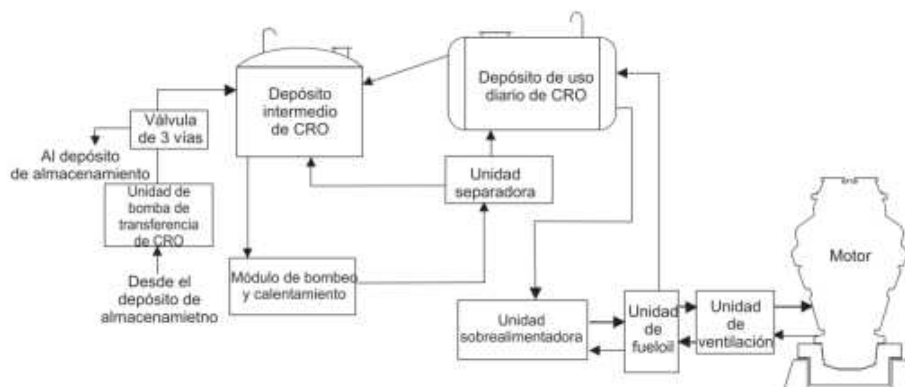
FIGURA 2.8 SISTEMA DE COMBUSTIBLE.
