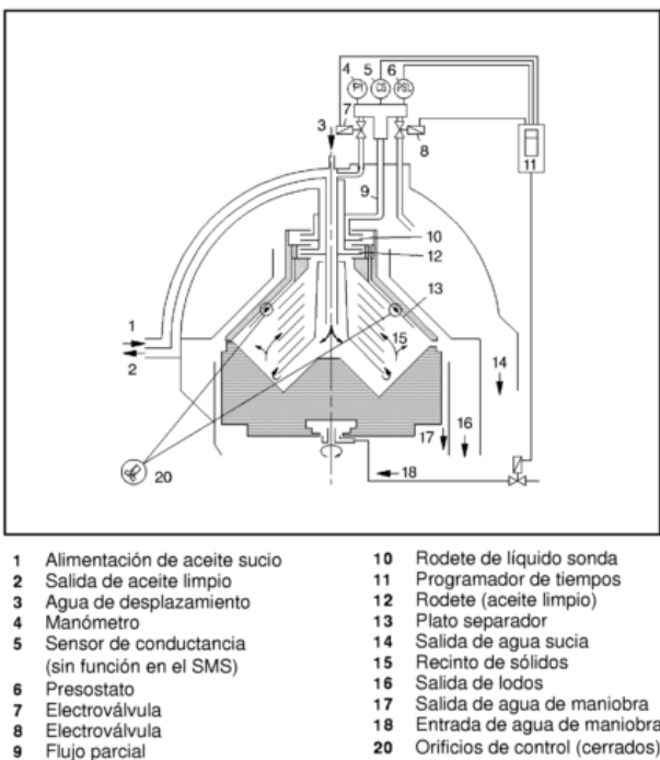
FIGURA 2.18 SISTEMA DE CONTROL DEL RECINTO DE LODOS (SMS) PARA TRATAMIENTO DEL COMBUSTIBLE.
