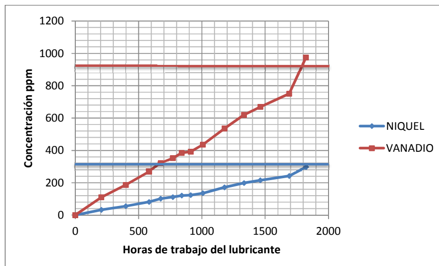
FIGURA 3.11 ANÁLISIS DE CONTAMINACIÓN DEL ACEITE POR NÍQUEL Y VANADIO.
