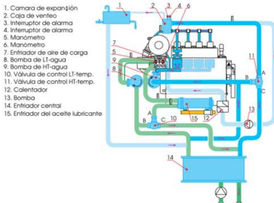
FIGURA 2.12 SISTEMA DE ENFRIAMIENTO.
