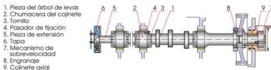
FIGURA 2.5 ÁRBOL DE LEVAS.
