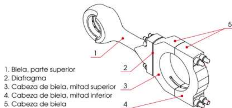
FIGURA 2.2 BIELA DEL MOTOR.
