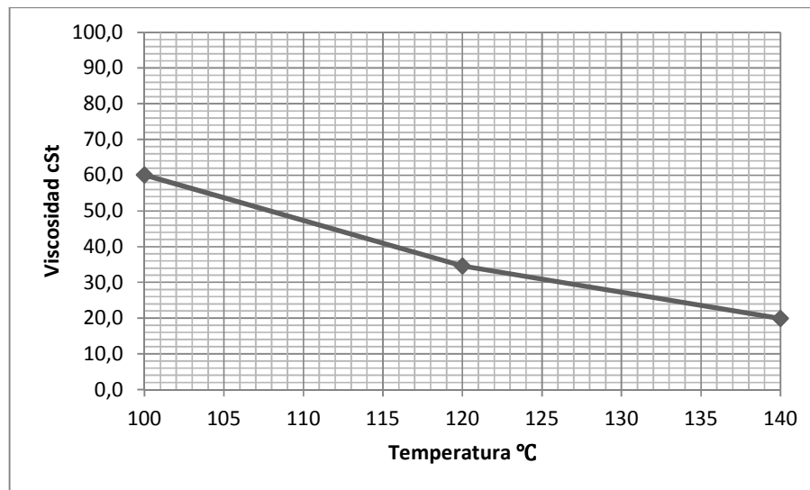
FIGURA 3.6 CURVA DE VISCOSIDAD-TEMPERATURA DEL CRUDO.
