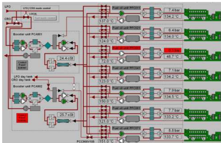
FIGURA 4.1 MODIFICACIÓN DE LA TEMPERATURA DE COMBUSTIBLE.
