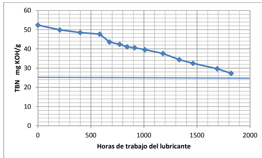
FIGURA 3.9 ANÁLISIS DEL TBN.
