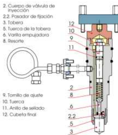
FIGURA 2.7 VÁLVULA DE INYECCIÓN (INYECTOR).
