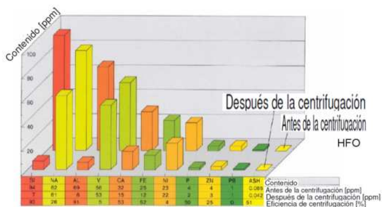
FIGURA 3.3 PORCENTAJE ESPERADO DE REMOCIÓN DE IMPUREZAS.
