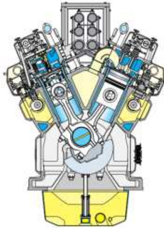
FIGURA 2.1 SECCIÓN TRANSVERSAL DEL MOTOR WARTSILA.
