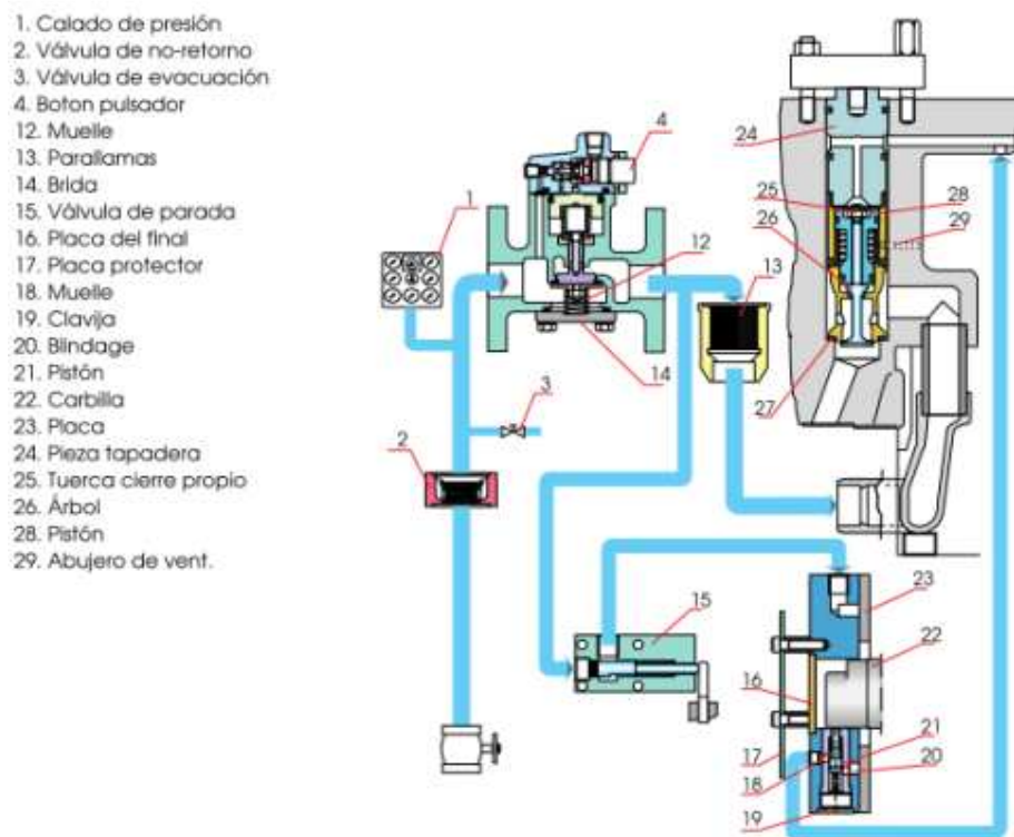
FIGURA 2.14 SISTEMA DE AIRE DE ARRANQUE.
