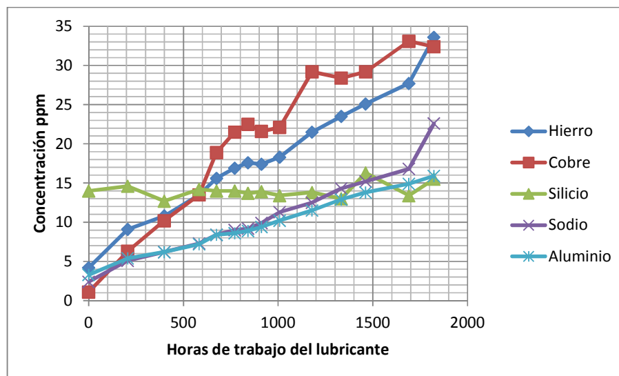
FIGURA 3.12 ANÁLISIS DE METALES EN EL ACEITE LUBRICANTE.
