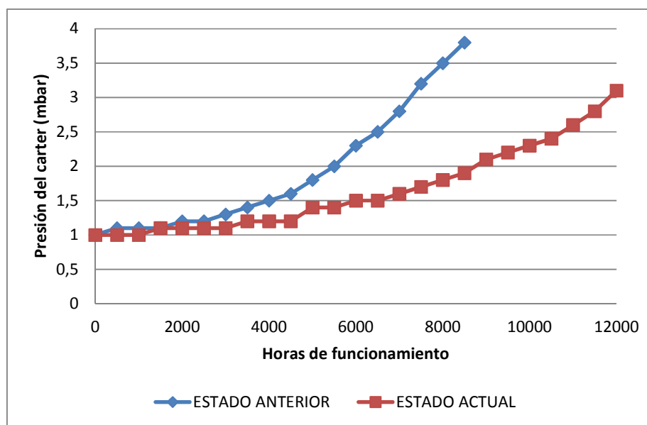
FIGURA 5.1 ESTADO ACTUAL MOTOR NÚMERO 6.
