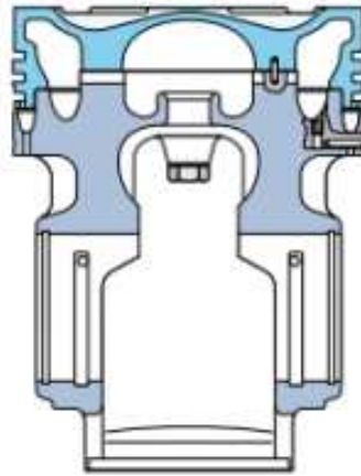
FIGURA 2.3 PISTÓN DEL MOTOR.
