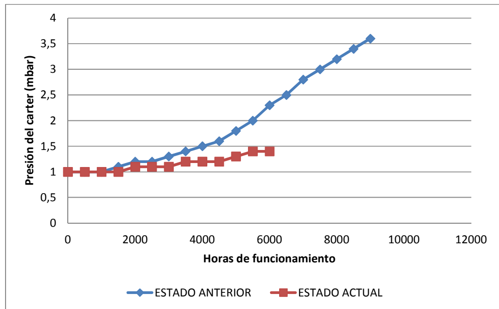
FIGURA 5.4 ESTADO ACTUAL MOTOR NÚMERO 2.
