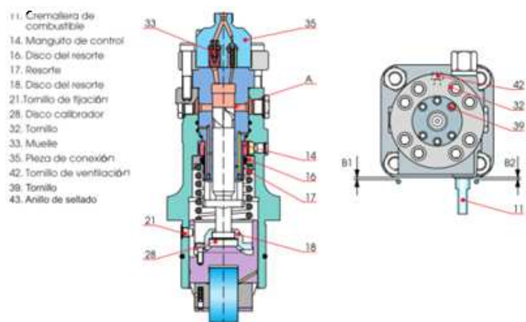
FIGURA 2.6 BOMBA DE INYECCIÓN.
