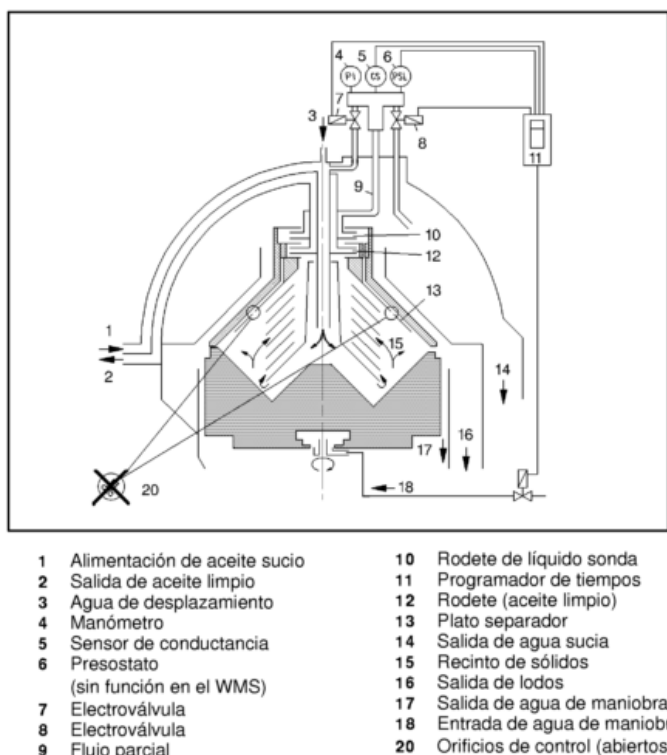
FIGURA 2.17 SISTEMA DE CONTROL DEL CONTENIDO DE AGUA (WMS) PARA TRATAMIENTO DEL COMBUSTIBLE.
