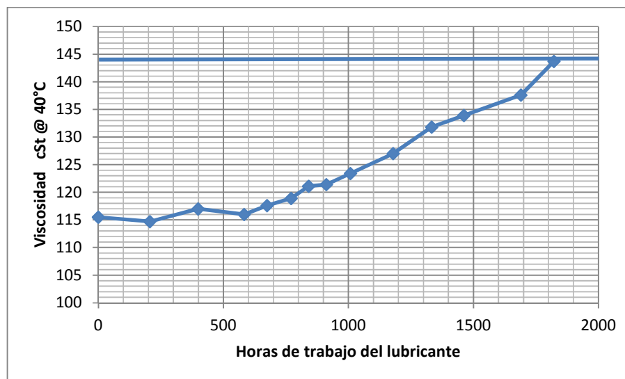
FIGURA 3.10 ANÁLISIS DE LA VISCOSIDAD DEL LUBRICANTE.
