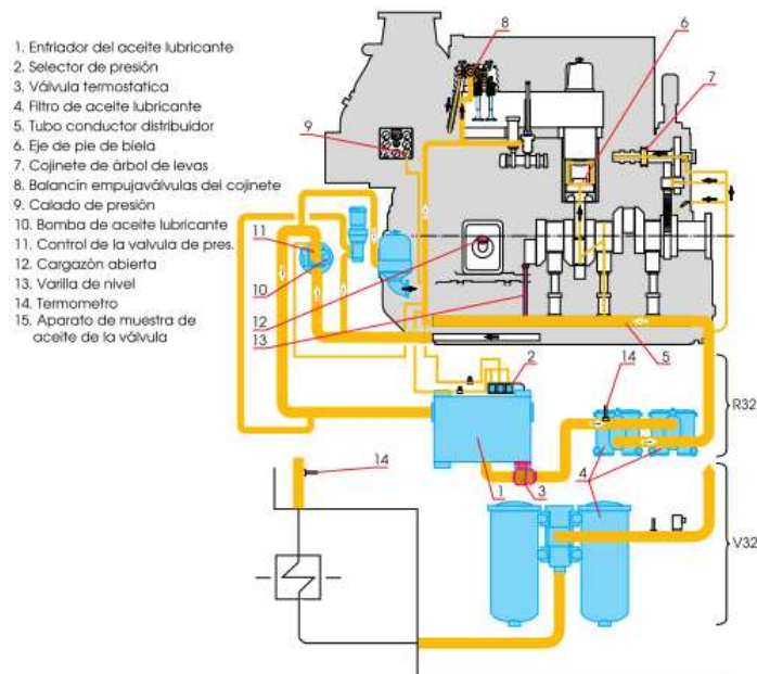
FIGURA 2.11 SISTEMA DE LUBRICACIÓN.
