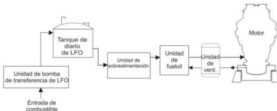
FIGURA 2.9 SISTEMA DE COMBUSTIBLE (LFO).
