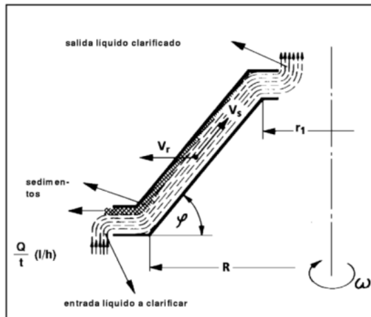
FIGURA 2.16 PRINCIPIO DE FUNCIONAMIENTO DE LA SEPARADORA CENTRÍFUGA.
