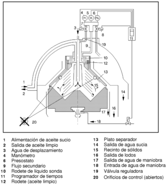
FIGURA 2.19 SISTEMA DE CONTROL DEL RECINTO DE LODOS (SMS) PARA TRATAMIENTO DEL ACEITE LUBRICANTE.
