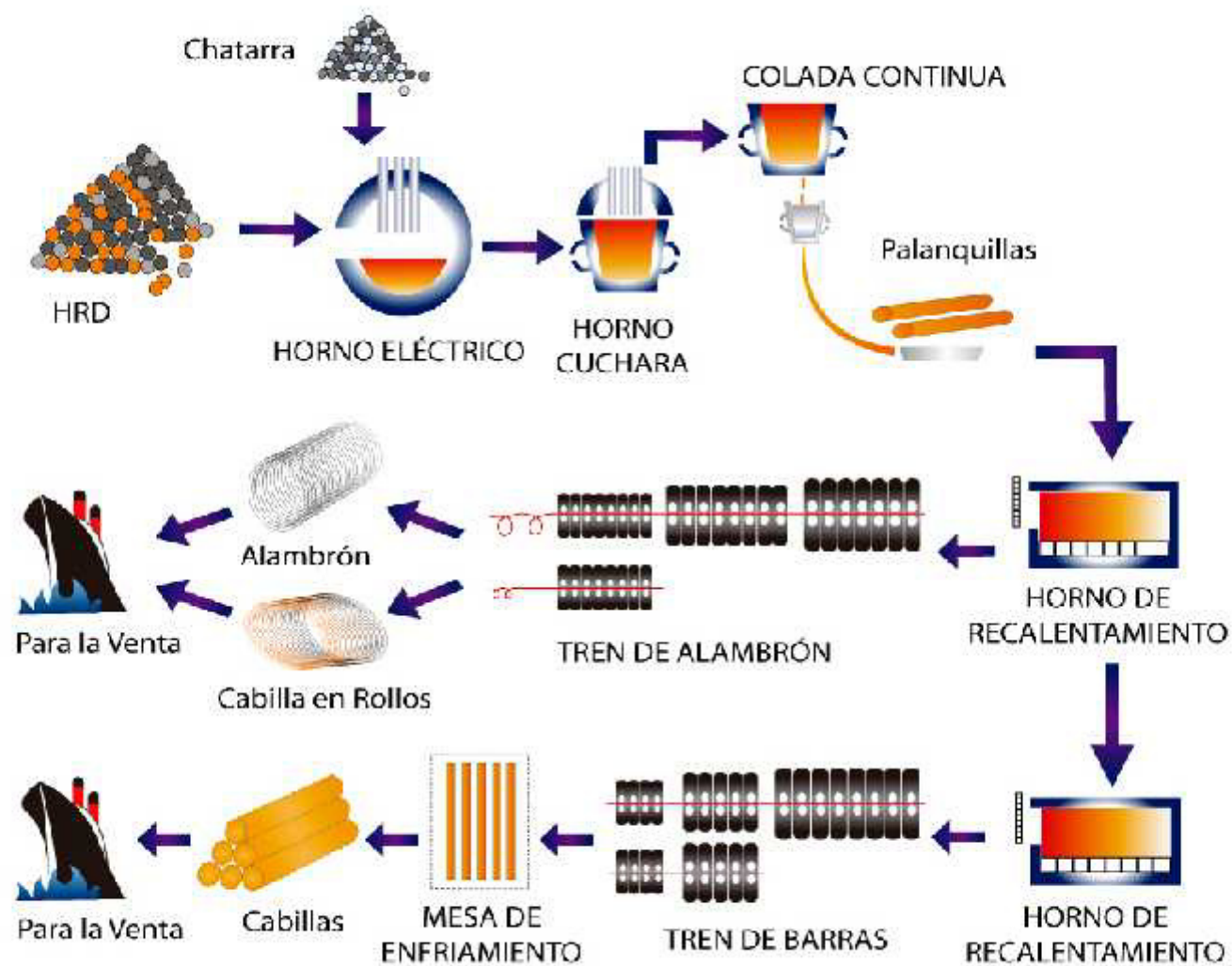
Figura 1: Procesos de Producción del Acero por Horno Eléctrico
