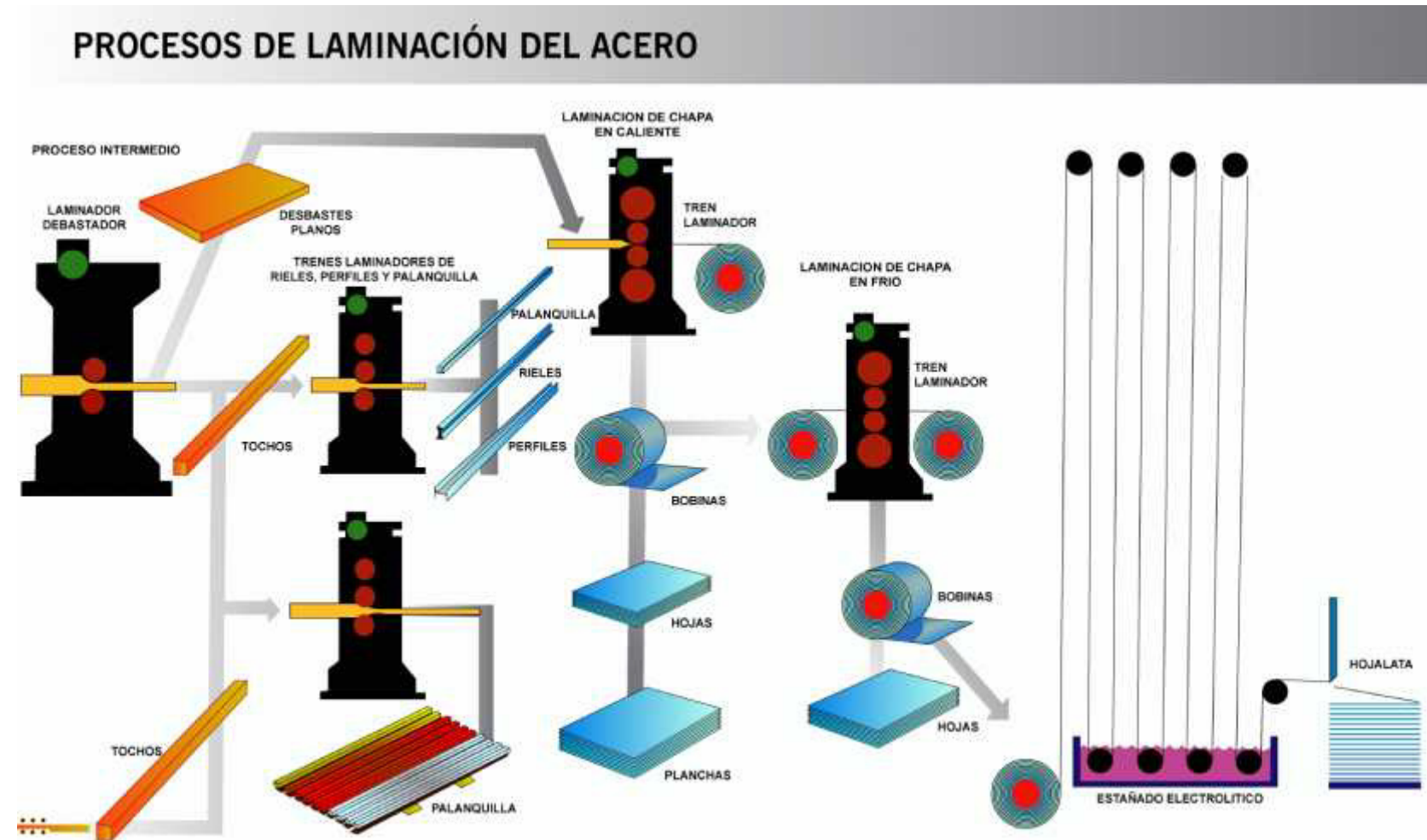
Figura 2: Proceso de Laminación del acero
