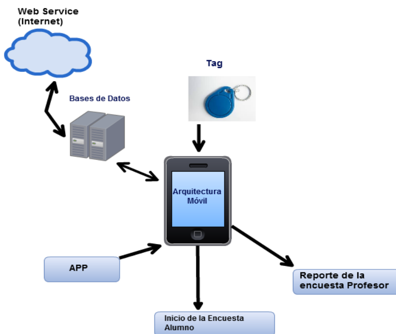
Figura 4.4. Arquitectura móvil
