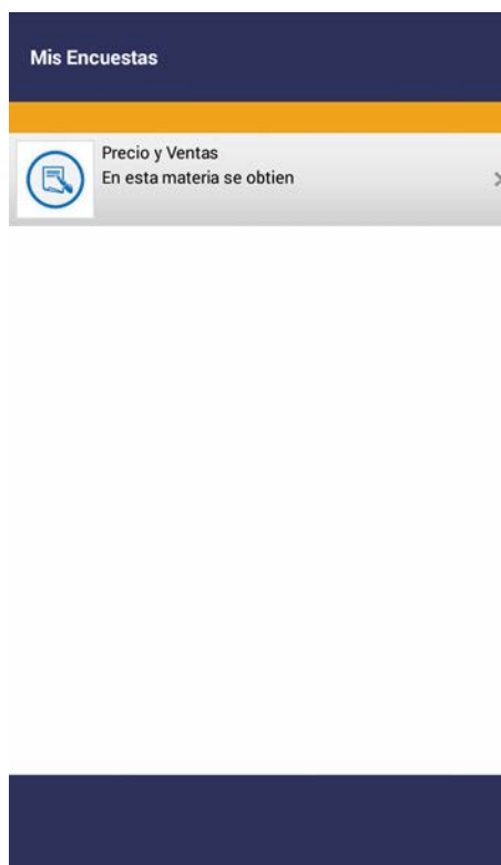
Figura 5.5. Realizar Encuesta
