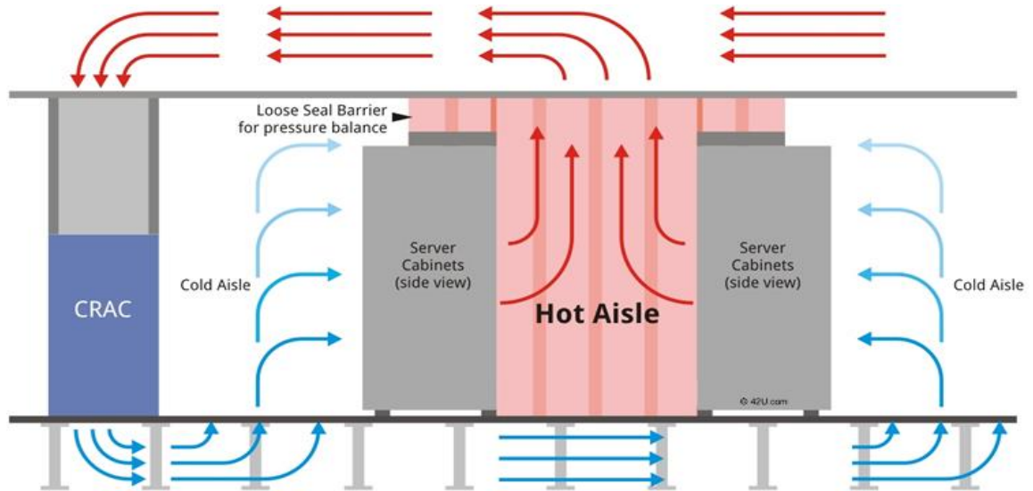
Figura 2.9. Problemas de Flujo de Aire
