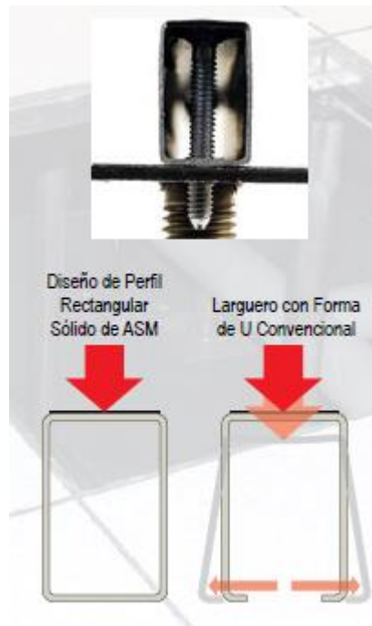
Figura 3.2. Larguero
