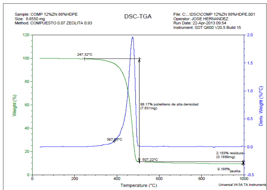
FIGURA A.7. TERMOGRAMA DE MEZCLA 12%ZE 88% HDPE
