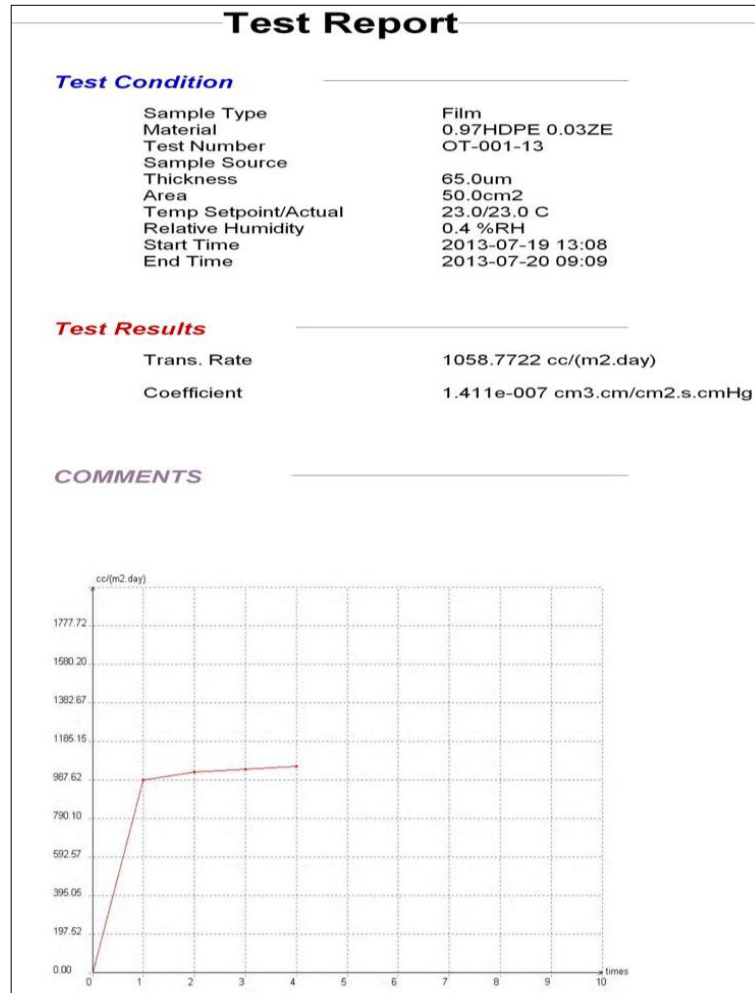
FIGURA F.9. IMAGEN DE LA MUESTRA CON 3% ZEOLITA NATURAL ECUATORIANA Y 97% POLIETILENO DE ALTA DENSIDAD (HDPE) EN OTR (CAMARA 1).
