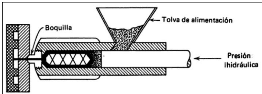
FIGURA 2.3 ESQUEMA DEL PROCESO DE MOLDEO POR INYECCIÓN [20].
