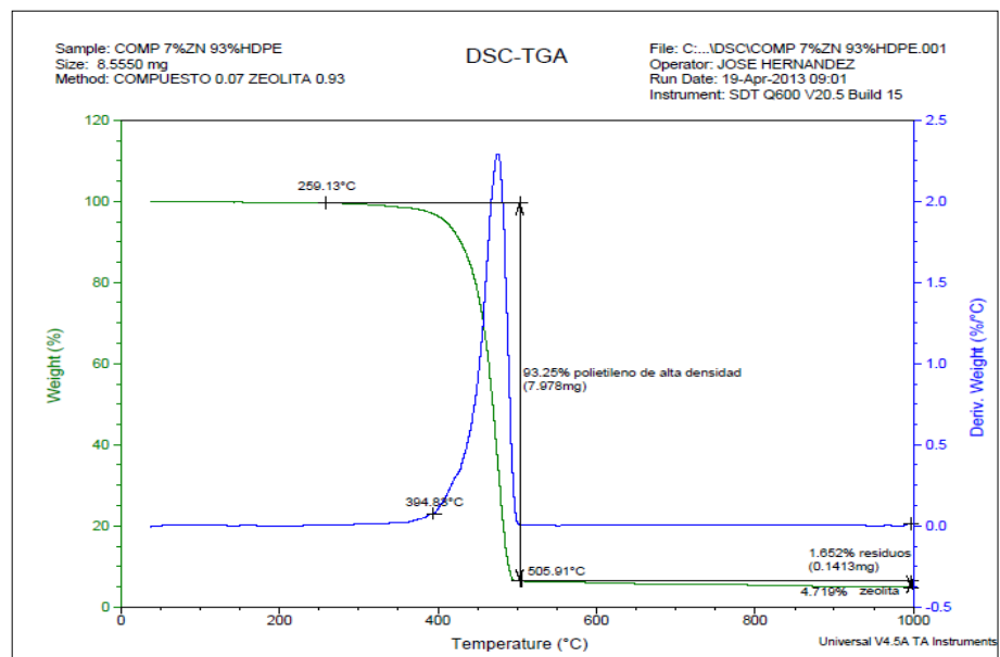
FIGURA A.5. TERMOGRAMA DE MEZCLA 7%ZE 93% HDPE
