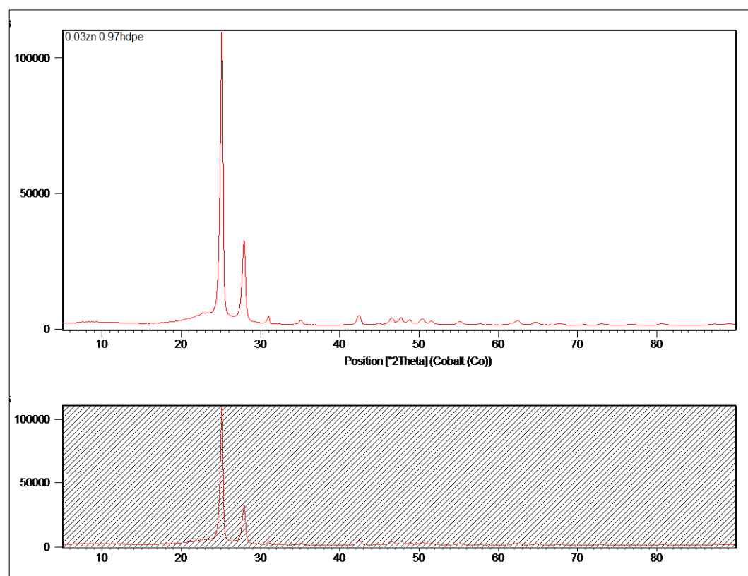
FIGURA E.7. DIFRACTOGRAMA DE 3%ZEO CON 97%HDPE.
