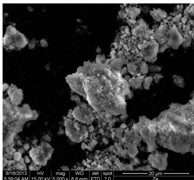
FIGURA D.10 IMAGEN DE LA MUESTRA CON ZEOLITA ECUATORIANA AMPLIFICADA A 5000X
