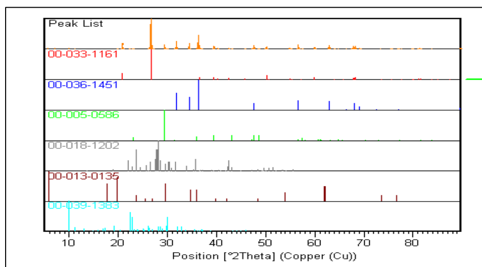
FIGURA E.5. DIFRACTOGRAMA DE ZEOLITA NATURAL
