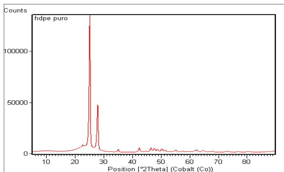
FIGURA E.6. DIFRACTOGRAMA DE HDPE PURO
