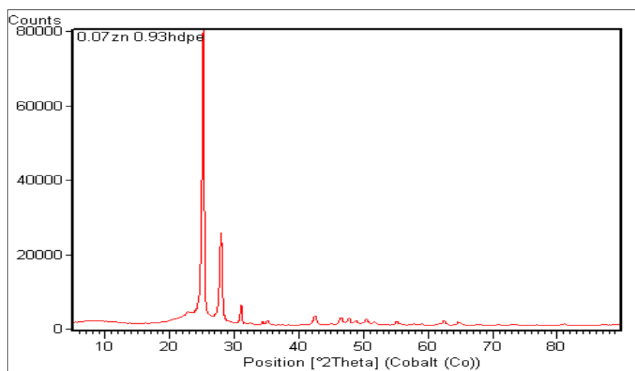
FIGURA E.9. DIFRACTOGRAMA 7%ZEO CON 93%HDPE.
