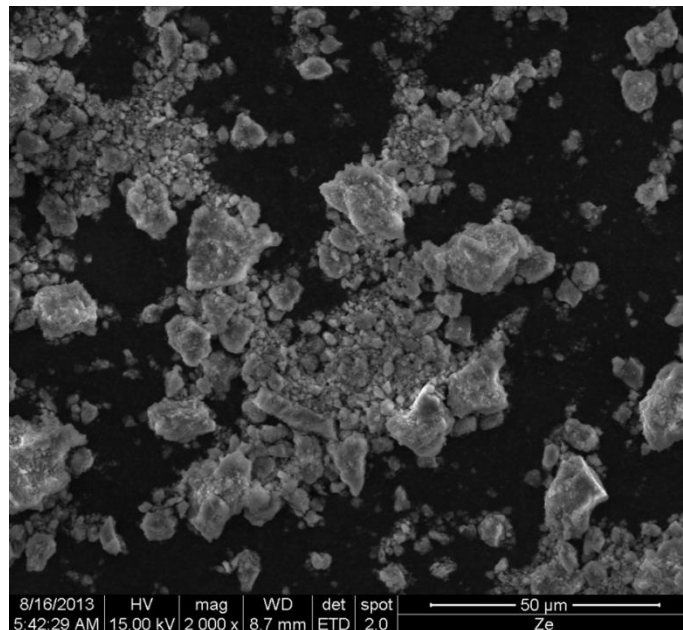
FIGURA D.8. IMAGEN DE LA MUESTRA CON ZEOLITA ECUATORIANA AMPLIFICADA A 2000X
