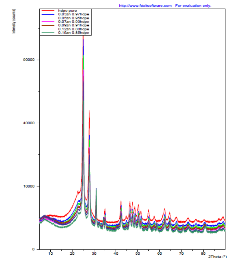
FIGURA E.3. SUPERPOSICIÓN DE DIFRACTOGRAMAS DE LAS MEZCLAS Y DEL POLIETILENO DE ALTA DENSIDAD
