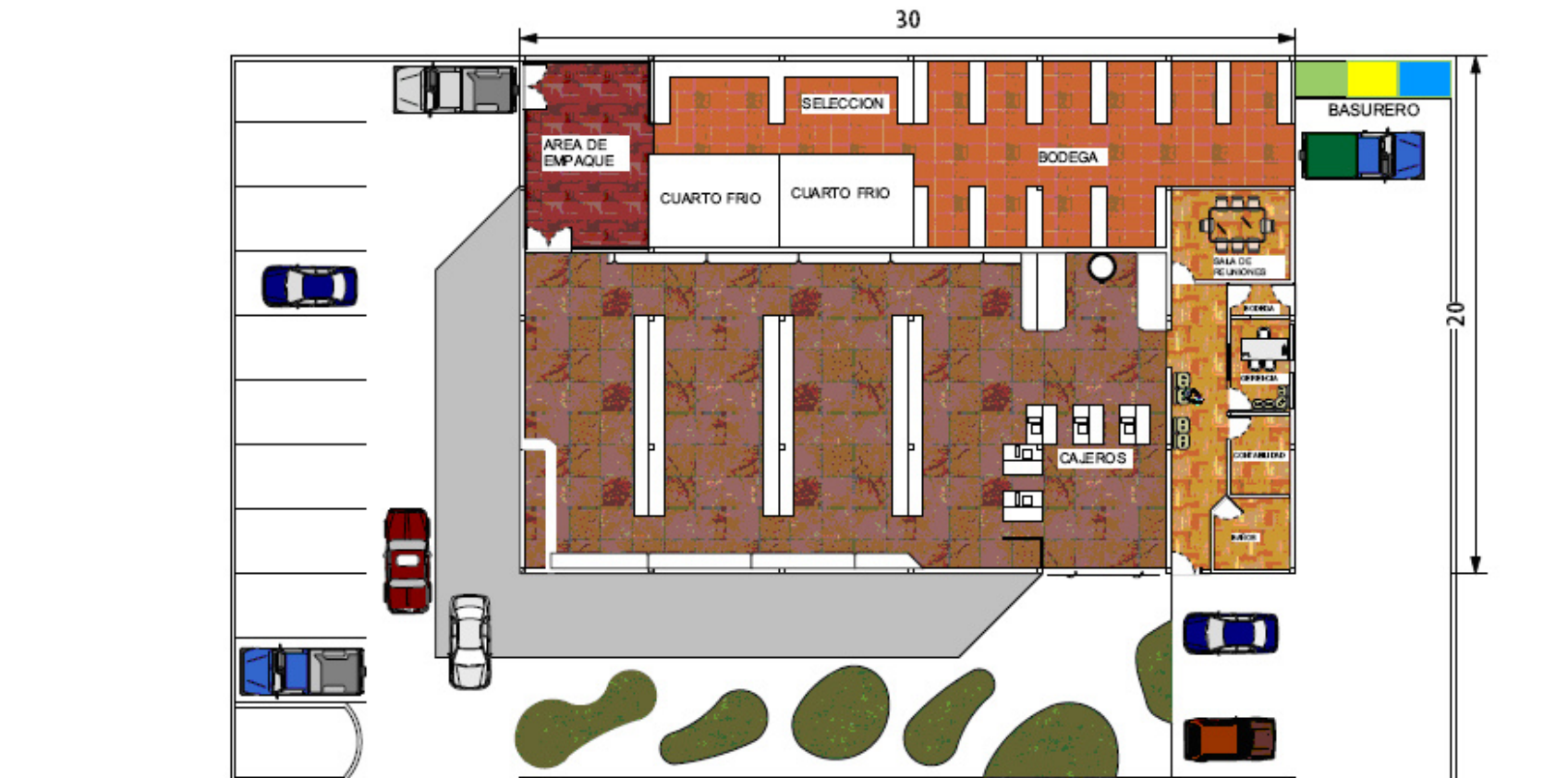
Grafico No. 15 Plano Arquitectónico
