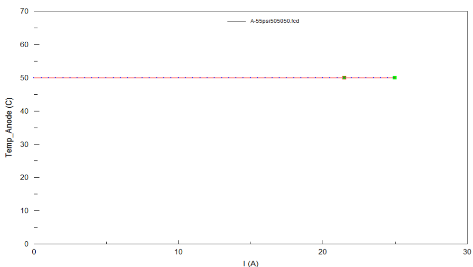
GRÁFICA 6.10. TEMPERATURA DEL HUMIDIFICADOR EN EL LADO DEL ÁNODO VS CORRIENTE DE LA CELDA PARA LA MEMBRANA A.
