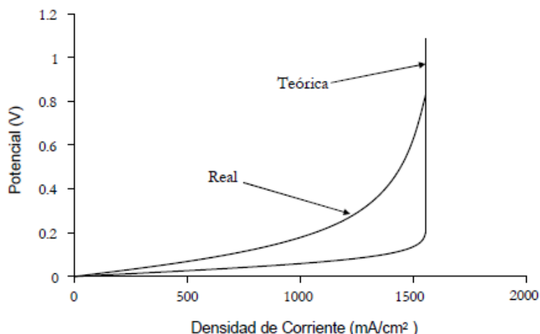
FIGURA 2.7. GRÁFICA DE POLARIZACIÓN POR CONCENTRACIÓN EN UNA CELDA DE COMBUSTIBLE PEM.
