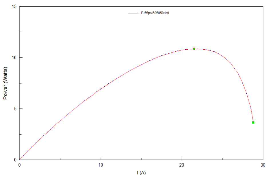
GRÁFICA 6.18. POTENCIAL DE LA CELDA DE COMBUSTIBLE VS CORRIENTE PARA LA MEMBRANA B
