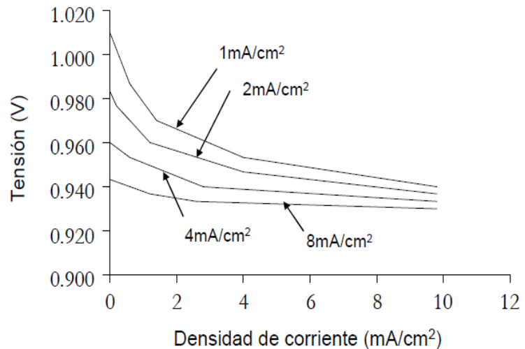
FIGURA 2.5. EFECTO DE LAS PÉRDIDAS POR CORRIENTE INTERNA Y EFECTO CROSSOVER
