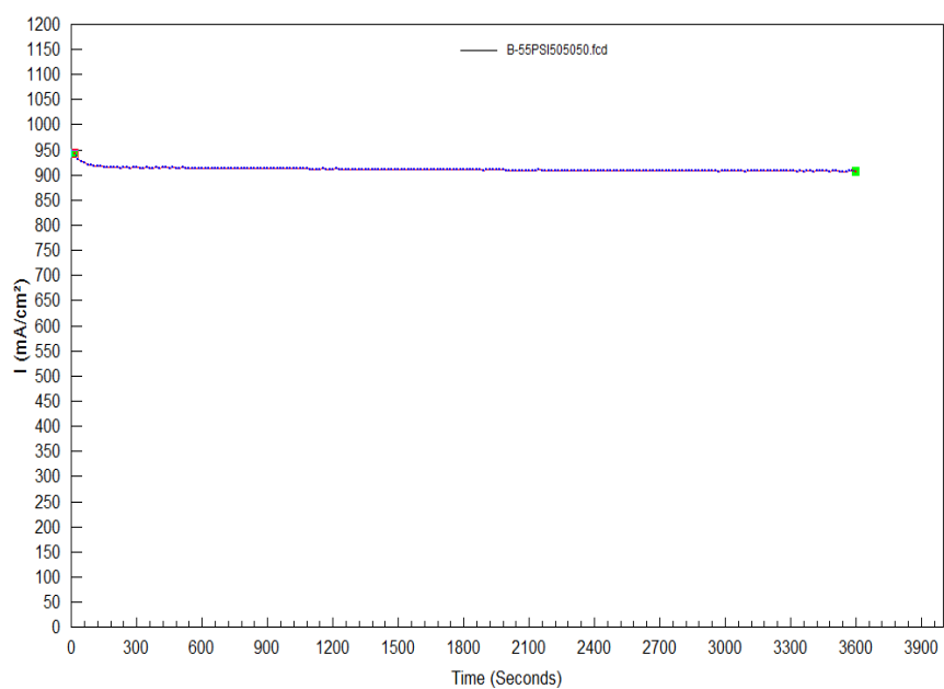
GRÁFICA 6.15. DENSIDAD DE CORRIENTE VS TIEMPO MEMBRANA B
