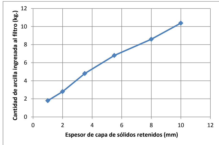
GRÁFICO 4.2 ESPESOR DE CAPA DE SÓLIDOS RETENIDOS VS. CANTIDAD DE ARCILLA INGRESADA AL FILTRO.
