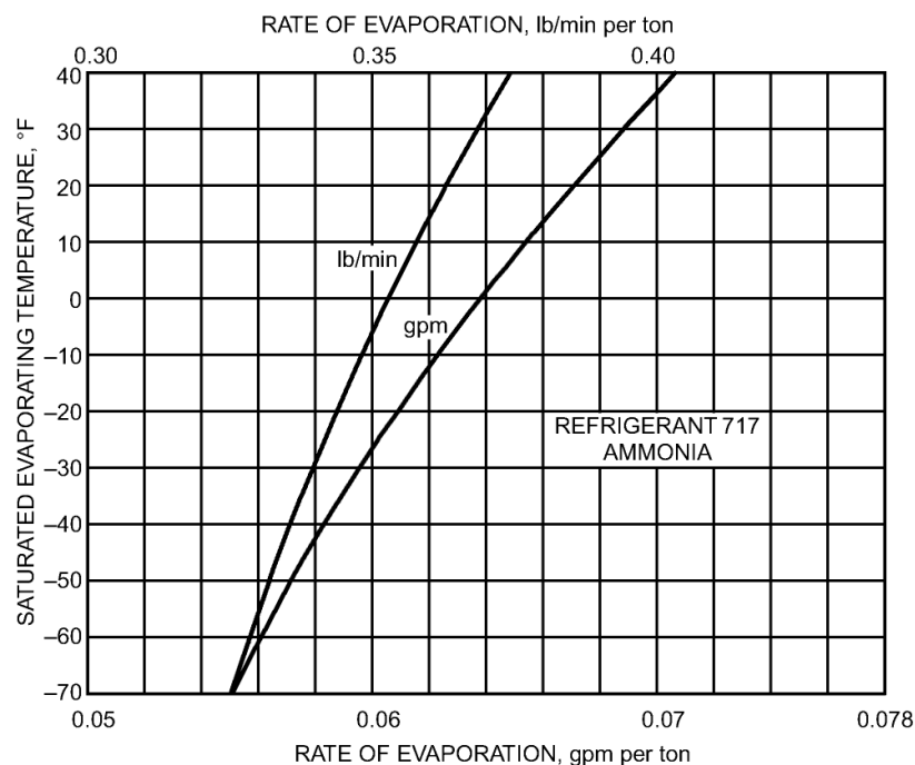
FIGURA 4.3. RELACIÓN ENTRE LA TASA DE EVAPORACIÓN Y TEMPERATURA DE EVAPORACIÓN,
