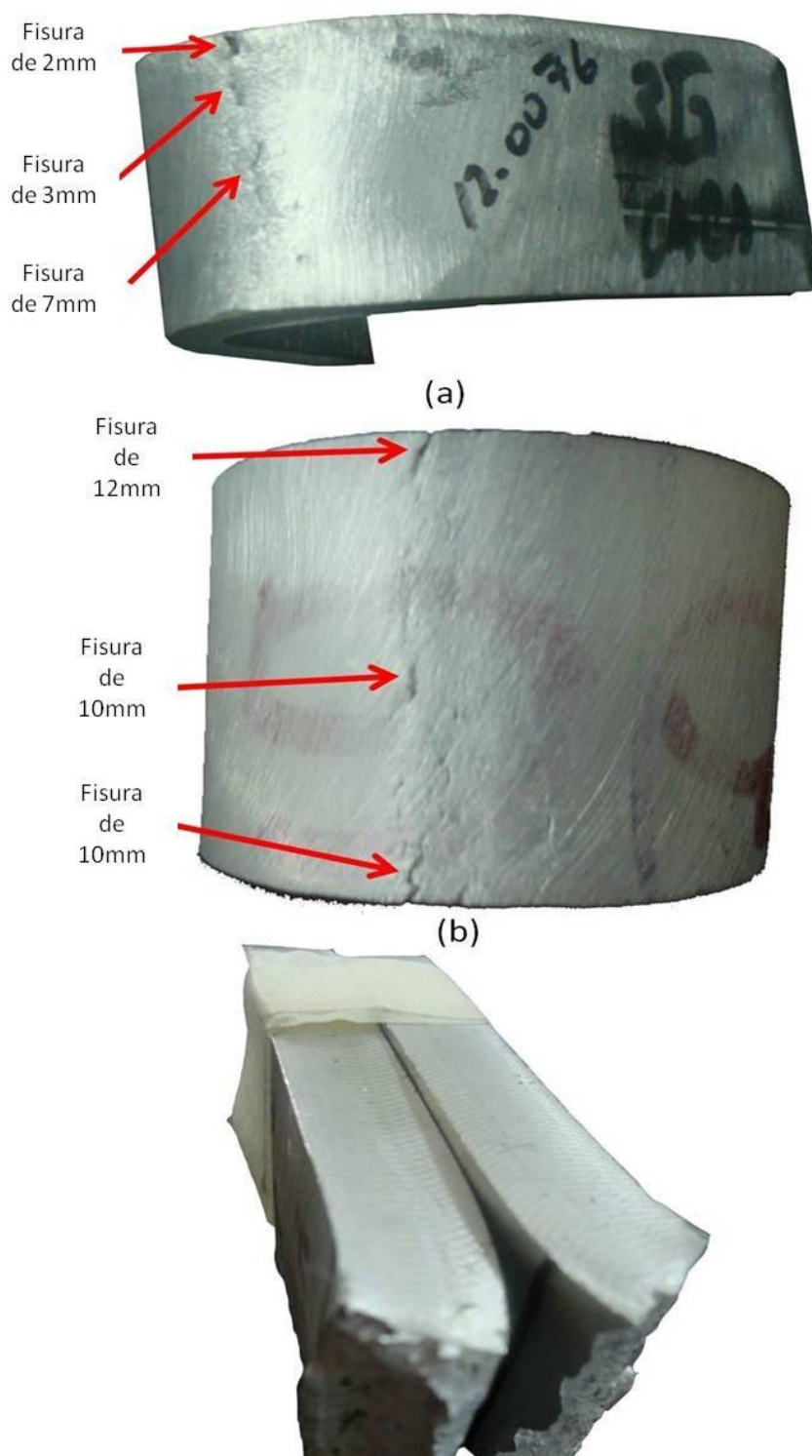
Figura 2. 33.- Especímenes con fisuras excesivas de: 12mm (a), 11mm (b) y fractura
