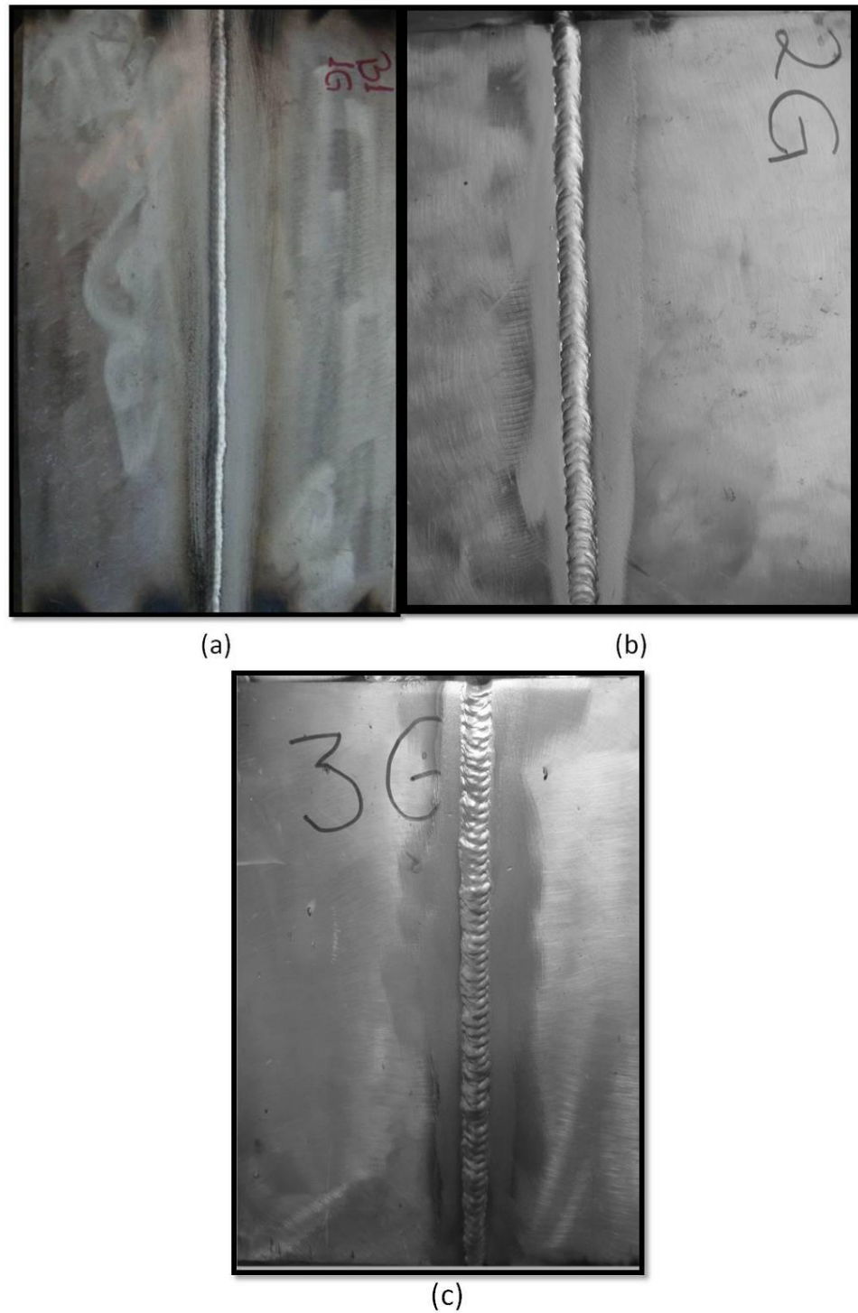
Figura 2. 12.- Probetas calificadas para las distintas posiciones en 6mm: 1G (a), 2G (b), y 3G (c)
