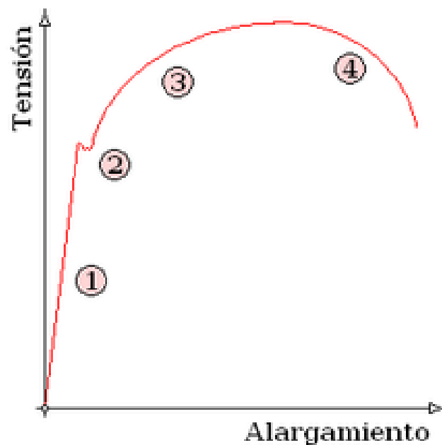
Figura 1. 7.- Curva tensión-alargamiento
