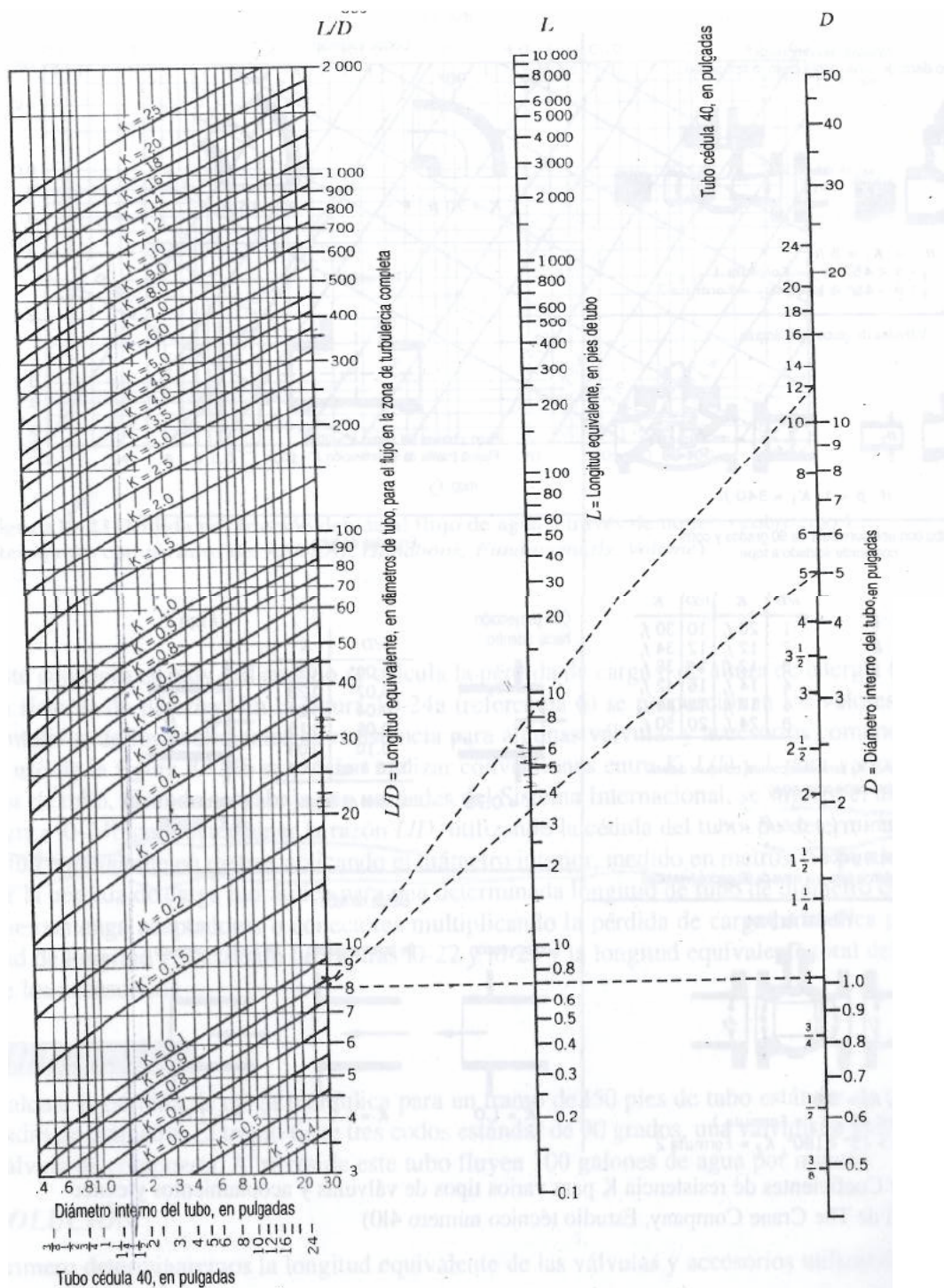
FIGURA 3.3 LONGITUDES EQUIVALENTES L Y L/D , COEFICIENTE DE RESISTENCIA K
