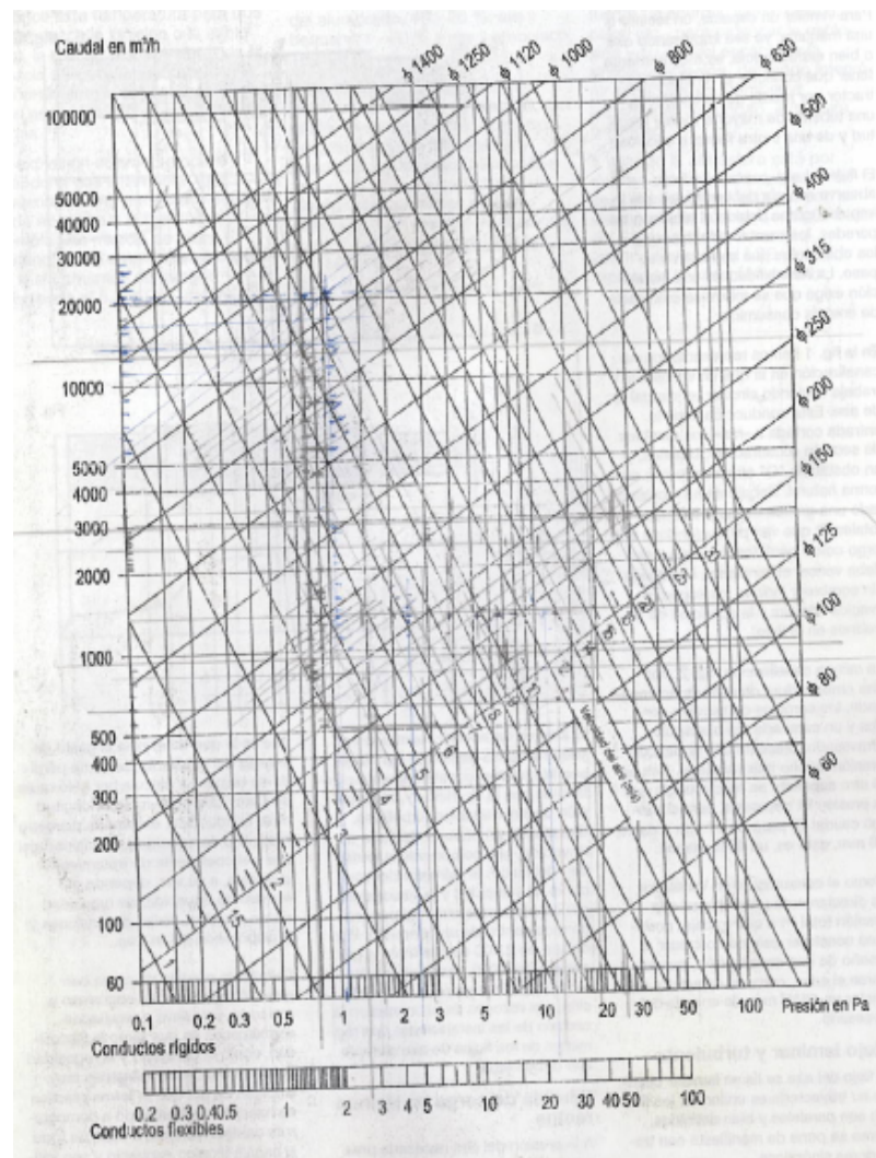
FIGURA 2.1 DIAGRAMA CAUDAL & PRESIÓN
