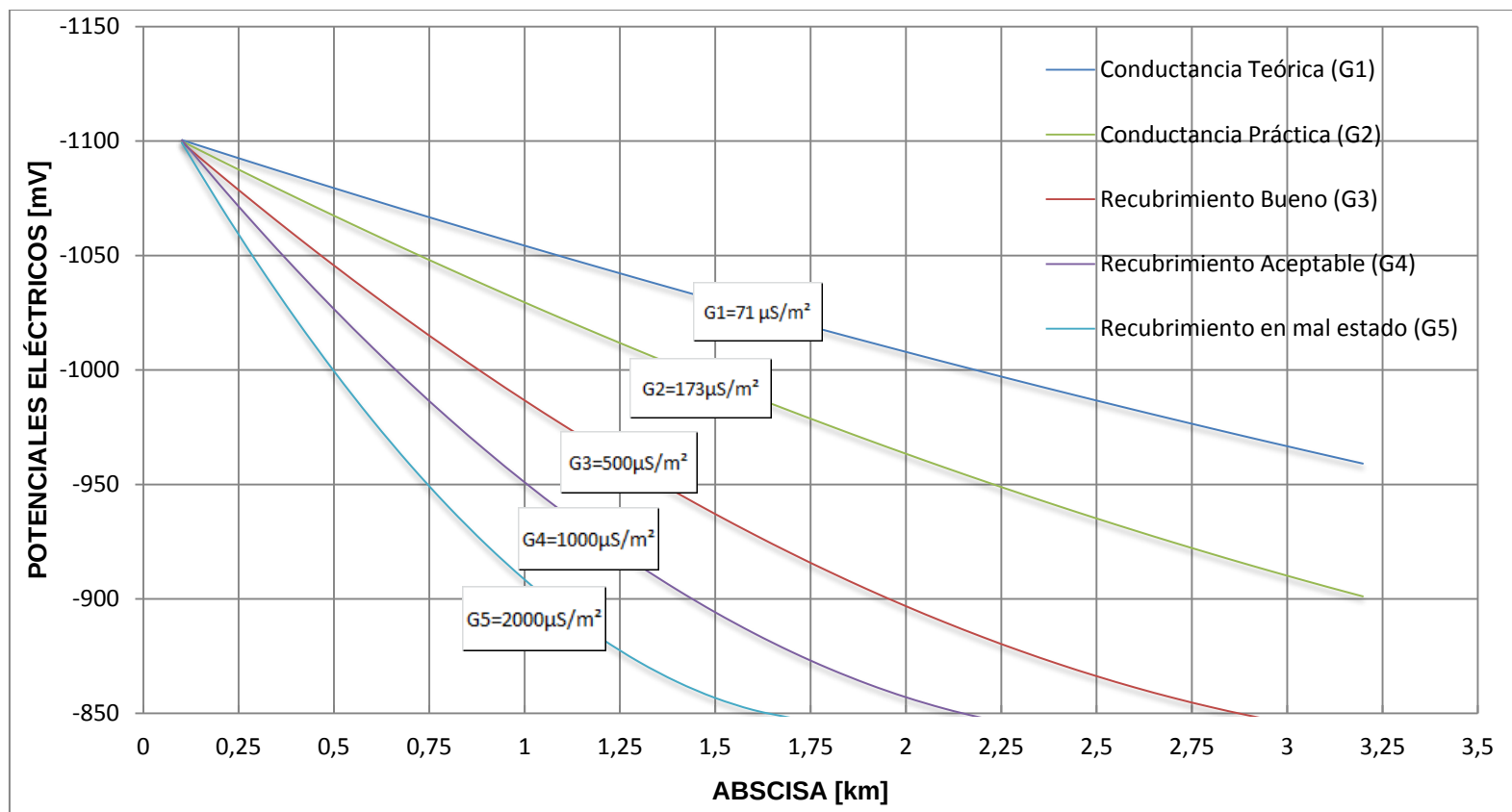
FIG. 3.8. DISTRIBUCIÓN DE POTENCIALES ELÉCTRICOS EN FUNCIÓN DE LA CALIDAD DEL RECUBRIMIENTO
