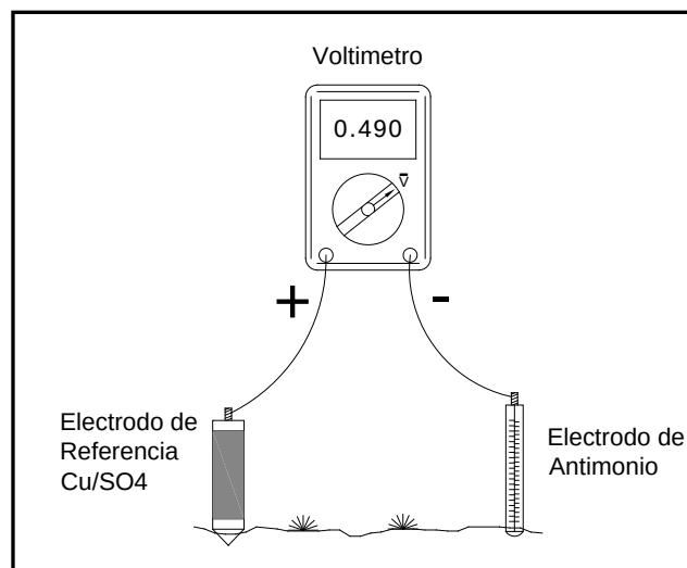
ESQUEMA DE EQUIPOS DE MEDICIÓN DE pH
