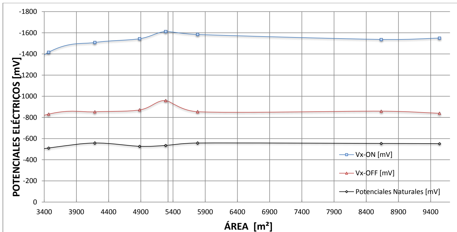
FIG. 3.4. DISTRIBUCIÓN DE POTENCIALES EN PRUEBA DE CONDUCTANCIA ELÉCTRICA DEL RECUBRIMIENTO EN FUNCIÓN DEL ÁREA SUPERFICIAL
