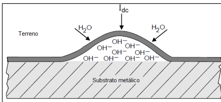
FIG. 1.9. AMPOLLAMIENTO DEL RECUBRIMIENTO
