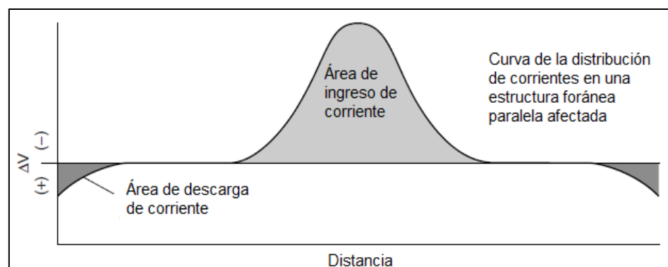
FIG. 1.10. VARIACIÓN DE VOLTAJE EN ZONAS DE INGRESO Y SALIDA DE CORRIENTE
