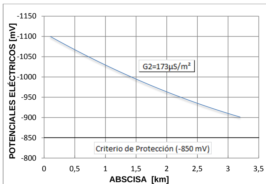
FIG. 3.6. DISTRIBUCIÓN ACTUAL DE POTENCIALES ELÉCTRICOS EN ACUEDUCTO
