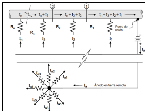
FIG. 1.4. RESISTENCIAS EN LA DISTRIBUCIÓN IDEAL DE CORRIENTES EN UN SPC
