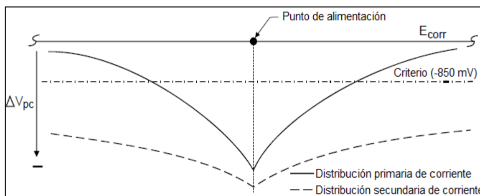
FIG.1.7. EFECTOS DEL TIEMPO DE POLARIZACIÓN EN EL PERFIL DE ATENUACIÓN DE LA ESTRUCTURA
