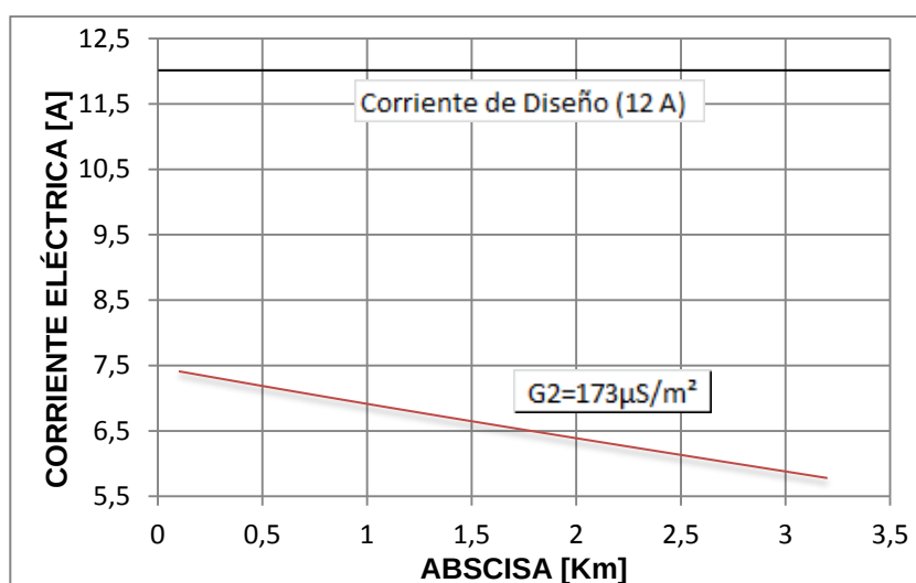
FIG. 3.7. DISTRIBUCIÓN ACTUAL DE CORRIENTE EN EL ACUEDUCTO
