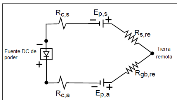
FIG. 2.8. CIRCUITO DEL SISTEMA DE PROTECCIÓN CATÓDICA PARA TUBERÍAS ENTERRADAS
