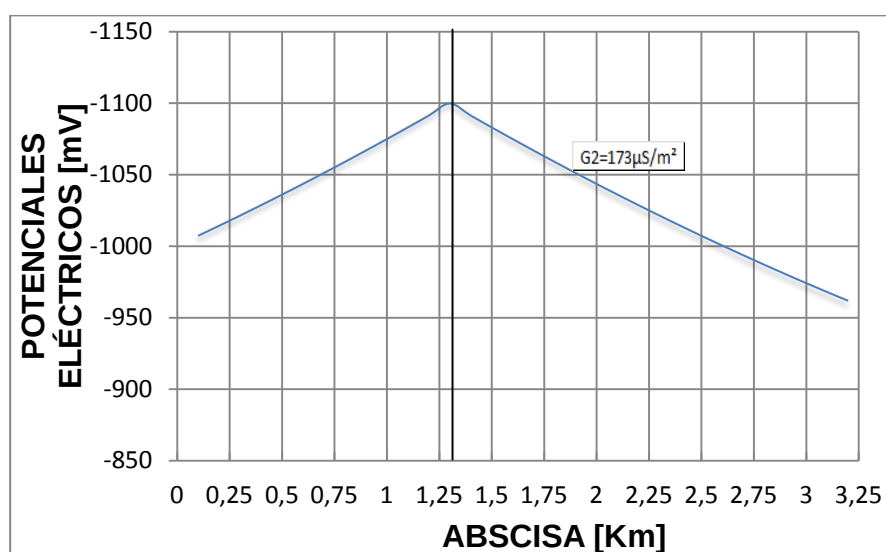
FIG. 3.11. DISTRIBUCIÓN DE POTENCIALES ELÉCTRICOS CON ALIMENTACIÓN EN ABSCISA SELECCIONADA
