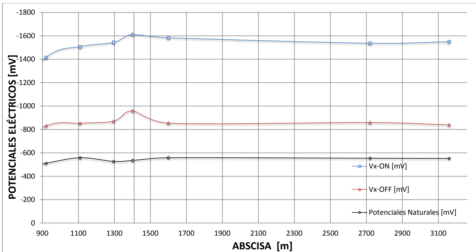
FIG. 3.3. DISTRIBUCIÓN DE POTENCIALES EN PRUEBA DE CONDUCTANCIA ELÉCTRICA DEL RECUBRIMIENTO
