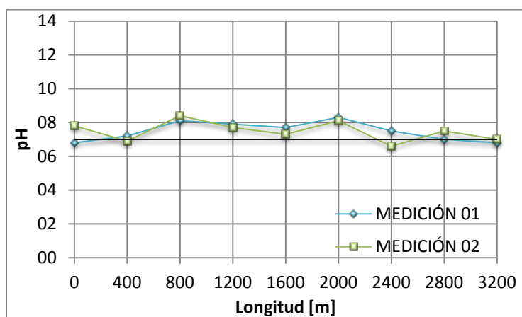
FIG. 2.4. NIVEL DE pH DEL SUELO
