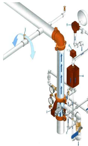
FIGURA 4.3 – SISTEMA DE ROCIADORES
