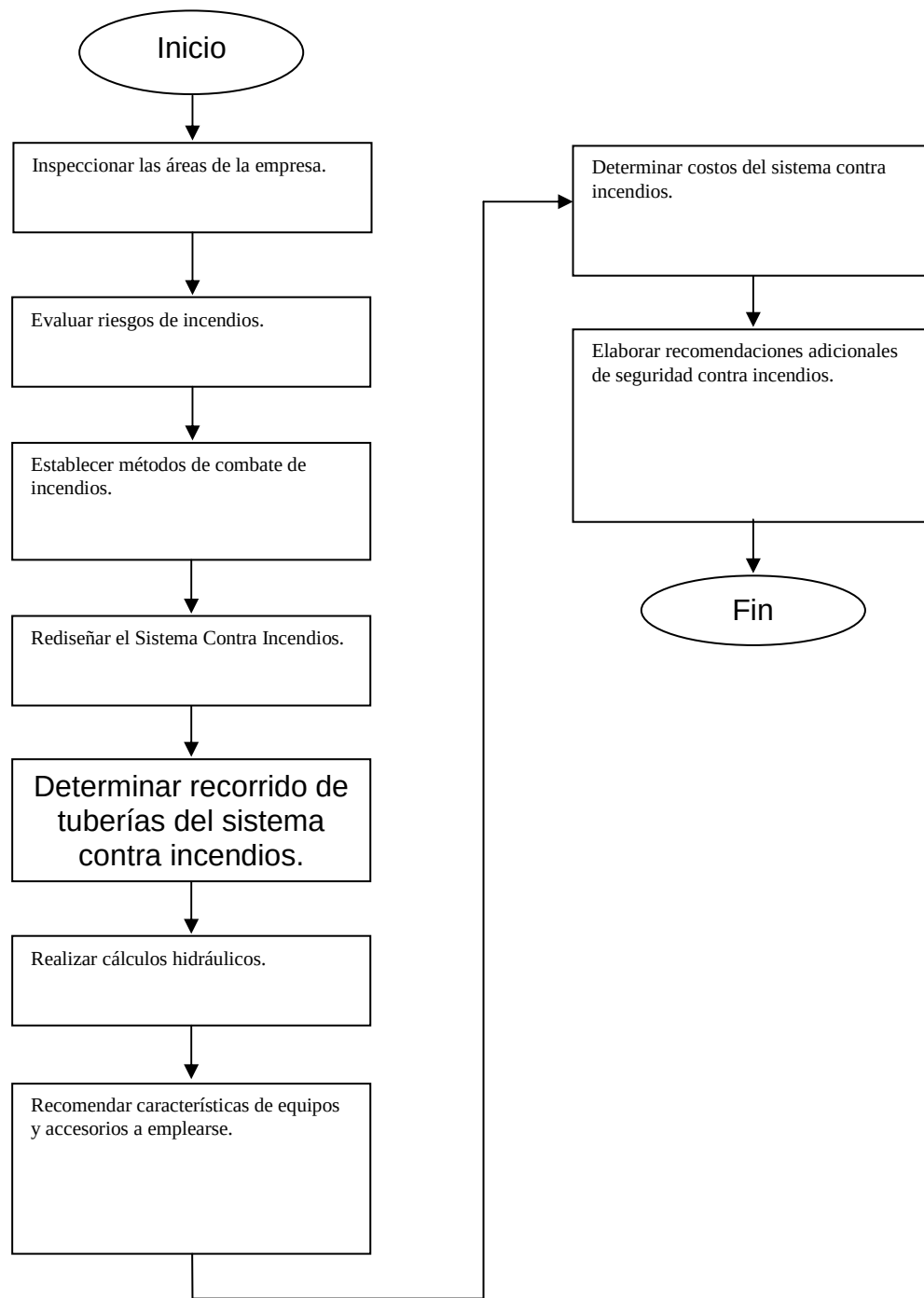
FIGURA 1.1 – METODOLOGÍA UTILIZADA EN EL PRESENTE TRABAJO
