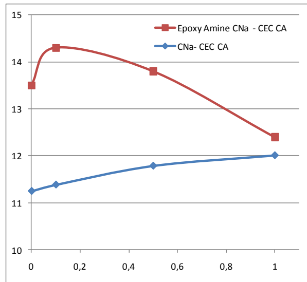
FIGURA 4.2 COMPARACIÓN DEL D-SPACING DE CNa CON EL CEC- CA Y SISTEMAS EPOXY AMINE.
