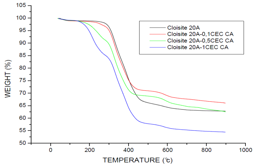
FIGURA 4.19 CURVAS DE DESCOMPOSICIÓN TÉRMICA DE TODAS LAS CLOISITE 20A Y CA
