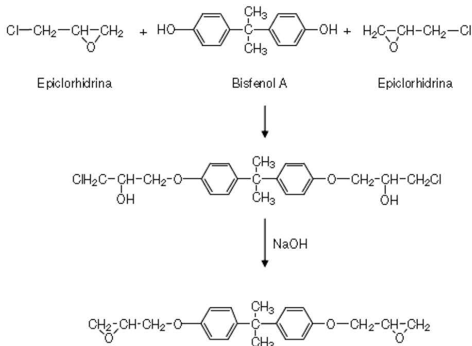
FIGURA 2.2 REACCIÓN ENTRE EL BISFENOL A Y LA EPICLORHIDRINA PARA FORMAR UNA RESINA EPÓXICA (9).
