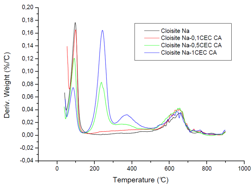
FIGURA 4.16 DERIVADAS DE LAS CURVAS DE DESCOMPOSICIÓN TÉRMICA DE TODAS LAS CLOISITE Na Y CA
