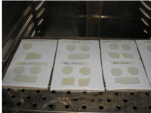
FIGURA 3.19 NANOCOMPUESTOS FABRICADOS.
