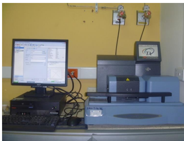
FIGURA 3.21 EQUIPO TÉRMICO GRAVIMÉTRICO.
