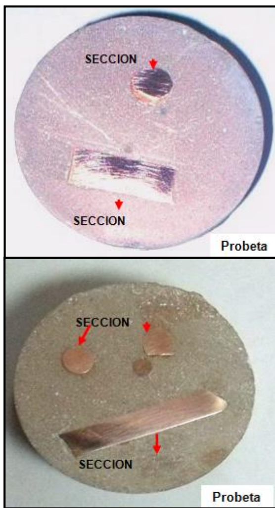
Figura 1.21. Probetas sin pulir.
