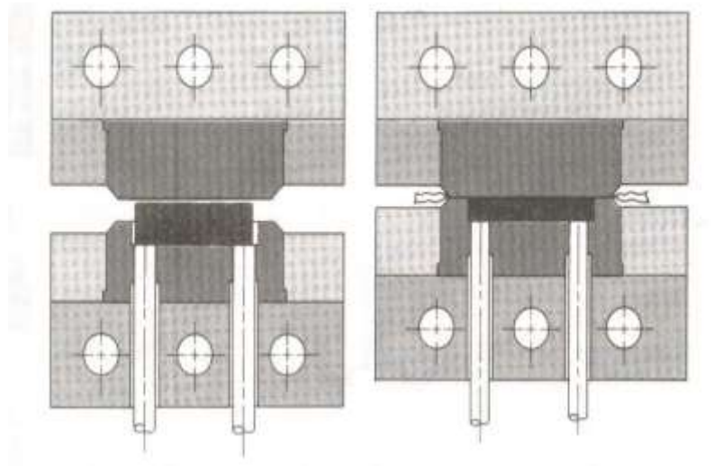
FIGURA 2.9. REPRESENTACIÓN ESQUEMÁTICA DE MOLDEO POR COMPRESIÓN
