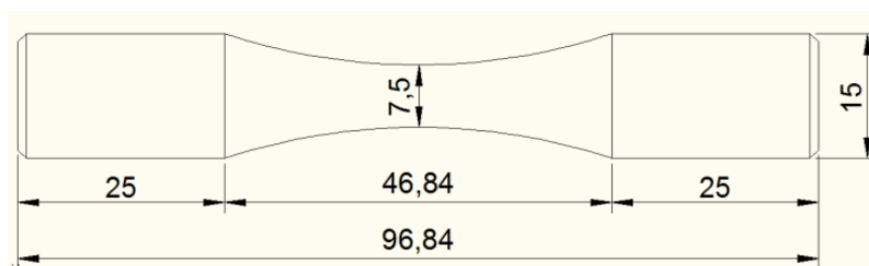
FIG. 1.12 DIMENSIONES DE LA PROBETA ESTANDARIZADA
