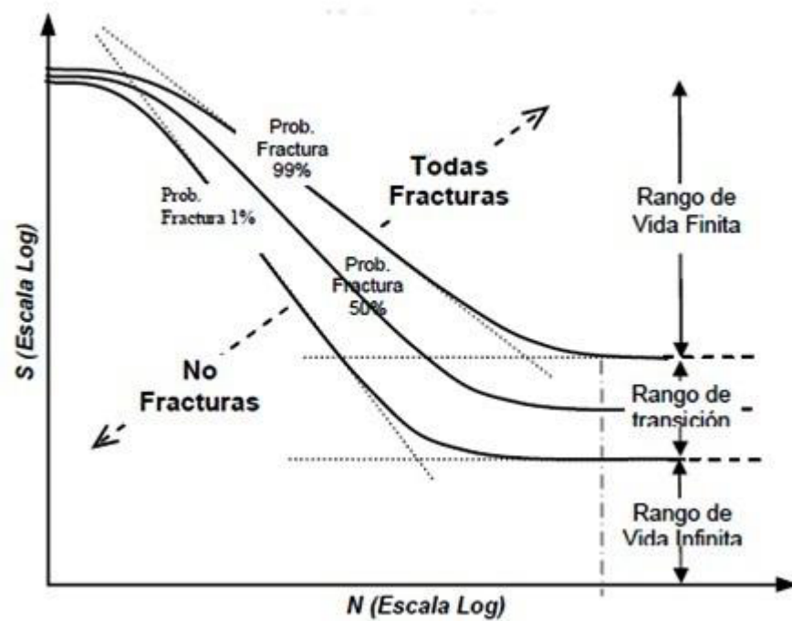
FIG. 1.15 CURVAS S-N-P [11].
