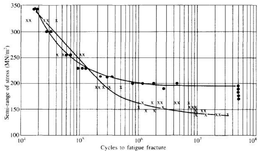
FIG. 1.5 CURVAS S-N PARA ALEACIONES FÉRREAS Y NO FÉRREAS [4]
