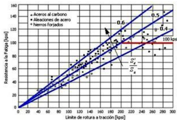
FIG. 1.7 LÍMITES DE RESISTENCIA A LA FATIGA [3]
