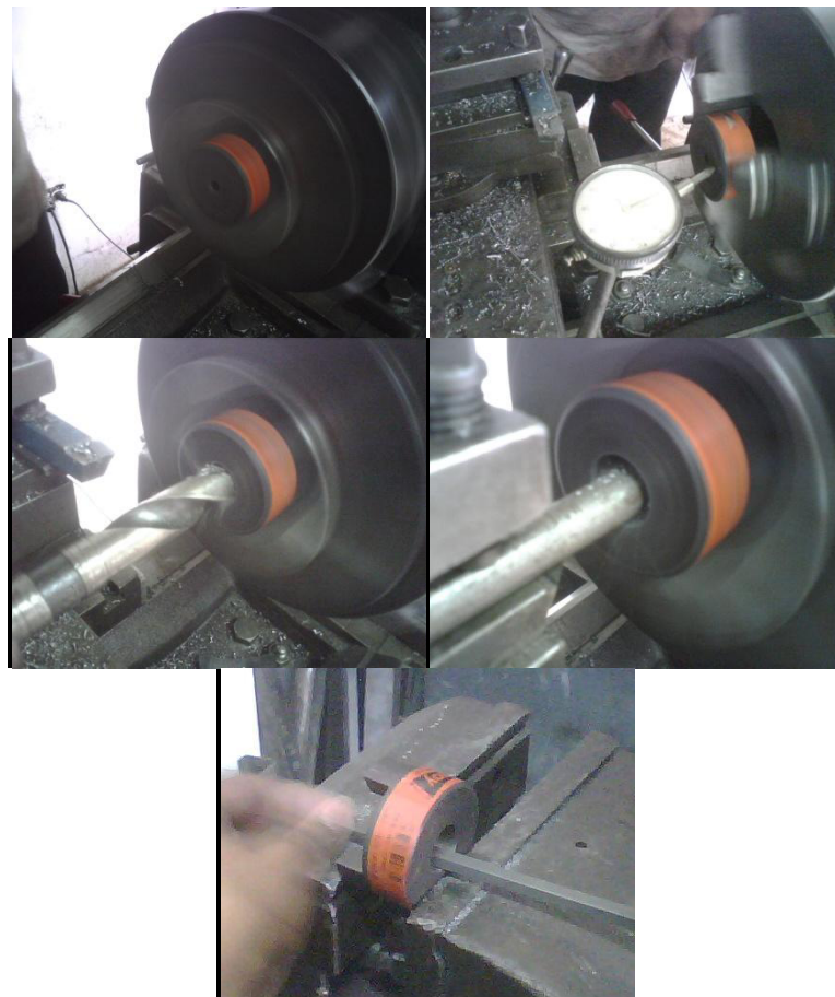
FIG. 2.5 PROCESO DE MECANIZADO DEL ACOUPLE SEMIFLEXIBLE
