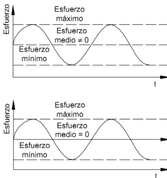
FIG. 1.3 TIPOS DE ESFUERZOS FLUCTUANTES
