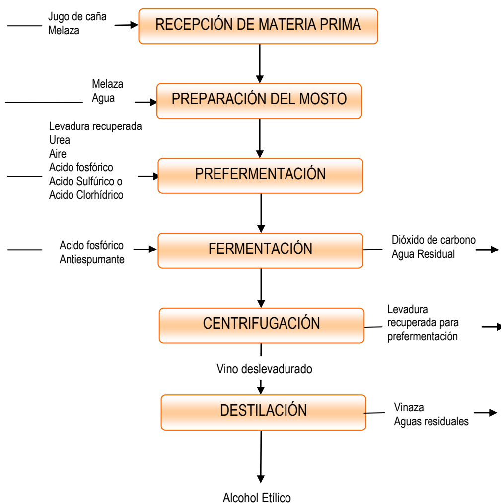
Figura 1.5 Diagrama de flujo del proceso
