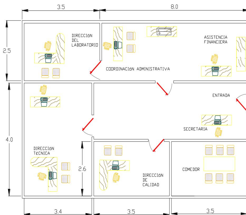
FIGURA 3.7 DIAGRAMA DE LAS OFICINAS DEL LABORATORIO-ADMINISTRATIVO.
