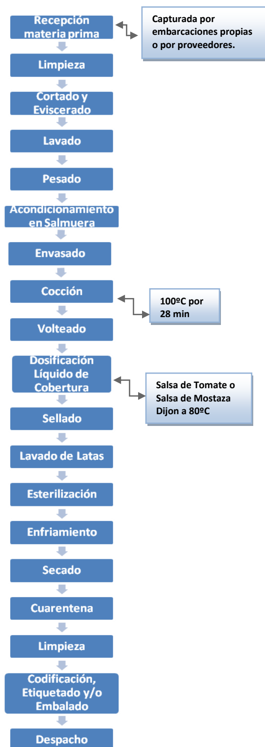
Figura 2.2 Diagrama Flujo Sardinas en Salsa Tomate Elaborado por: Fabián Vera, 2010.
