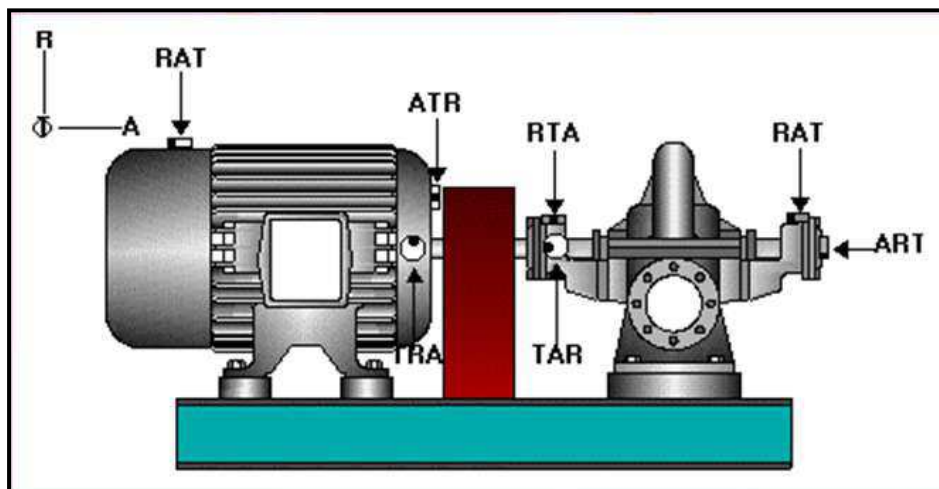
Figura 3.21 Ejes de medición
