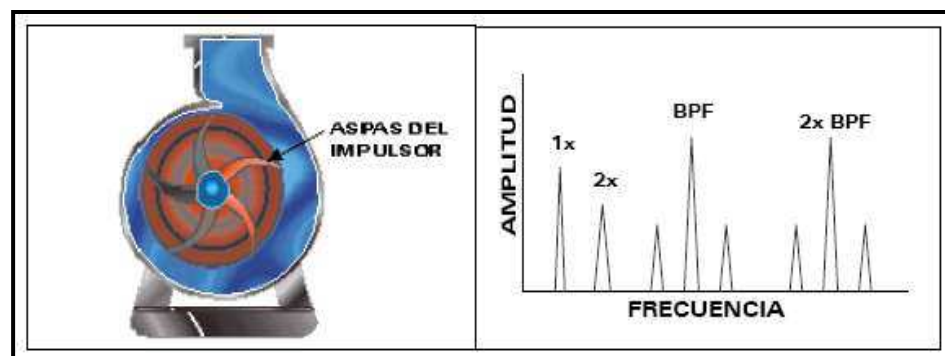
Figura 4.17 Frecuencia de aspas
