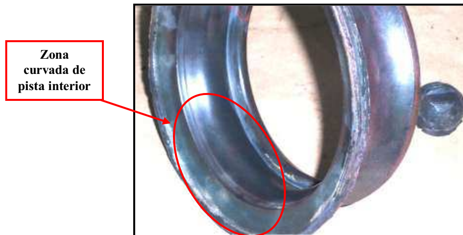
Figura 4.7 Pista interior curvada del rodamiento
