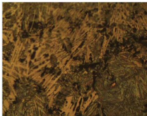
Figura 2.34 ZAT 500X producto B-1 Figura 2.35 ZAT 500X producto B-2
