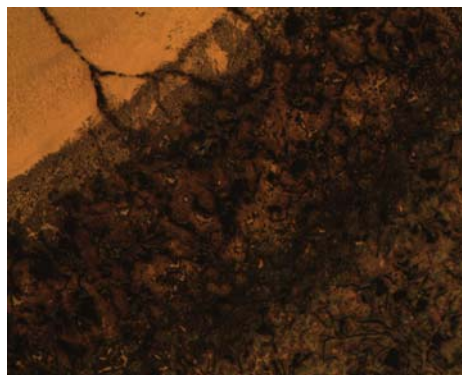
Figura 2.24 ZAT 50X producto A-1
