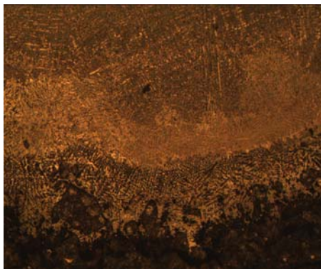
Figura 2.11 ZF 100X Producto A-1
