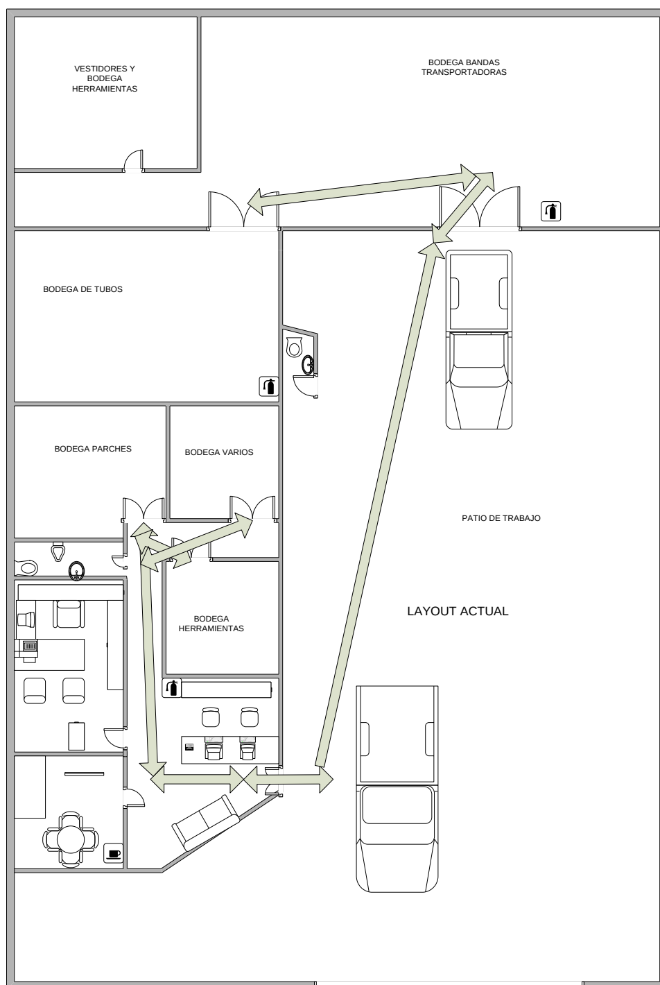
FIGURA 3.2. LAYOUT ACTUAL
