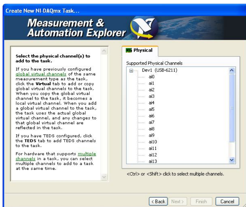
Figura 1.10 Measurement & Automation Explorer, Canales Físicos
