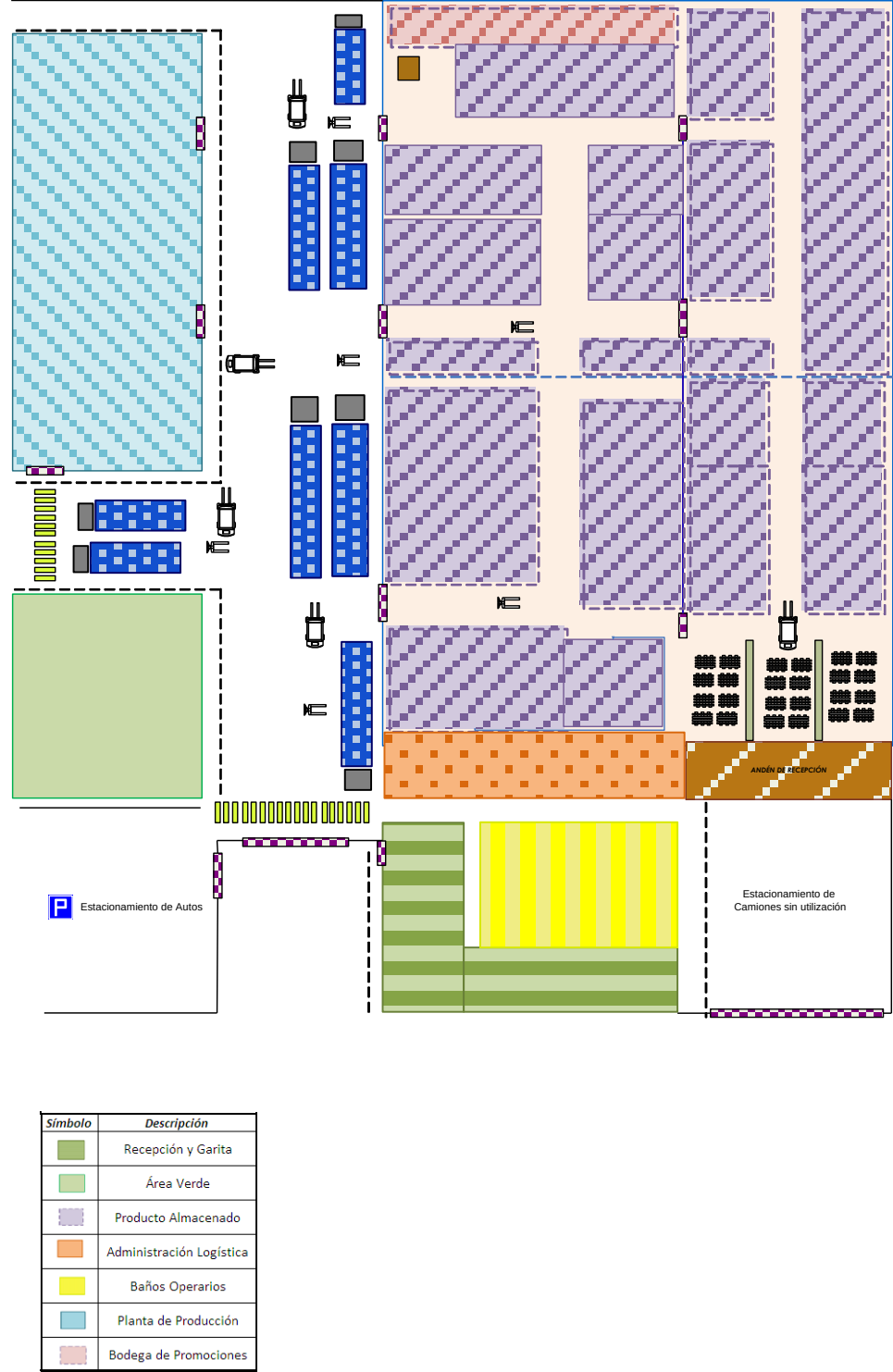
FIGURA 3.11 BOSQUEJO DE BPT CENTRAL ACTUAL
