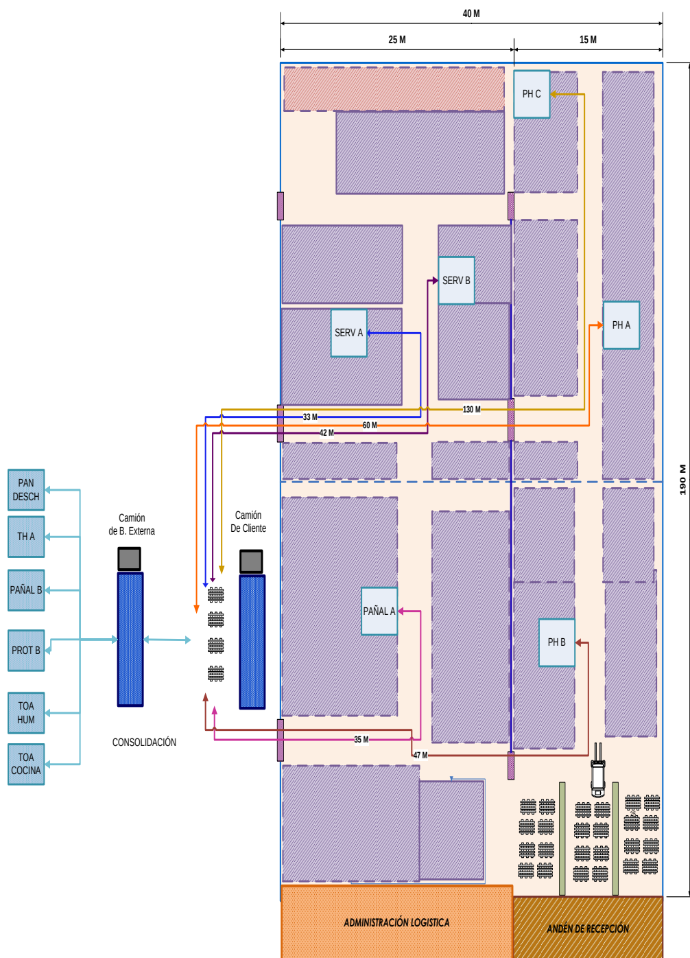
FIGURA 3.9 DIBUJO DE POSICIÓN DE ÍTEMS DEL PEDIDO CON APROXIMACIÓN DE DISTANCIAS
