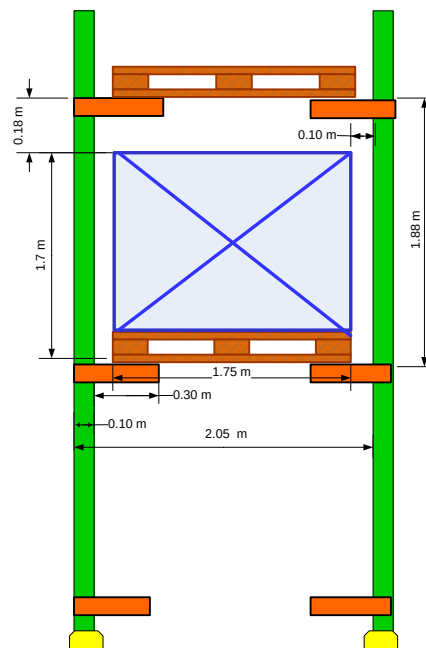
FIGURA 4.2 ESTANTERÍA CON DIMENSIONES
