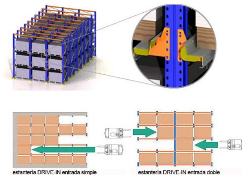
FIGURA 2.4 ESTANTERÍA COMPACTA O DRIVE IN
