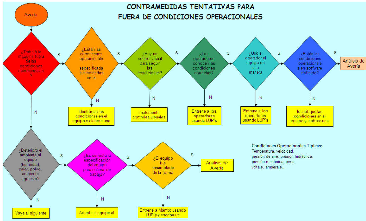
FIGURA 3.8: FLUJO PARA LA CONTRAMEDIDA DETERIORO NATURAL
