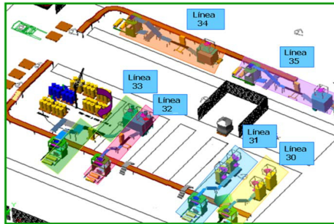
FIGURA 2.1: LAYOUT DEL ÁREA DE ENVASADO
