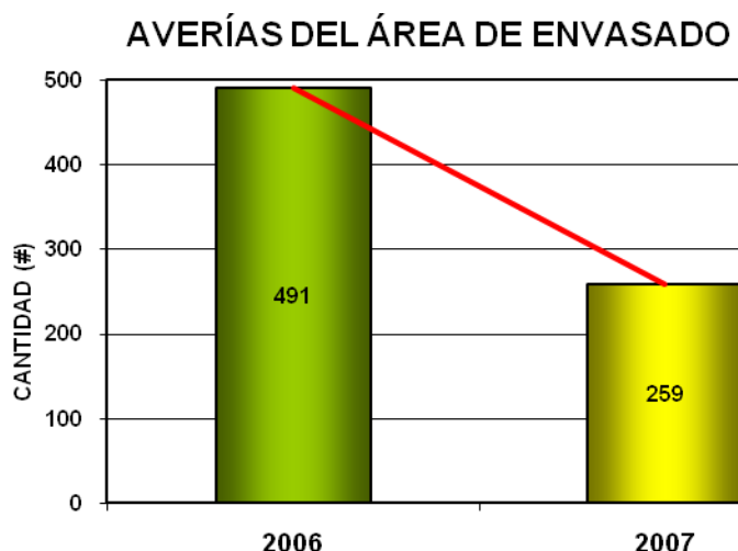
FIGURA 2.3: NÚMERO DE AVERÍAS DE ENVASADO DEL 2006 Y 2007
