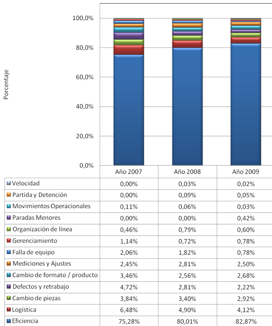
FIGURA 3.32: EFICIENCIA OPERACIONAL
