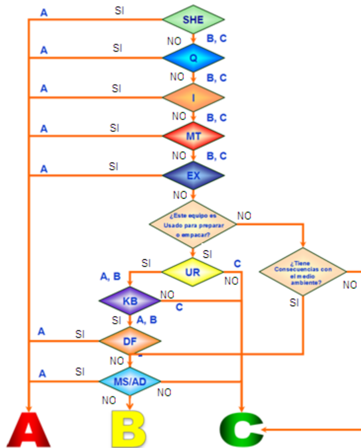
FIGURA 3.1: FLUJO PARA DETERMINAR CRITICIDAD DE LOS EQUIPOS
