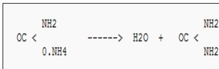
Figura 1.1 Fórmula carbamato amónico.
