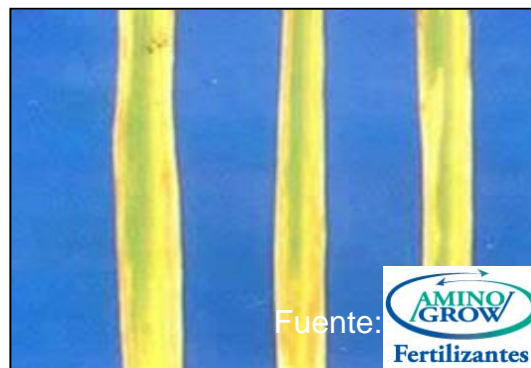
Figura 1.5 Planta con deficiencia de magnesio
