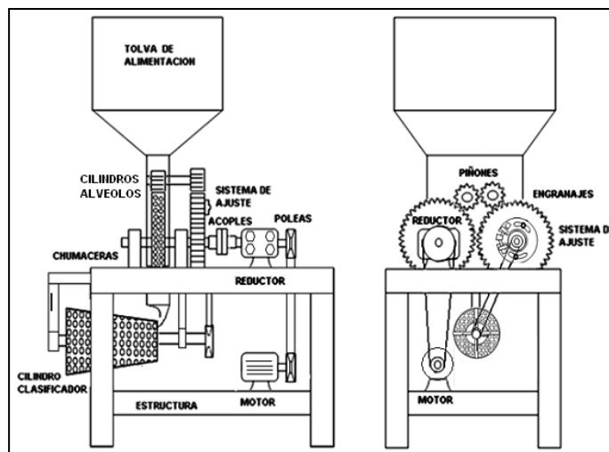
Figura 2.1 Máquina de hacer briquetas.
