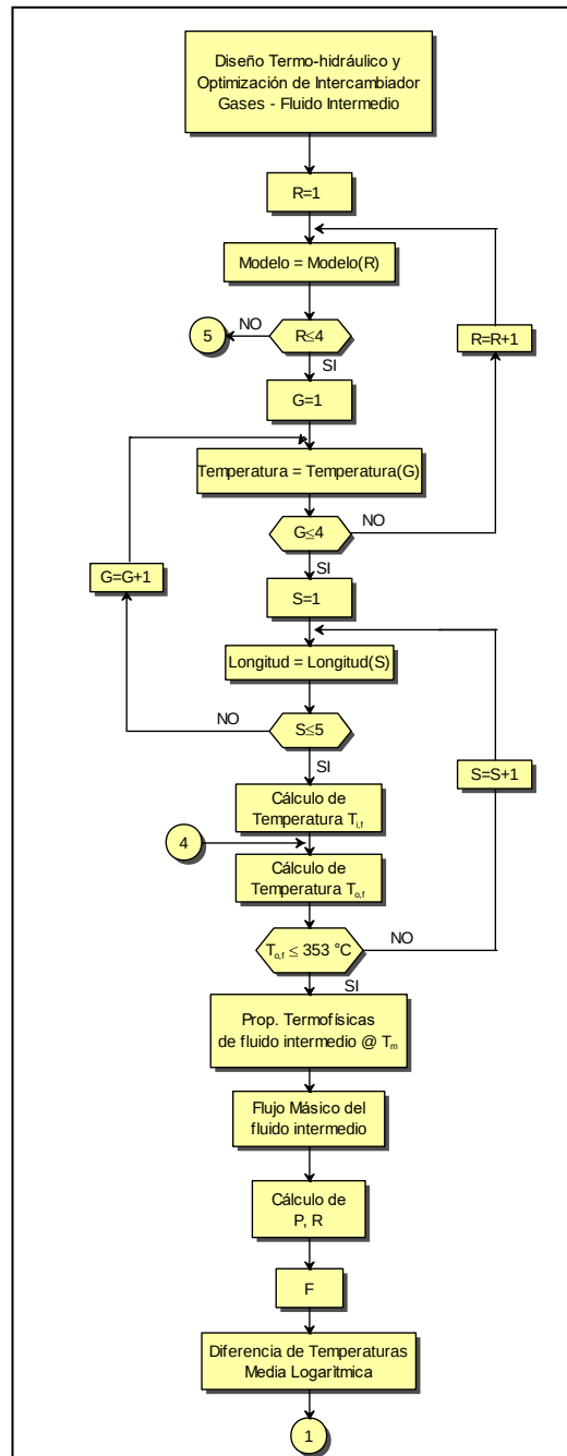
FIGURA 5.2 FLUJOGRAMA DEL DISEÑO INTERCAMBIADOR GASES – FLUIDO INTERMEDIO
