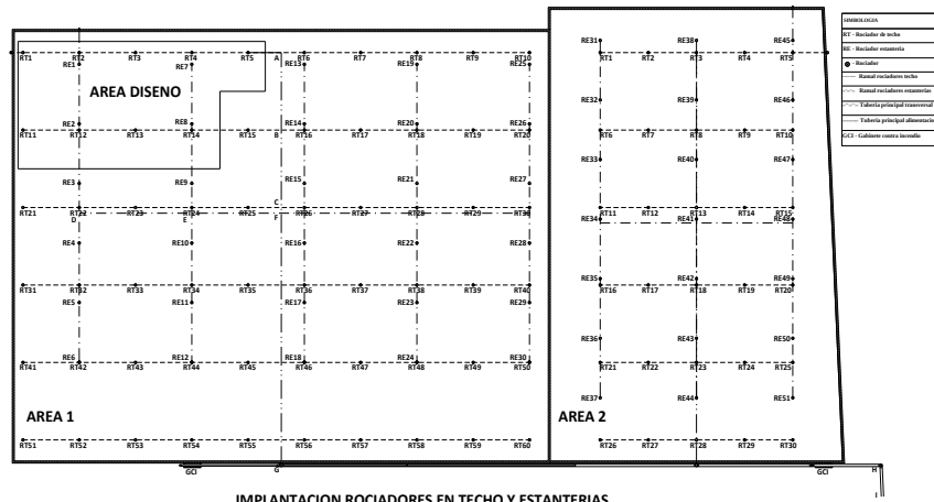
FIGURA 4.9.- UBICACIÓN DEL ÁREA DE DISEÑO.
