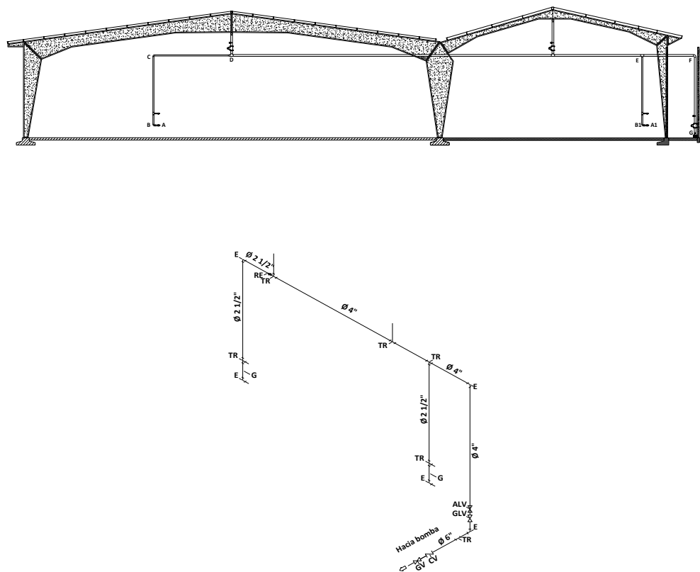
FIGURA 4.15.- ISOMÉTRICO TUBERÍAS DE GABINETES CONTRA INCENDIO.
