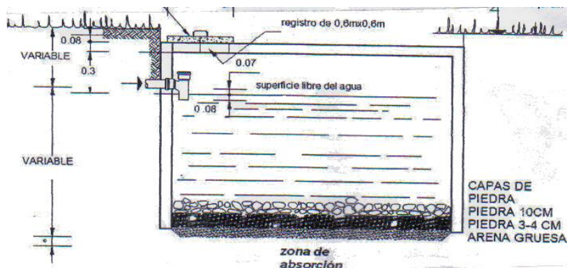
Modelo de propuesta de la fosa séptica Diseño: Ing. Víctor Orozco
